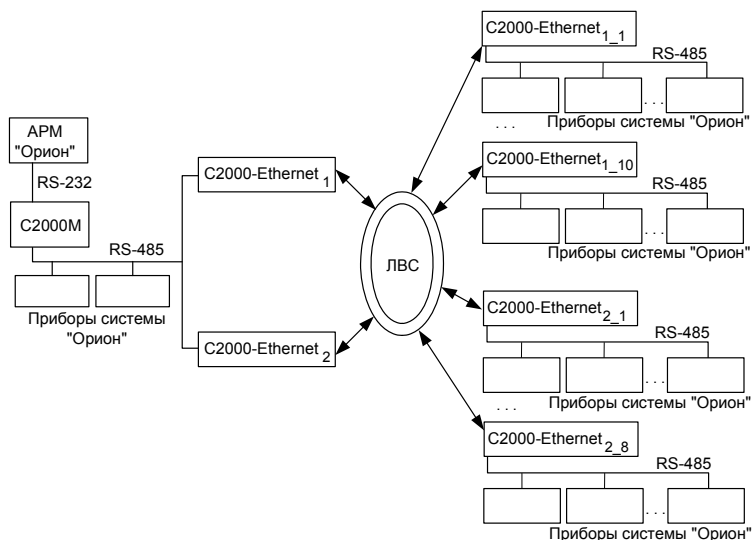
Рисунок 5 Пример схемы подключения «C2000-Ethernet»
