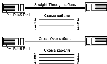
Рисунок 7 Типы Ethernet-кабелей
