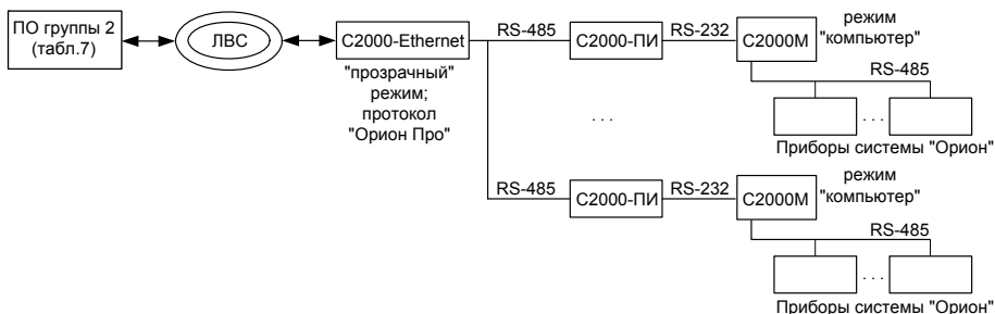
Рисунок 4 Схема подключения нескольких пультов «C2000»/«C2000M» к одному виртуальному COM-порту
