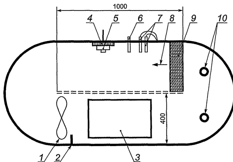
1 — вентилятор с двигателем; 2 — вводной патрубок газа; 3 — техническое окно; 4 — площадка с поворотным устройством для установки испытываемого ИПГ; 5 — испытываемый ИПГ; 6 — газоанализатор; 7 — измерители температуры и скорости потока воздуха; 8 — направление потока воздуха; 9 — линейаризатор; 10 — приточно-вытяжная вентиляция
