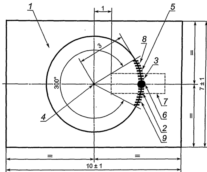
1 — помещение для проведения огневых испытаний; 2 — измеритель оптической плотности дыма (приемник/передатчик); 3 — устройство контроля температуры; 4 — место расположения тестового очага; 5 — измерительная зона точечных ИП (см. рис А.2); 6 — воздухозаборное отверстие ИПДА; 7 — устройство циркуляции воздуха (см. рис. А.5); 8 — контрольно-ионизационная камера ; 9-газоанализатор
