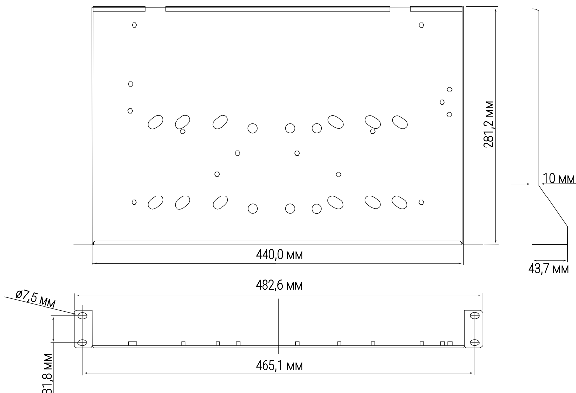
Рисунок 5.1 – Габаритные размеры
