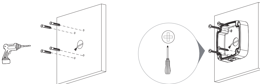
Рисунок 4.3 – Монтаж
