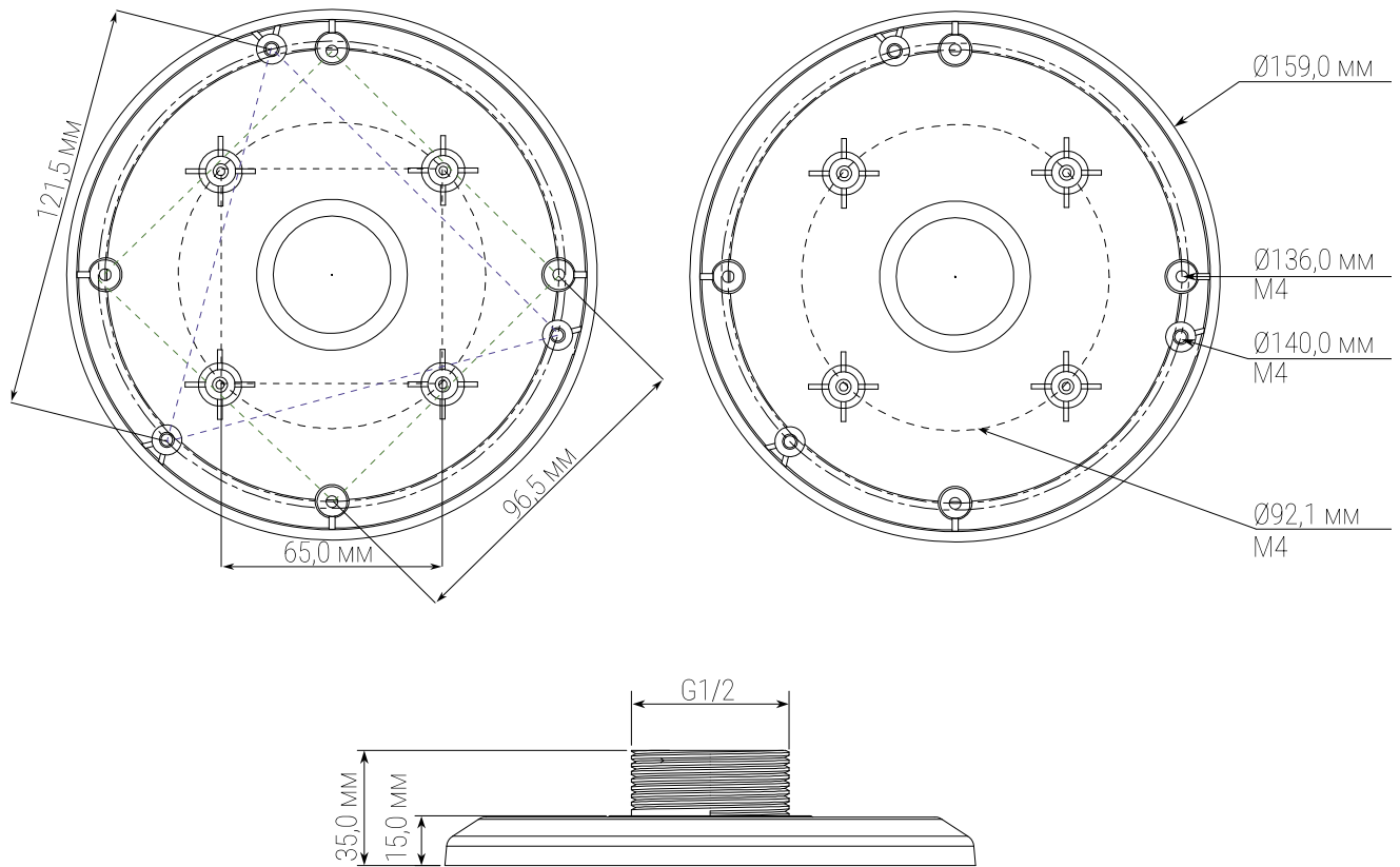
Рисунок 4.1 – Габаритные размеры
