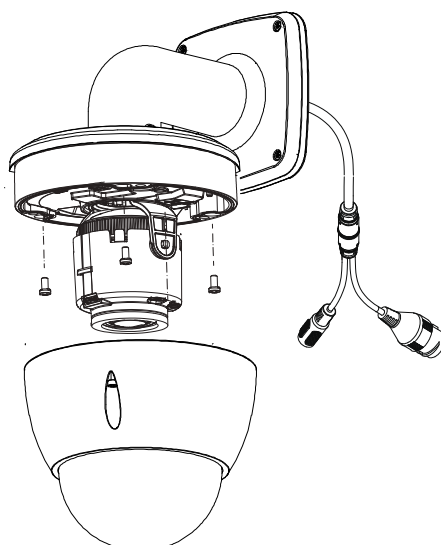
Рисунок 4.5 – Монтаж
