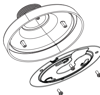
Рисунок 4.5 – Монтаж
