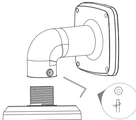
Рисунок 4.4 – Монтаж
