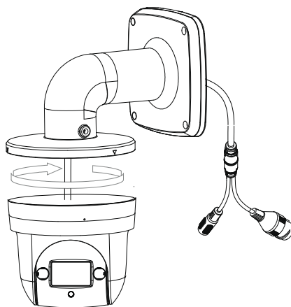
Рисунок 4.6 – Монтаж
