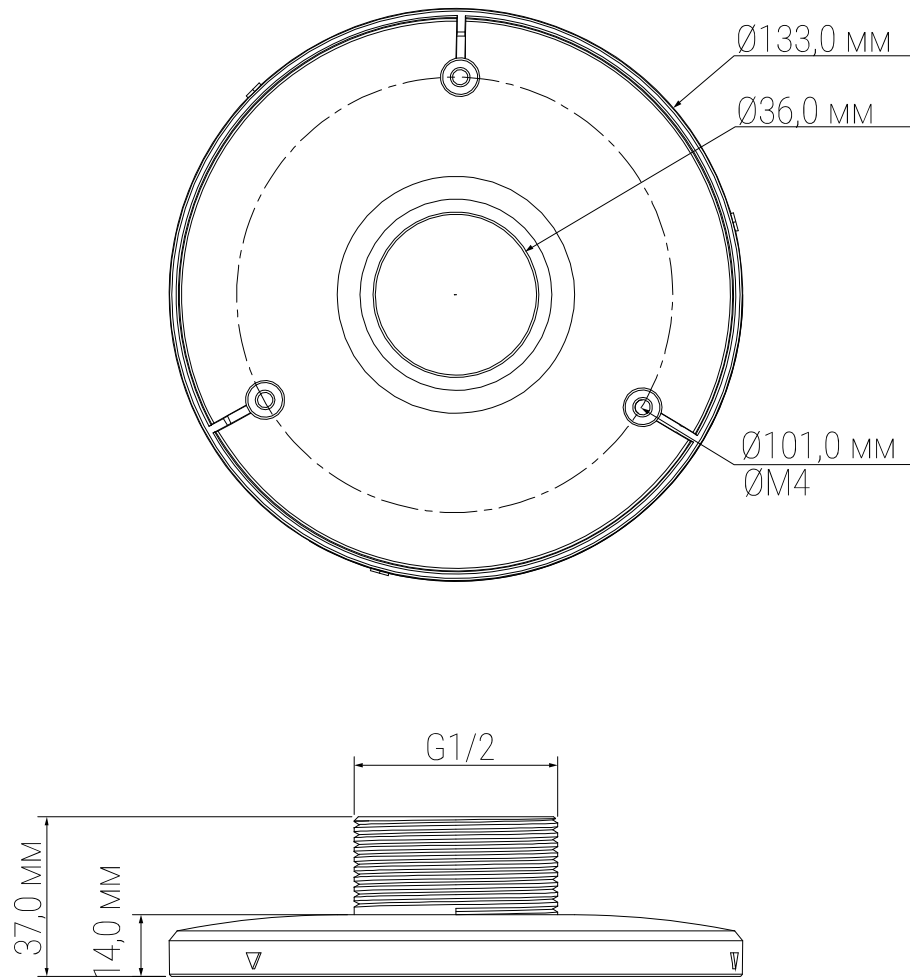
Рисунок 4.1 – Габаритные размеры
