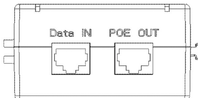
Рисунок 3.1 – Передняя панель
