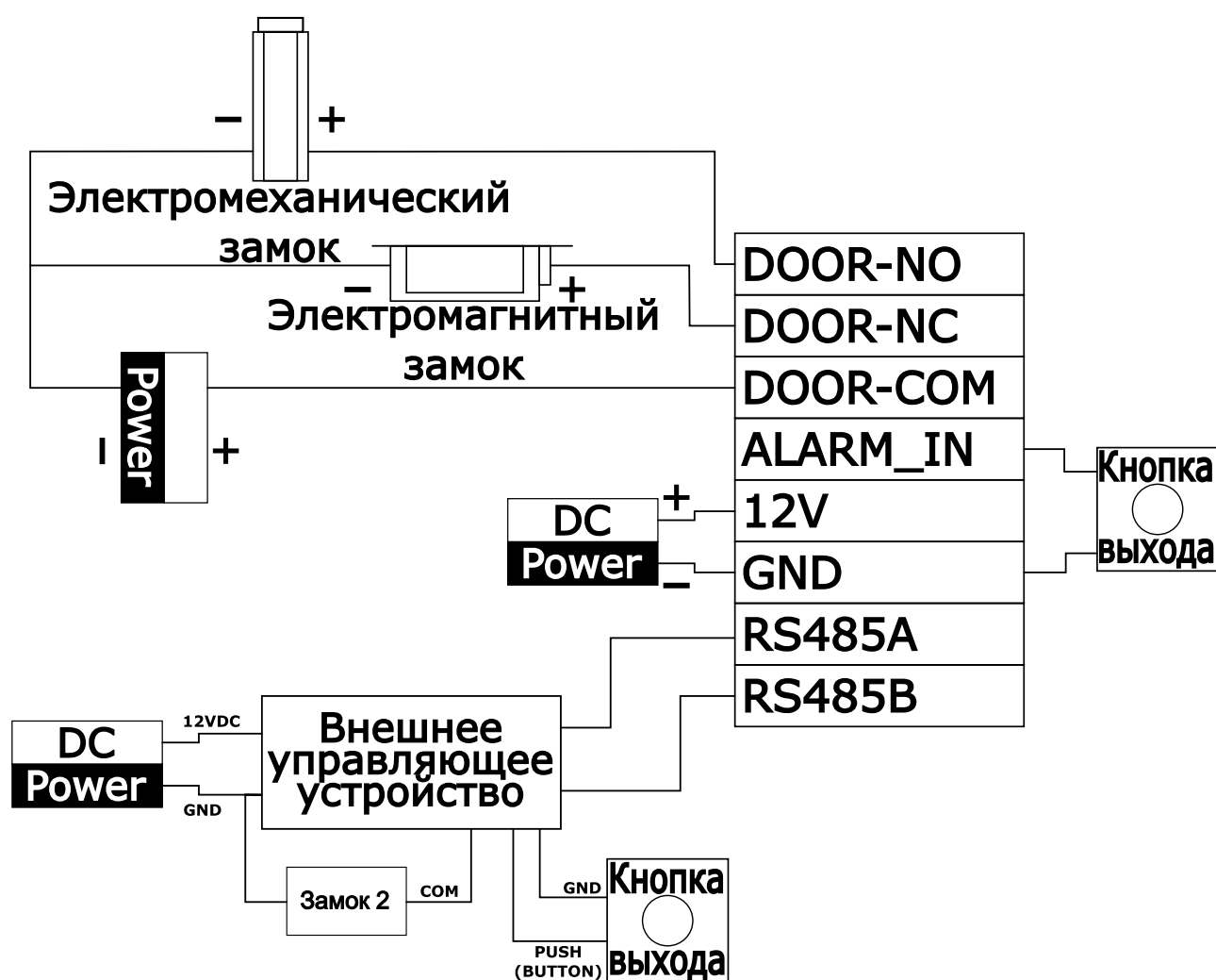
Рисунок 3.5 – Схема подключения. Замок 2
