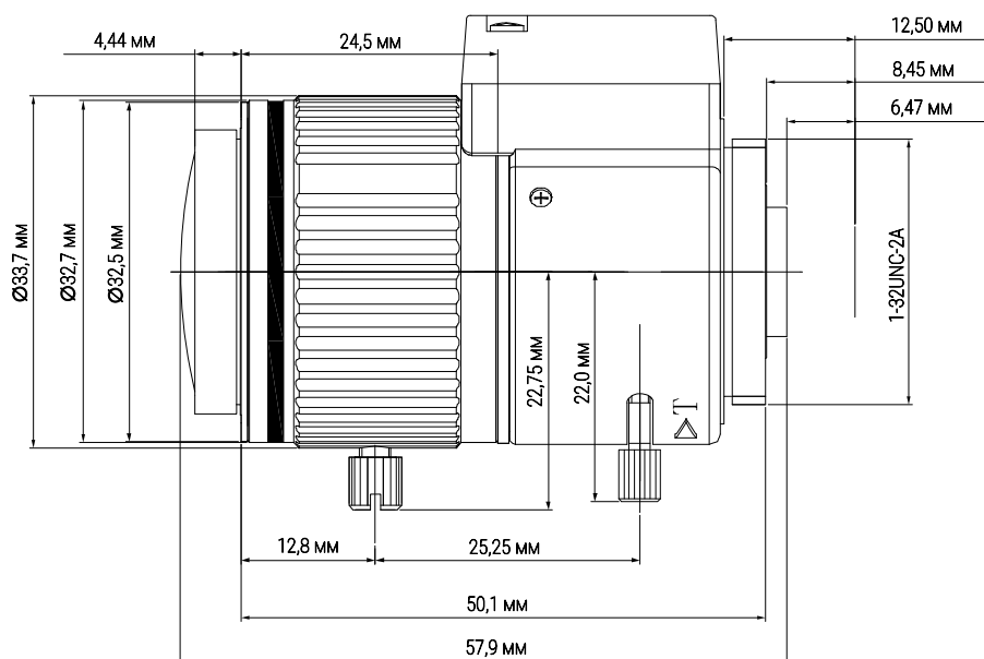
Рисунок 5.1 – Габаритные размеры
