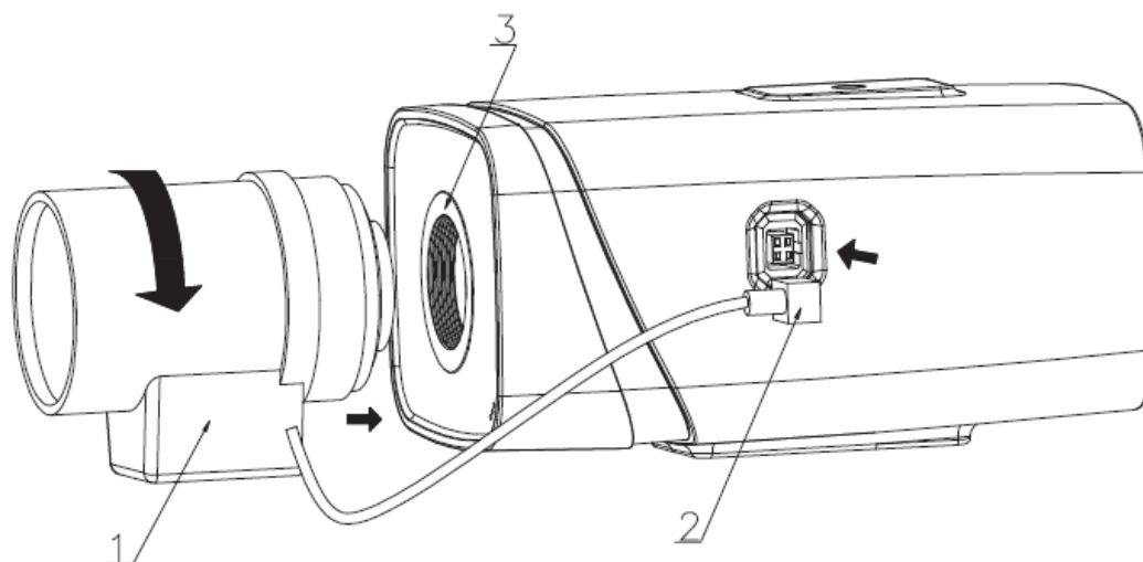
Рисунок 5.2 – Присоединение объектива
