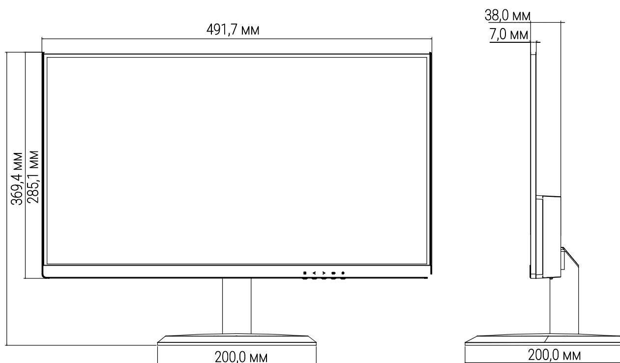
Рисунок 4.1 – Габаритные размеры
