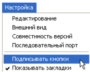
Рисунок 20 – Меню «Настройка»
