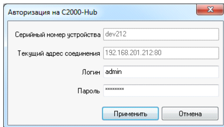
Рисунок 13 – Окно авторизации
