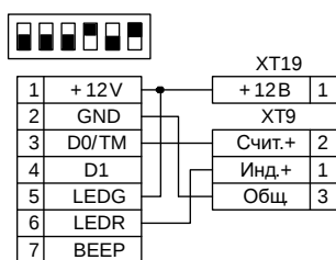
«Сигнал ВК-6»
