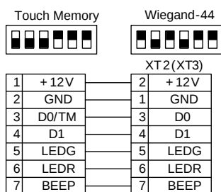
«С2000-2»
