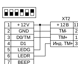
«Сигнал ВК-2»
