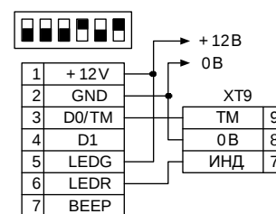
«УО-4С»
