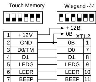
«Сигнал-ВК-4» исп. 05
