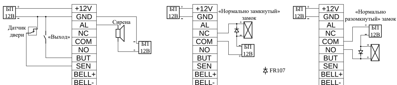
Рисунок 2. Схемы подключения в автономном режиме
