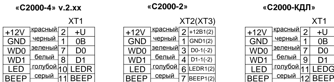
Рисунок 3. Схемы подключения к ПКП и контроллерам СКД (контроллер всегда слева)
