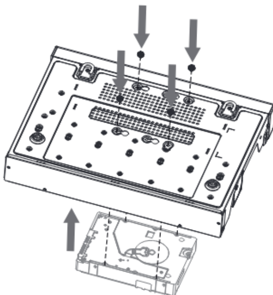
Рисунок 4.6 – Установка жесткого диска
