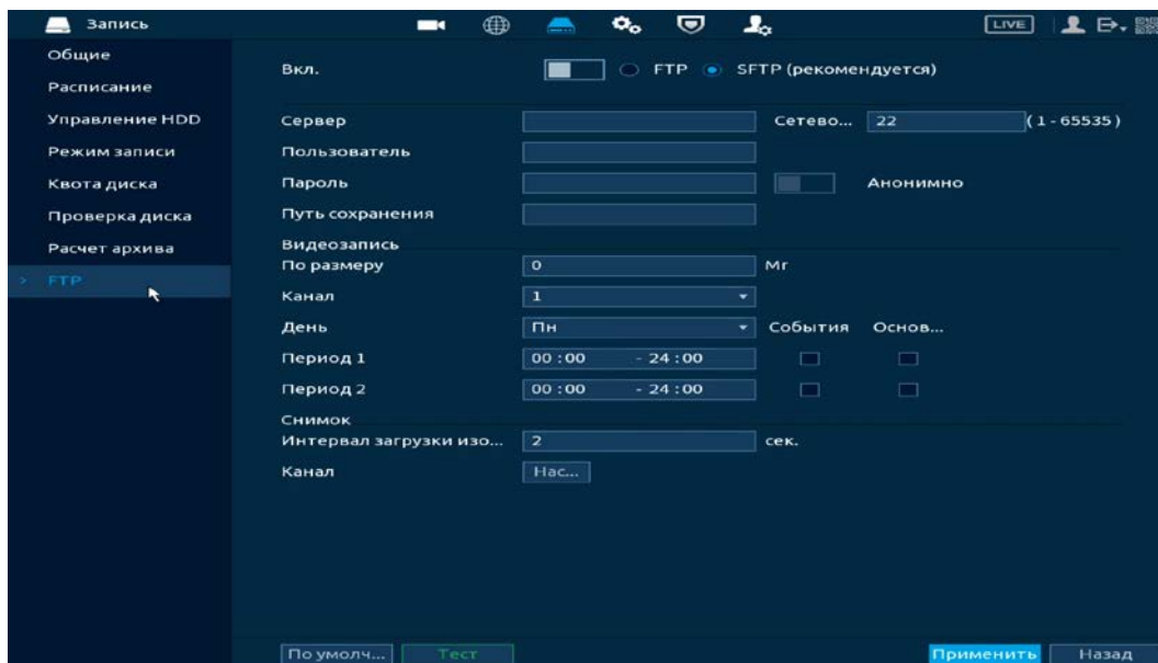
Рисунок 14.23 – Настройка FTP
