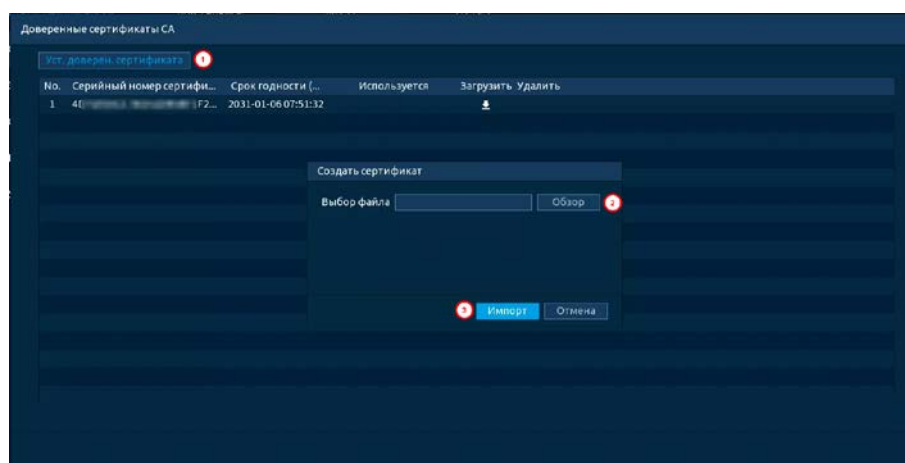
Рисунок 16.4 – Импорт
