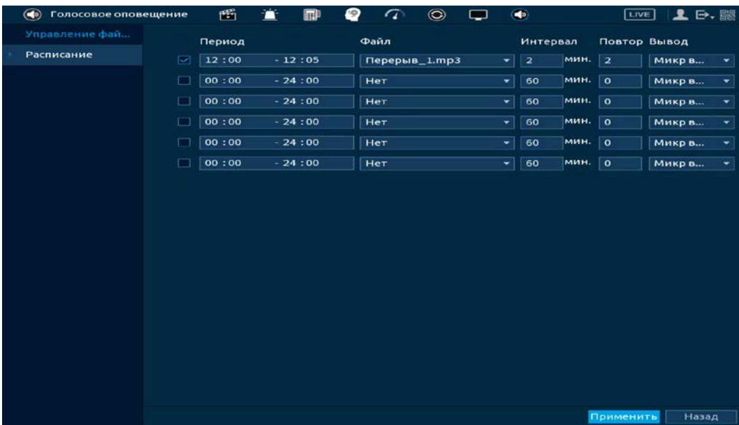
Рисунок 25.3 – Расписание
