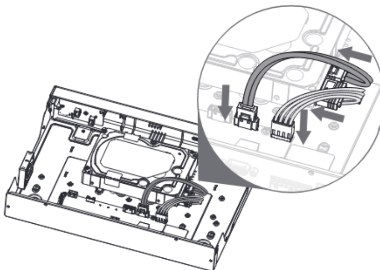
Рисунок 4.7 – Установка жесткого диска
