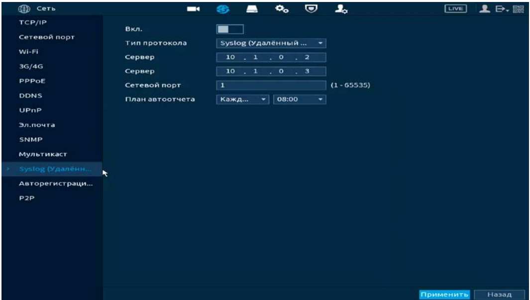
Рисунок 13.13 – Интерфейс настройки «Syslog (Удаленный журнал)»
