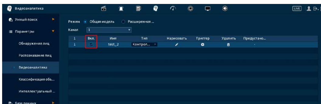
Рисунок 21.29 – Настройка
