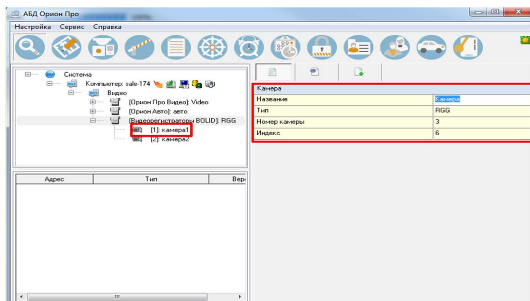
Рисунок 29.3 – Добавление камер
