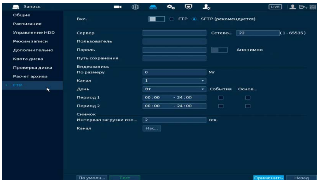
Рисунок 14.28 – Настройка FTP
