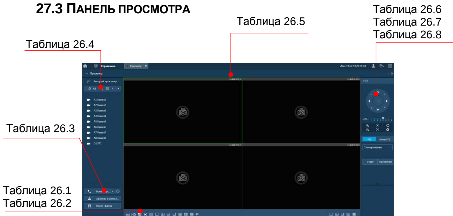
Рисунок 27.1 – Режим просмотра
