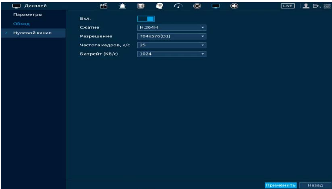
Рисунок 24.15 – Интерфейс настройки
