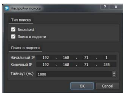
Рисунок 28.3 – Настройка поиска
