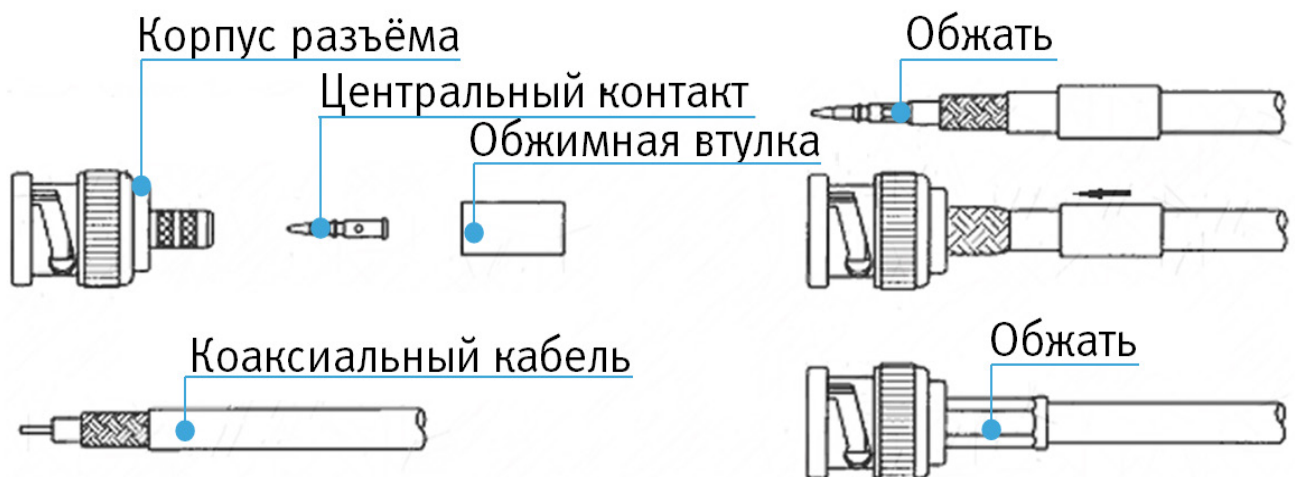
Рисунок 4.1 – Схема обжима BNC
