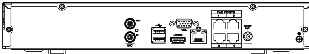
Рисунок 2 Задняя панель.
