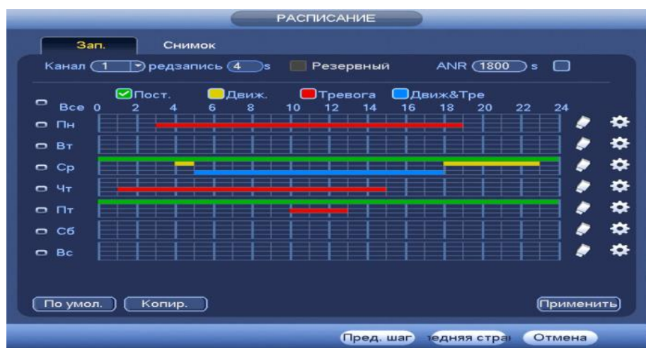
Рисунок 10 Настройка расписания.
