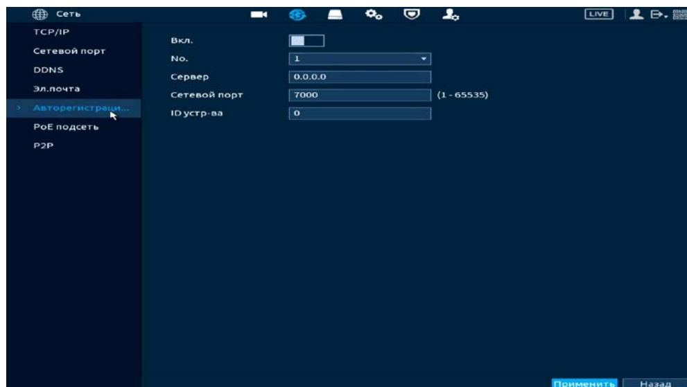
Рисунок 12.6 – Интерфейс настройки «Авторегистрация на прокси»
