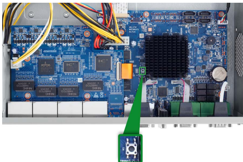
Рисунок 24.8 – Пример расположения кнопки сброса
