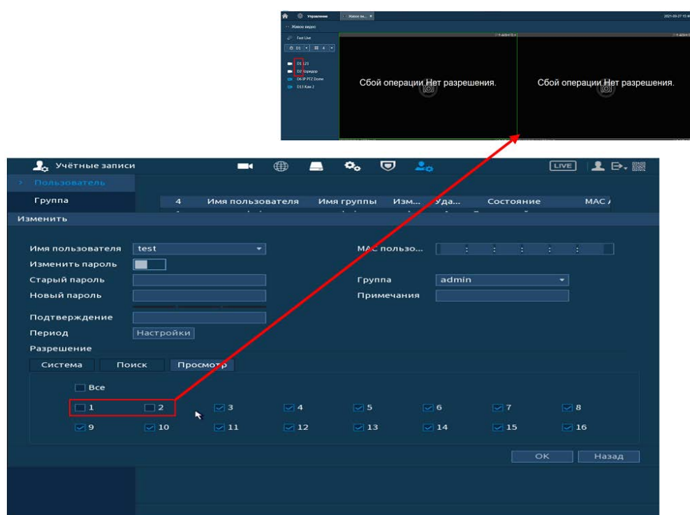
Рисунок 16.6 – Снят доступ для просмотра видеопотока пользователем (каналы D1 и D2)
