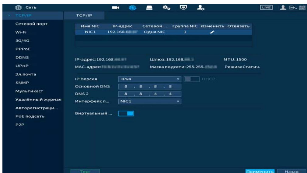
Рисунок 12.1 – Интерфейс настройки «Сеть»
