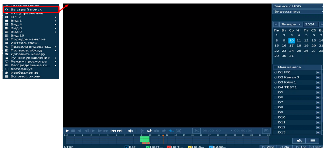
Рисунок 17.2 – Меню просмотра «Архив»
