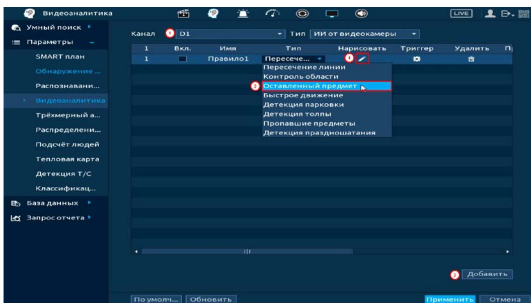
Рисунок 19.43 – Функция видеоаналитики «Оставленный предмет»
