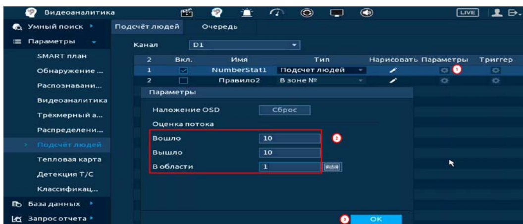
Рисунок 19.79 – Интерфейс настройки подсчета посетителей
