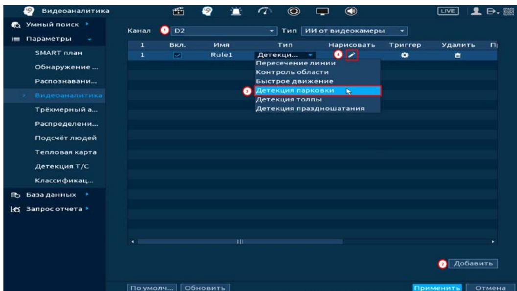
Рисунок 19.58 – Функция видеоаналитики «Детекция парковки»
