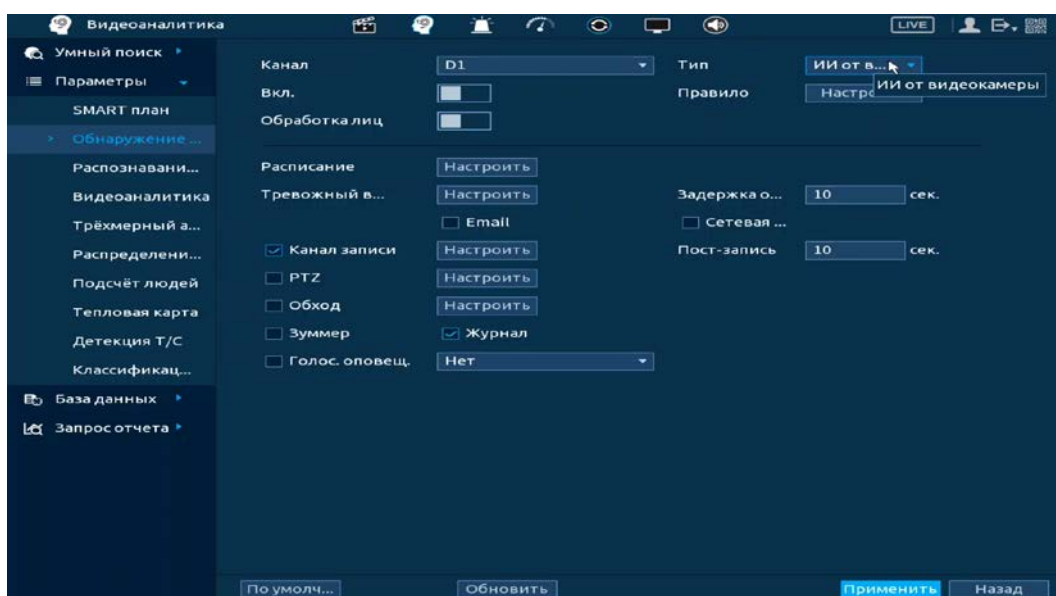
Рисунок 19.10 – Интерфейс настройки обнаружения лиц. ИИ от видеокамеры
