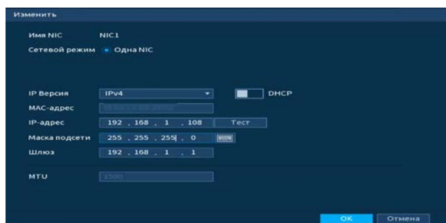
Рисунок 12.2 – Интерфейс настройки «Сеть»
