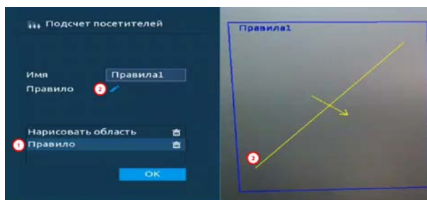
Рисунок 19.78 – Интерфейс настройки подсчета посетителей
