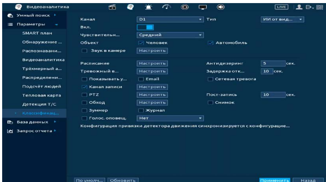
Рисунок 19.100 – Классификация объектов
