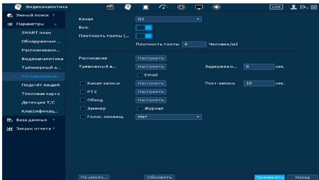
Рисунок 19.72 – Распределение толпы
