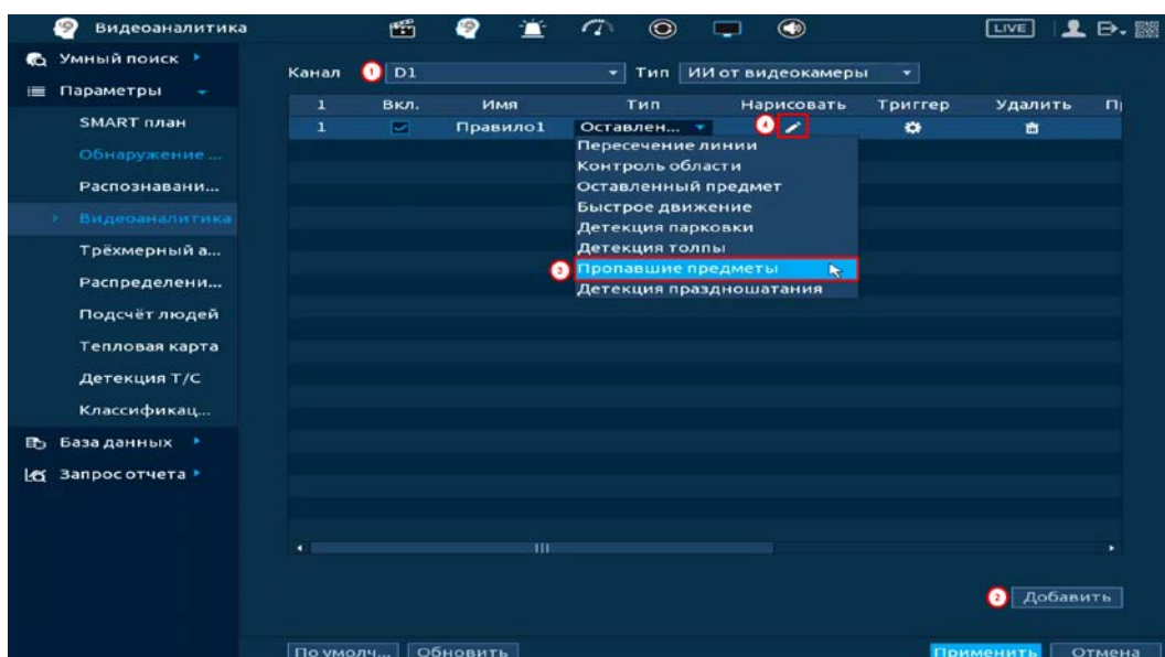
Рисунок 19.48 – Функция видеоаналитики «Пропавший предмет»
