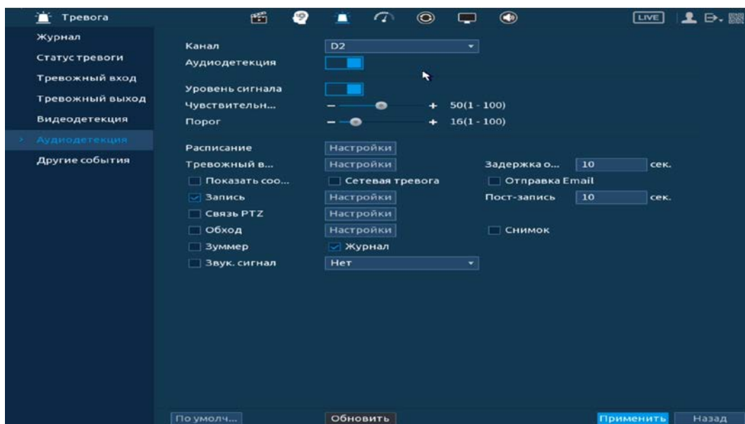
Рисунок 17.33 – Настройка аудиодетекции
