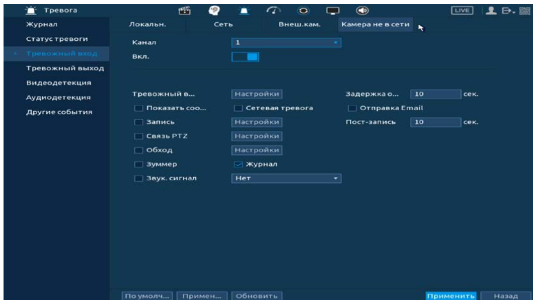
Рисунок 19.4 – Интерфейс настройки
