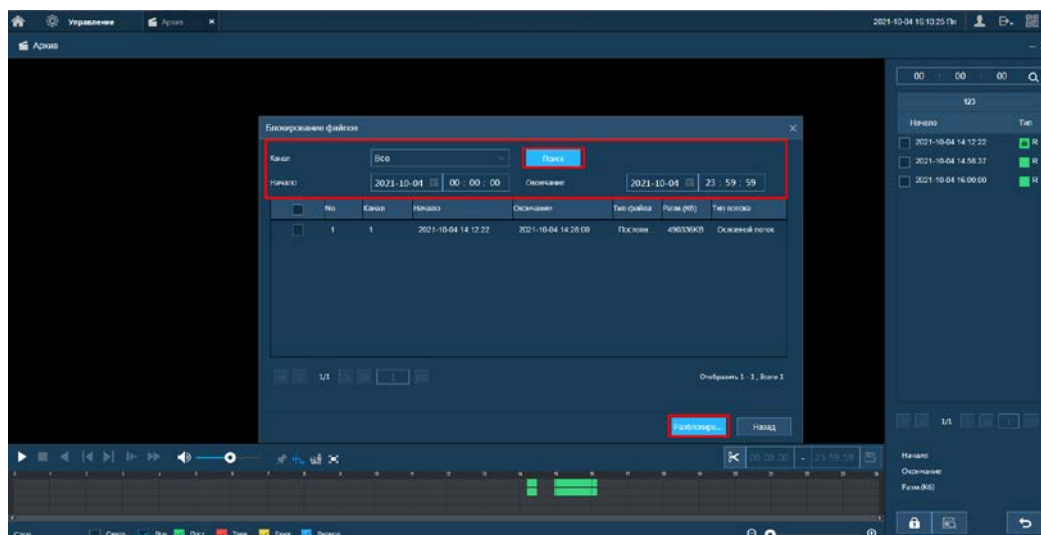
Рисунок 23.11 – Блокировка/Разблокировка файлов
