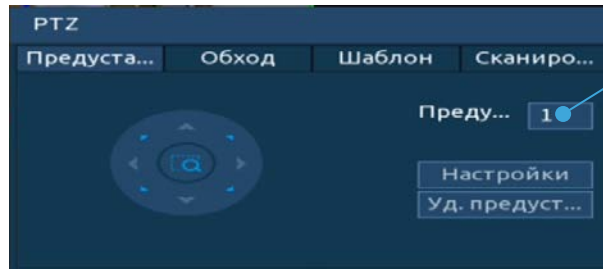
Рисунок 6.11 – Интерфейс «Предустановки»
