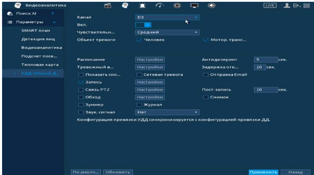
Рисунок 17.32 – Настройка УДД
