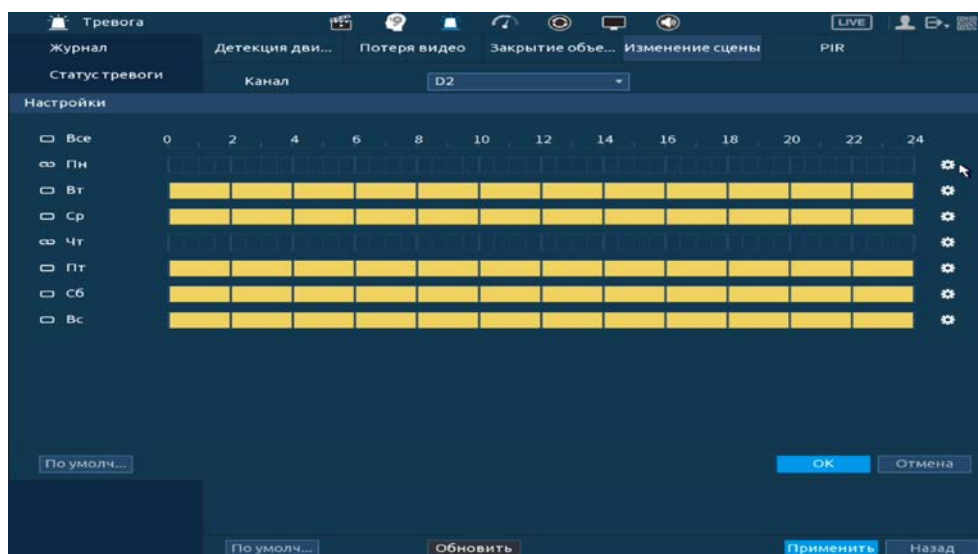
Рисунок 13.12 – Панель расписания
