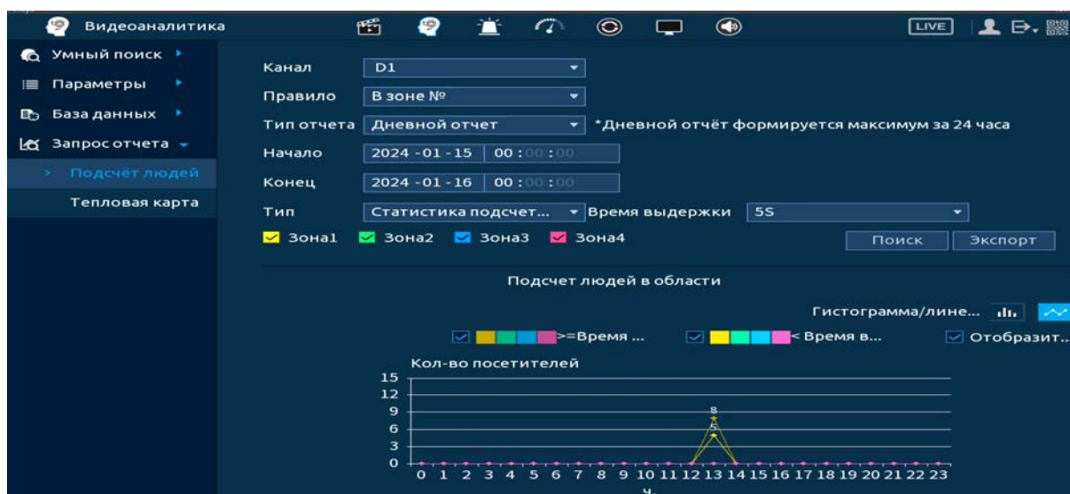
Рисунок 20.109 – Статистика по количеству человек
