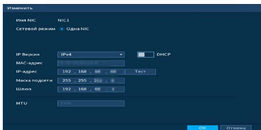
Рисунок 13.2 – Интерфейс настройки «Сеть»
