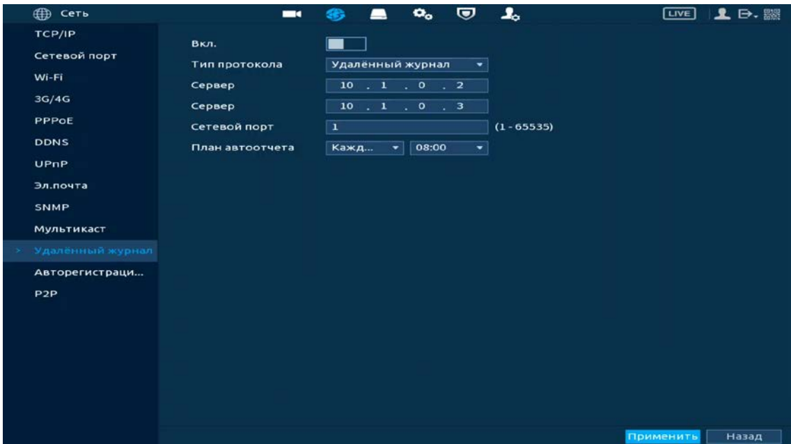
Рисунок 13.14 – Интерфейс настройки «Удаленный журнал»
