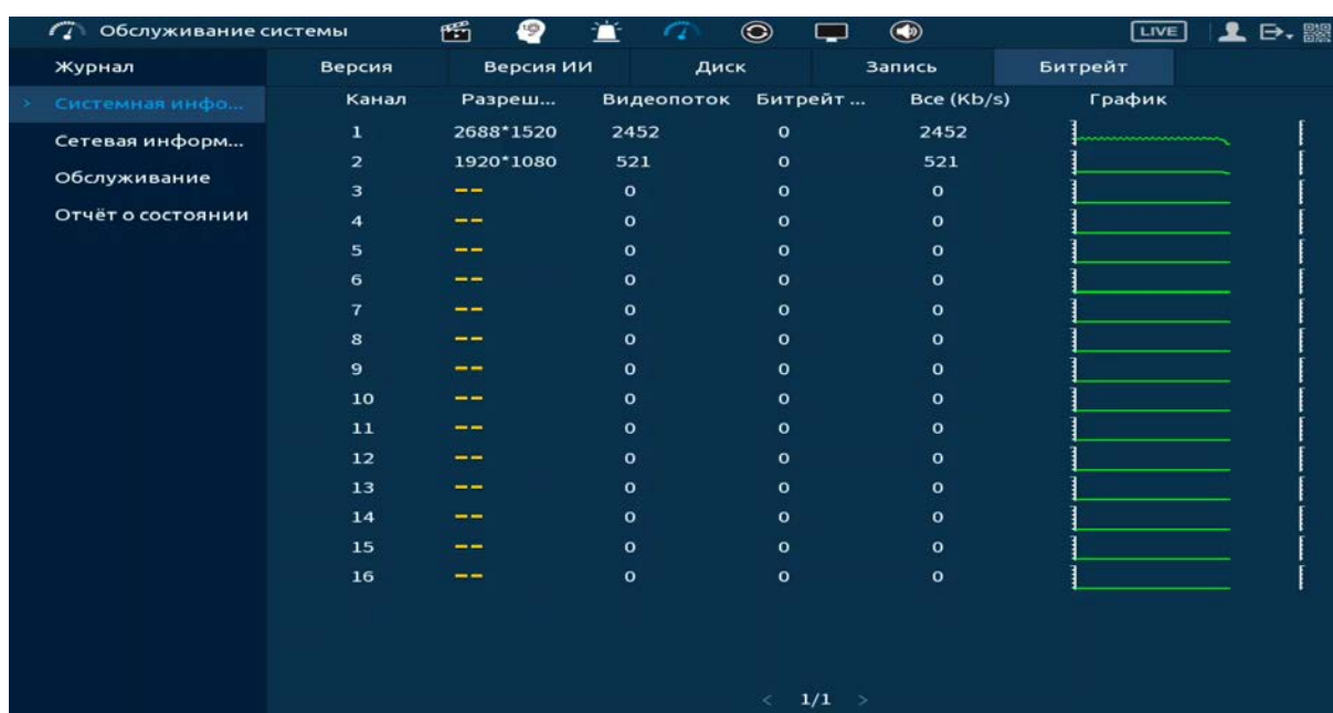
Рисунок 21.6 – Интерфейс просмотра битрейта
