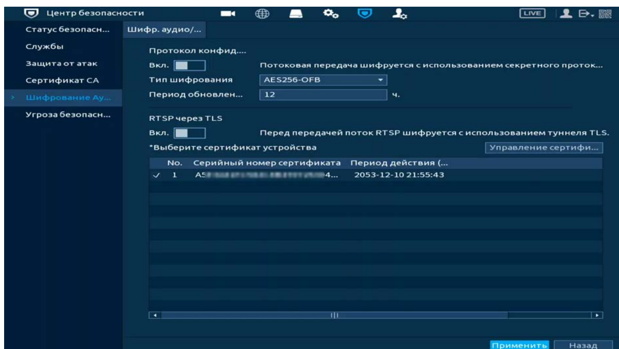
Рисунок 16.21 – Интерфейс шифрования аудио/видео
