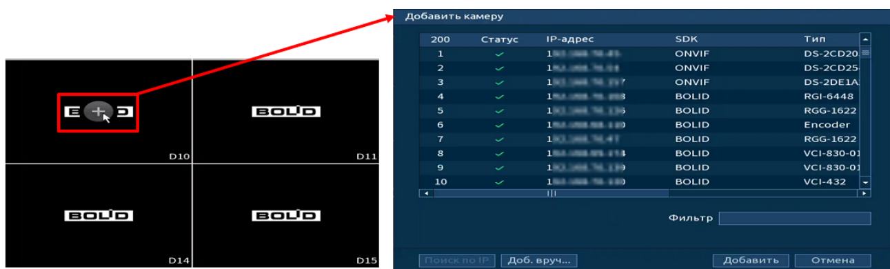
Рисунок 12.2 – Добавление в режиме просмотра
