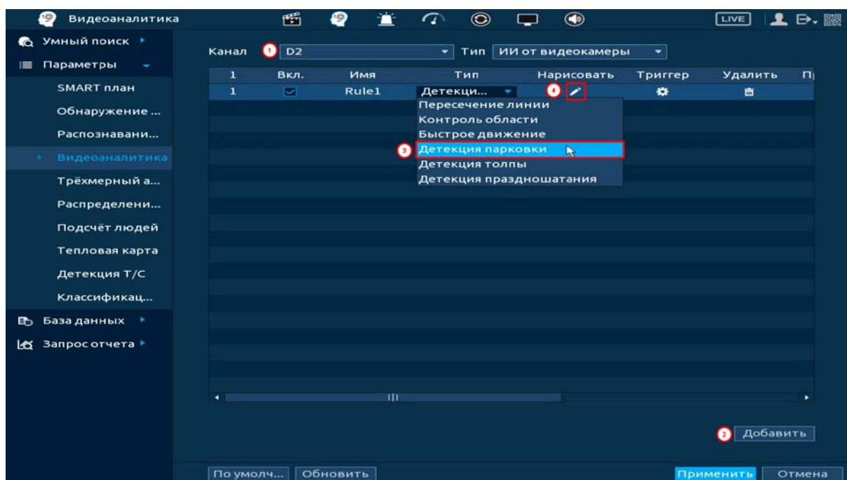
Рисунок 20.55 – Функция видеоаналитики «Детекция парковки»
