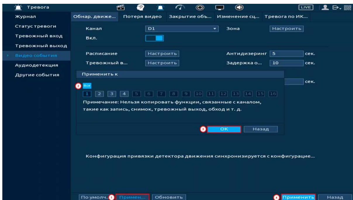
Рисунок 19.23 – Копирование настроек на другие каналы
