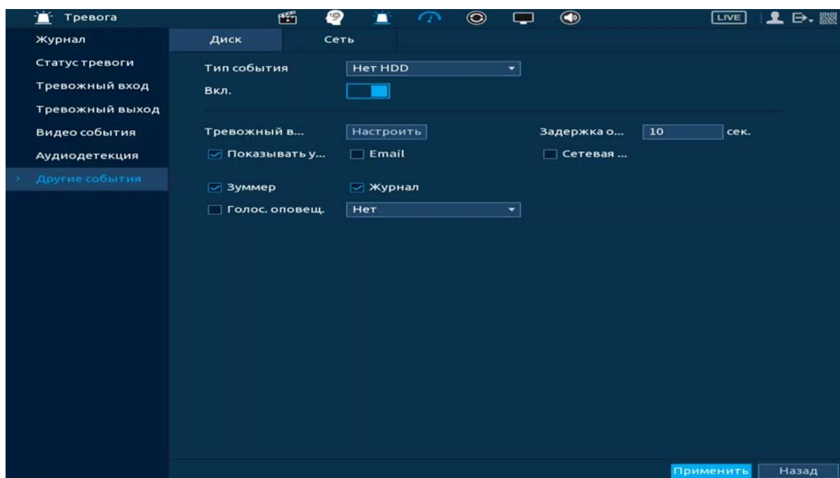
Рисунок 19.41 – Интерфейс настройки оповещения об ошибках HDD
