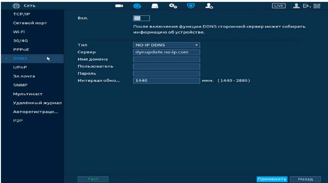
Рисунок 13.7 – Интерфейс настройки «DDNS»
