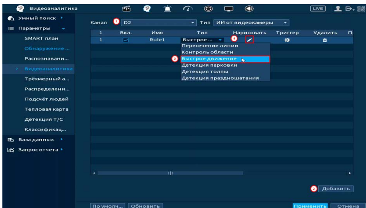
Рисунок 20.50 – Функция видеоаналитики «Быстрое движение»
