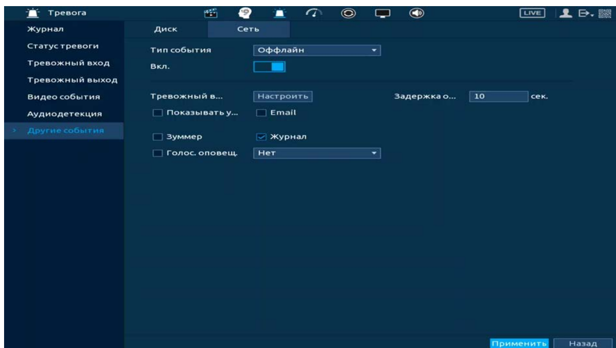
Рисунок 19.42 – Интерфейс настройки оповещения
