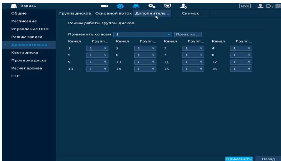
Рисунок 14.20 – Интерфейс настройки доп.потока
