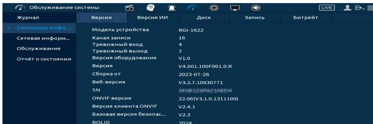
Рисунок 21.2 – Интерфейс просмотра информации о версии
