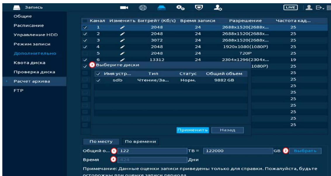
Рисунок 14.27 – Выбор диска для расчёта и результат
