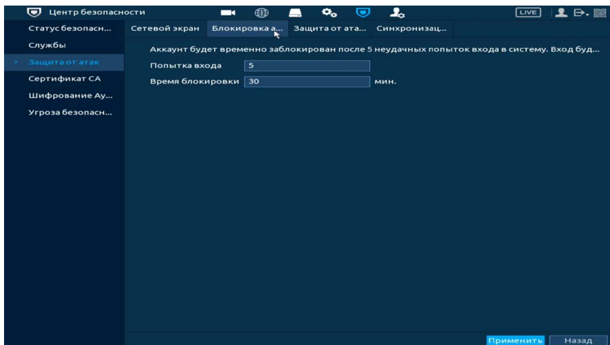
Рисунок 16.13 – Блокировка учетной записи
