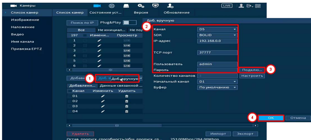
Рисунок 12.16 – Интерфейс ручного добавления удаленного устройства
