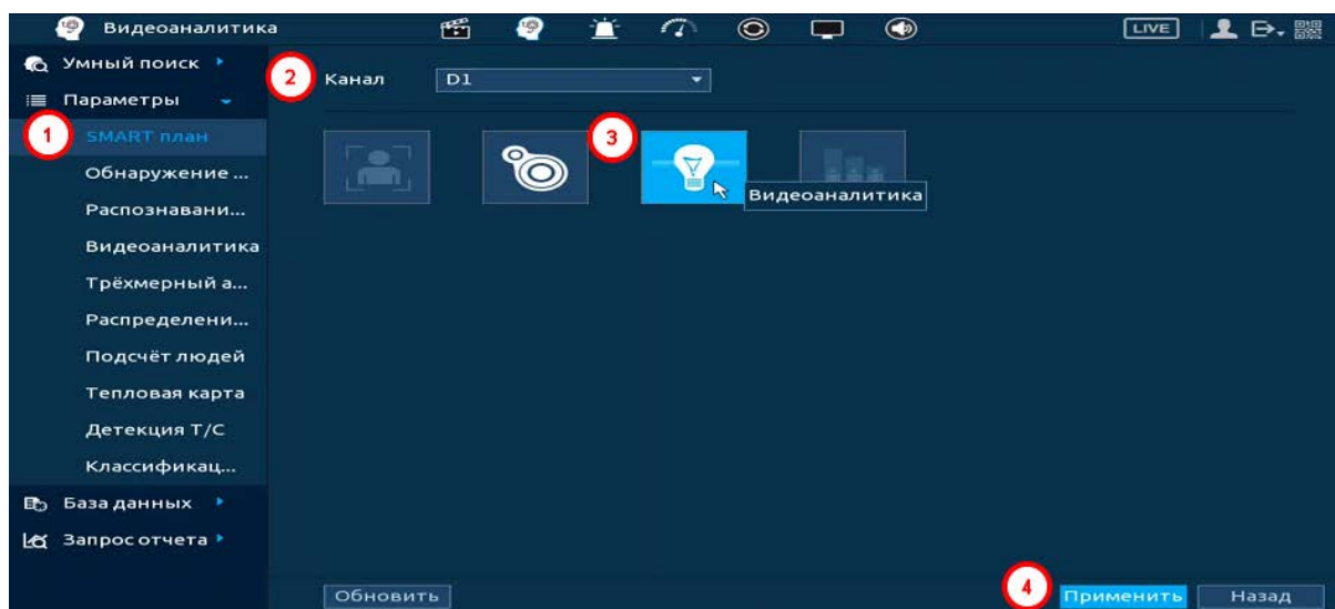
Рисунок 20.54 – Настройка
