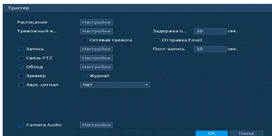
Рисунок 20.52 – Настройка параметров
