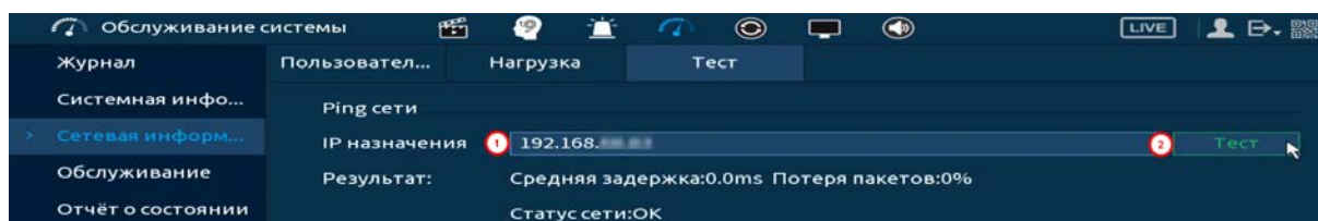
Рисунок 21.9 – Проверка IP-адреса
