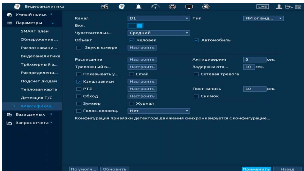
Рисунок 20.97 – Классификация объектов
