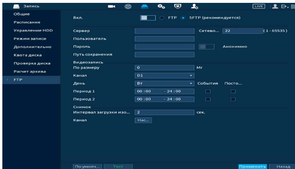
Рисунок 14.30 – Настройка FTP
