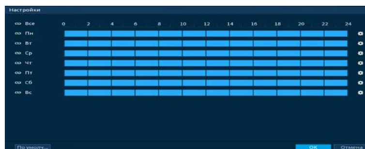
Рисунок 20.98 – Расписание
