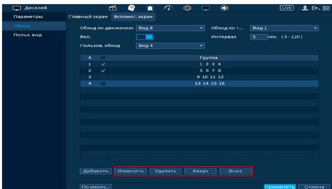
Рисунок 10.12 – Расположение групп
