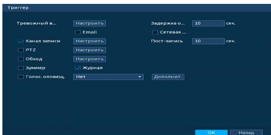
Рисунок 20.19 – Настройка
