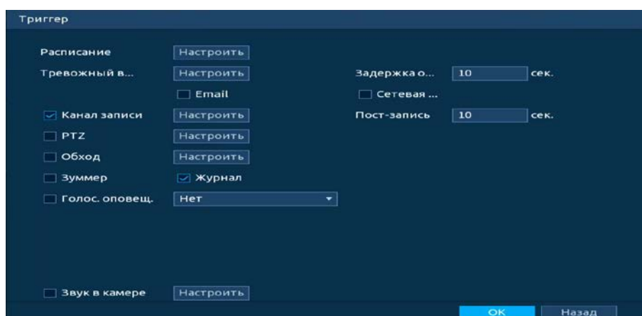
Рисунок 20.47 – Настройка параметров
