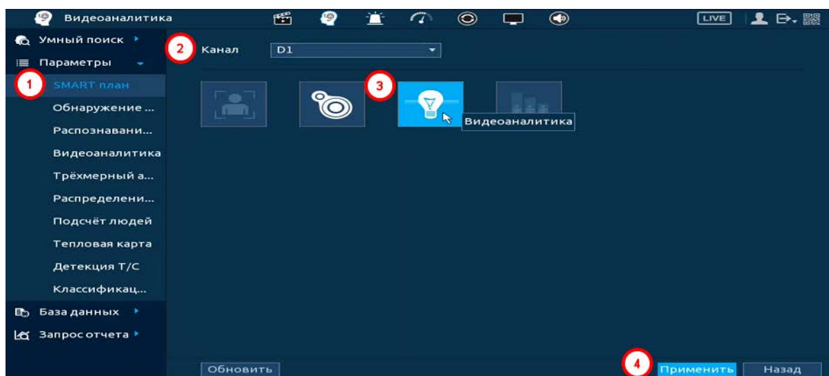
Рисунок 20.31 – Настройка
