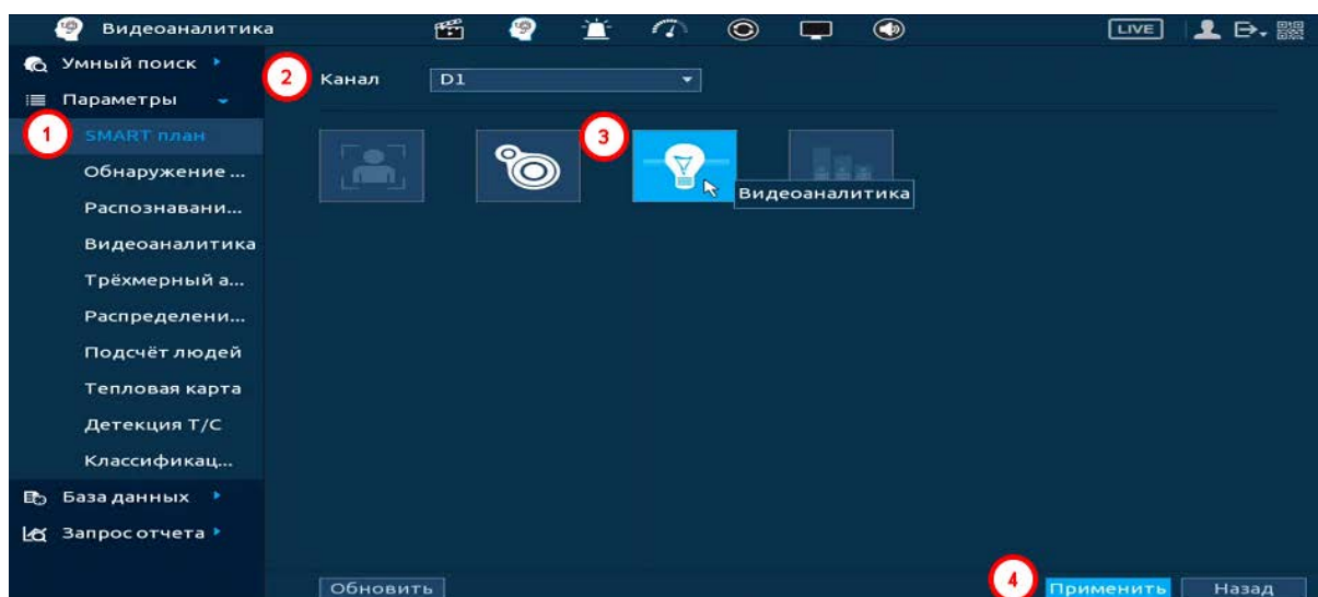
Рисунок 20.24 – Настройка
