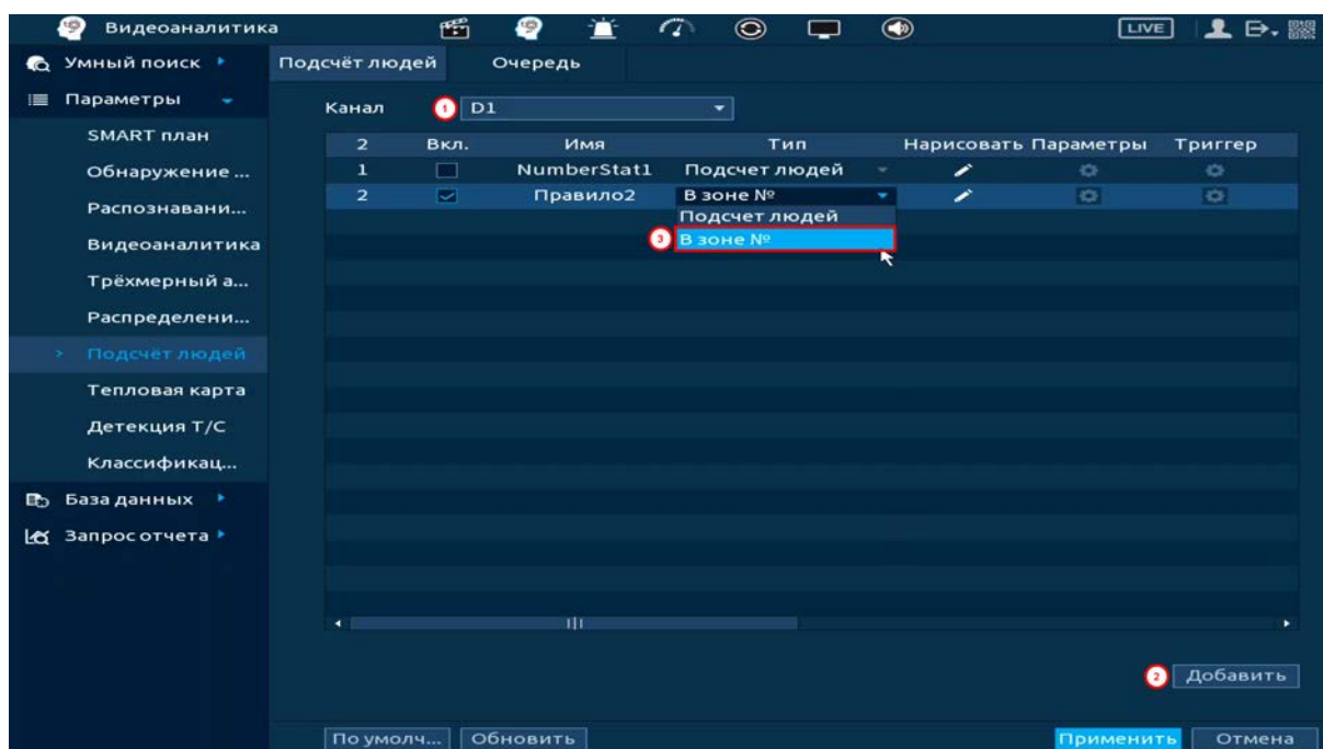
Рисунок 20.81 – Настройка
