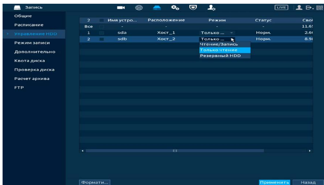
Рисунок 14.16 – Интерфейс настройки
