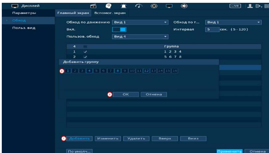
Рисунок 23.10 – Добавление группы
