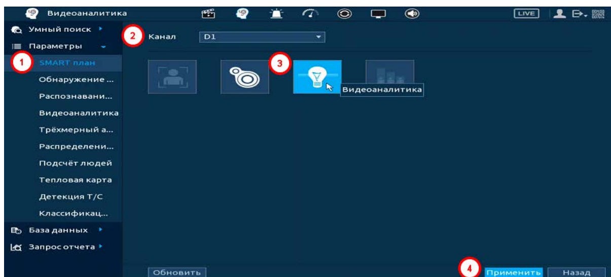
Рисунок 20.49 – Настройка
