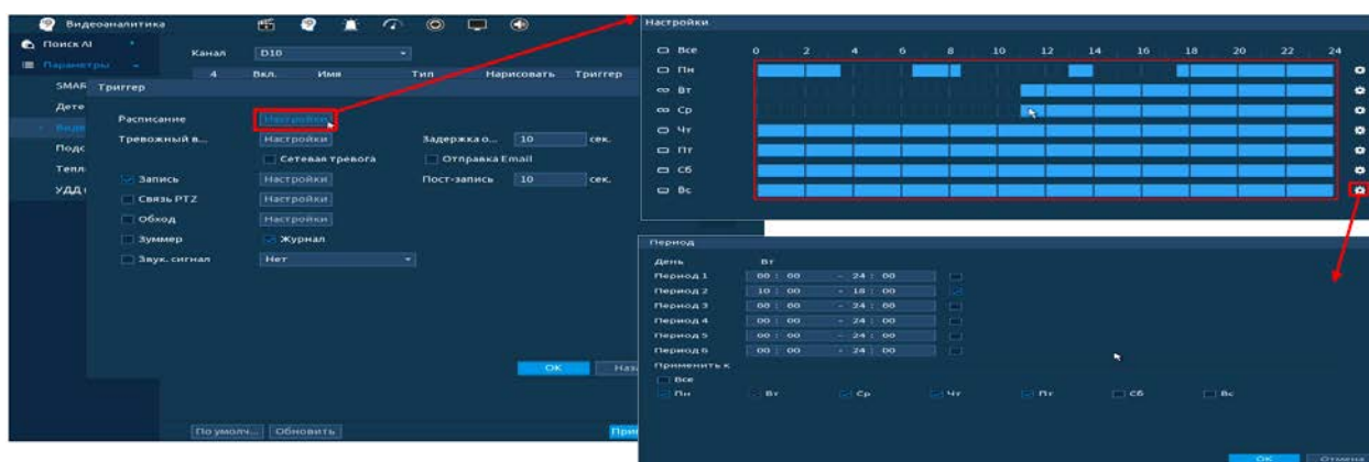
Рисунок 20.43 – Расписание
