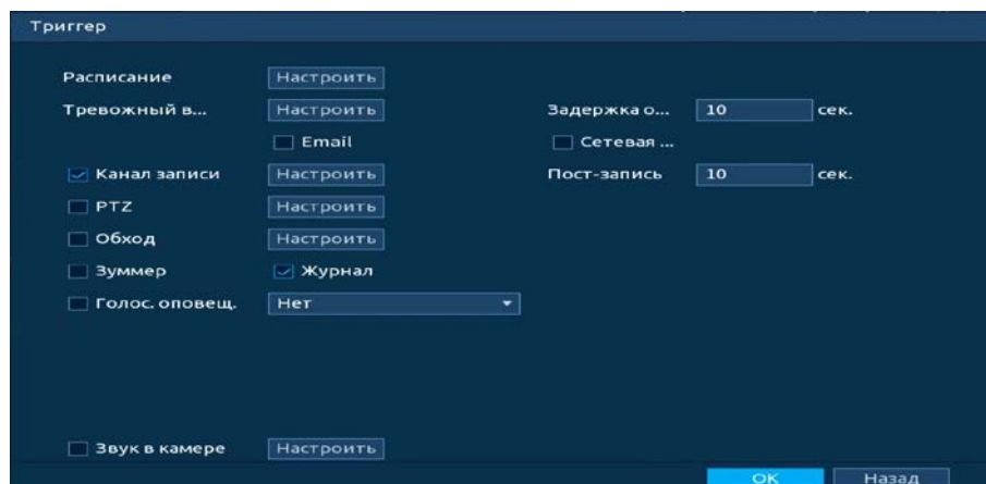
Рисунок 20.62 – Настройка параметров
