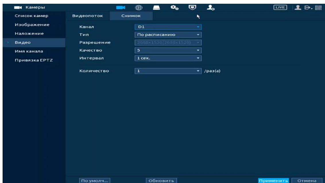
Рисунок 12.32 – Настройка снимка
