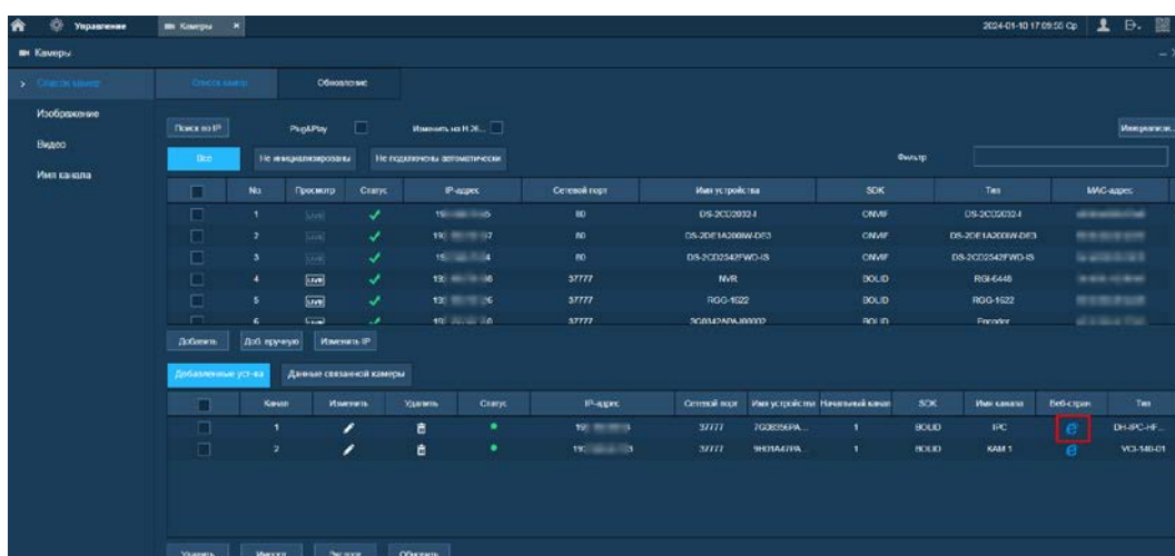
Рисунок 26.5 –Список камер
