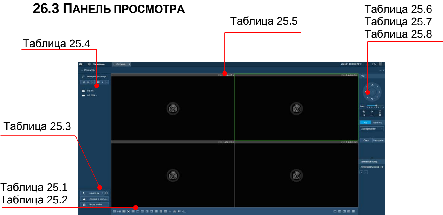
Рисунок 26.1 – Режим просмотра
