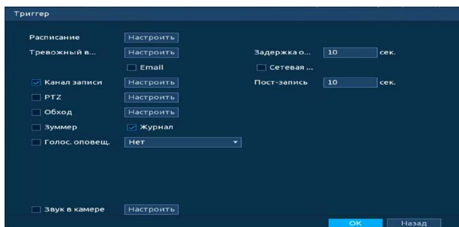
Рисунок 20.42 – Настройка параметров
