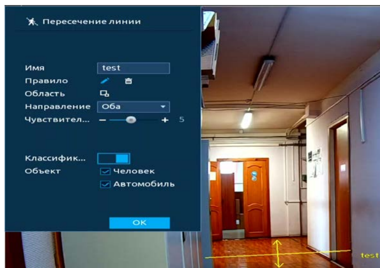
Рисунок 20.26 – Настройка правила
