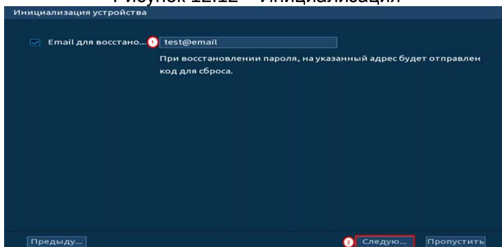
Рисунок 12.13 – Инициализация
