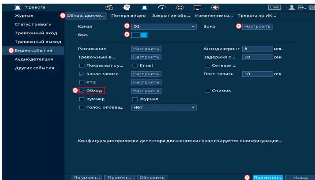
Рисунок 23.5 – Пример настройки
