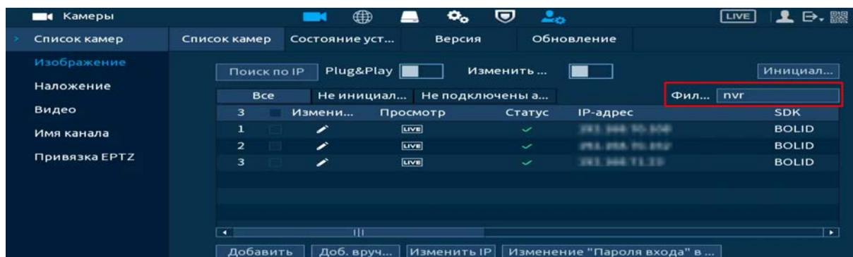
Рисунок 12.8 – Фильтр
