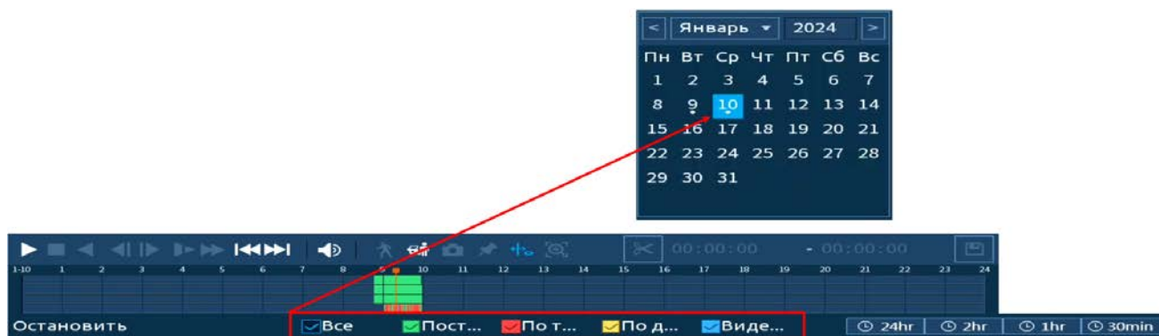
Рисунок 18.5 – Шкала времени
