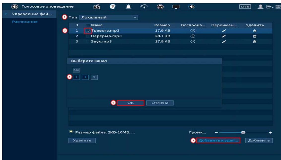
Рисунок 24.3 – Добавление
