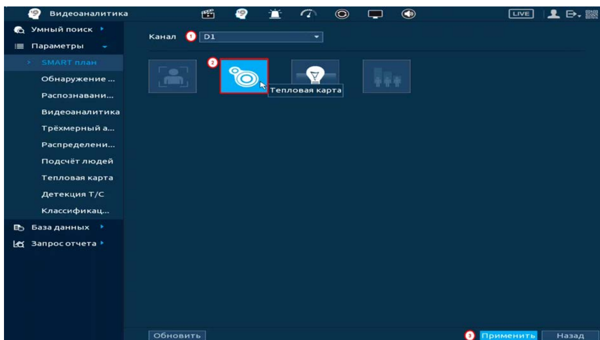
Рисунок 20.94 – Настройка
