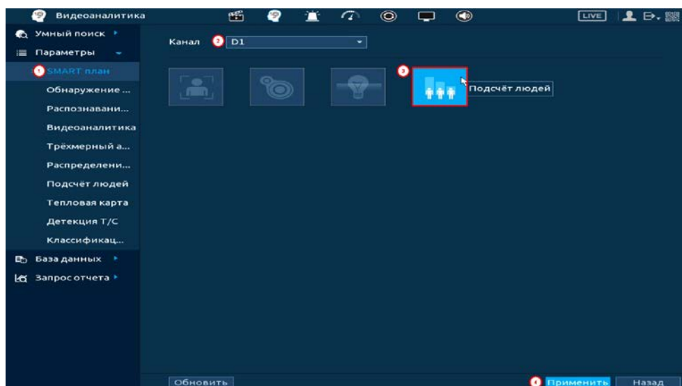
Рисунок 20.80 – Настройка
