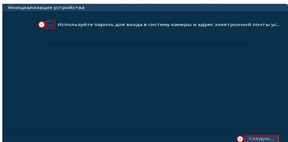
Рисунок 12.11 – Инициализация
