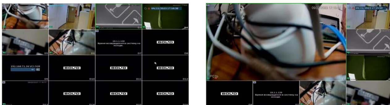
Рисунок 23.6 – Пример настройки
