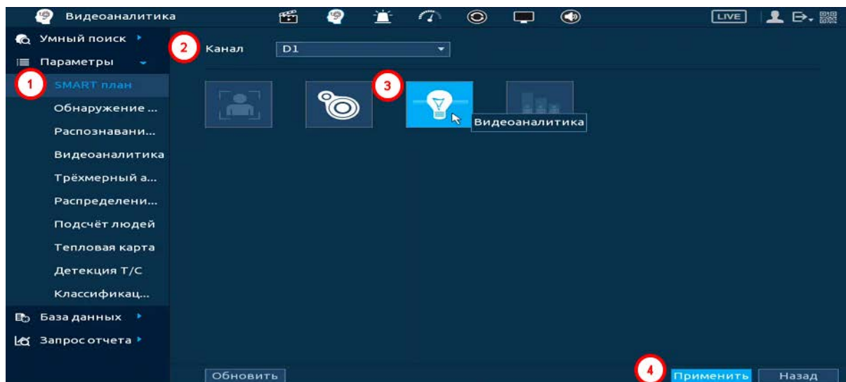
Рисунок 20.44 – Настройка
