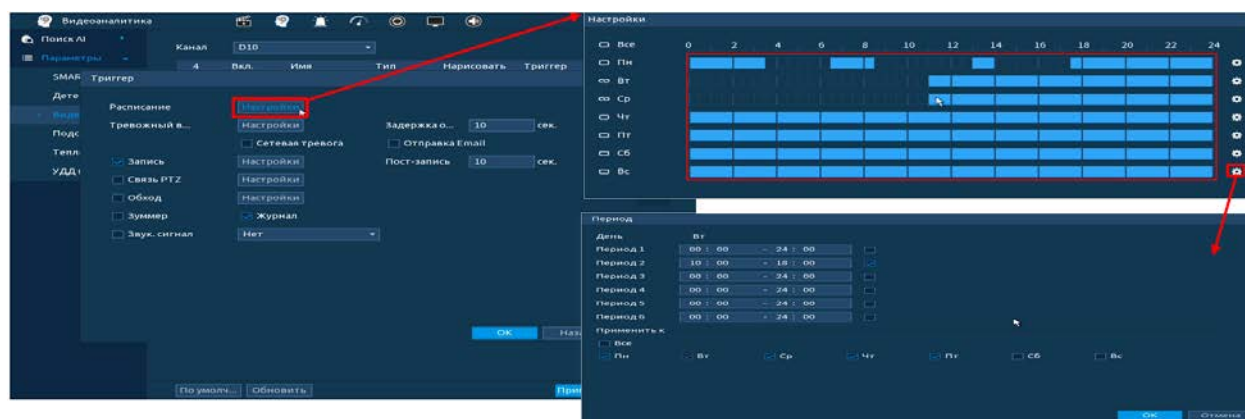
Рисунок 20.48 – Расписание
