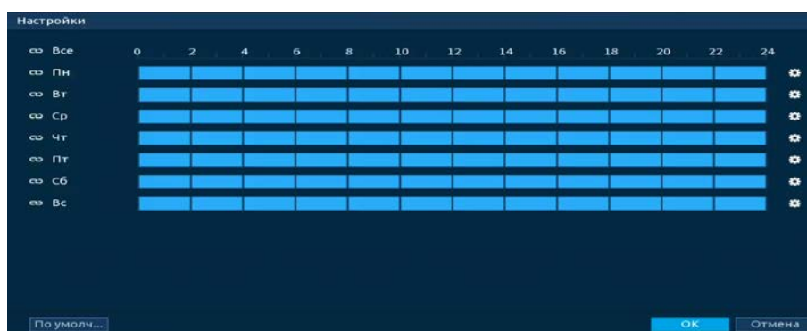
Рисунок 20.21 – Расписание
