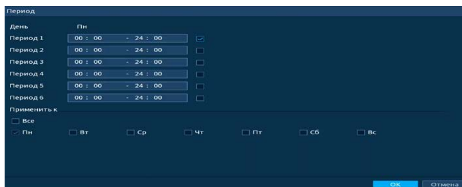
Рисунок 19.5 – Расписание
