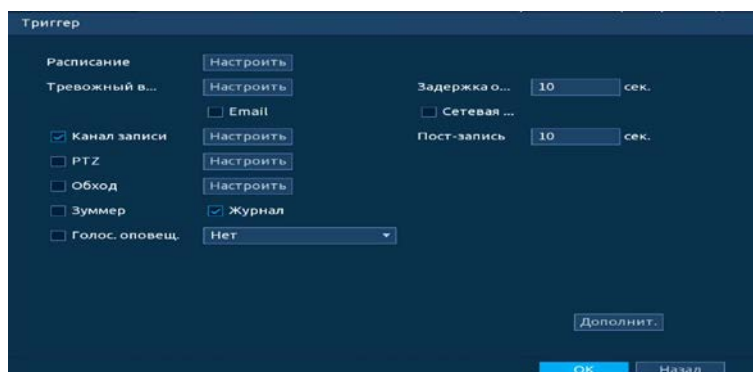
Рисунок 20.28 – Настройка
