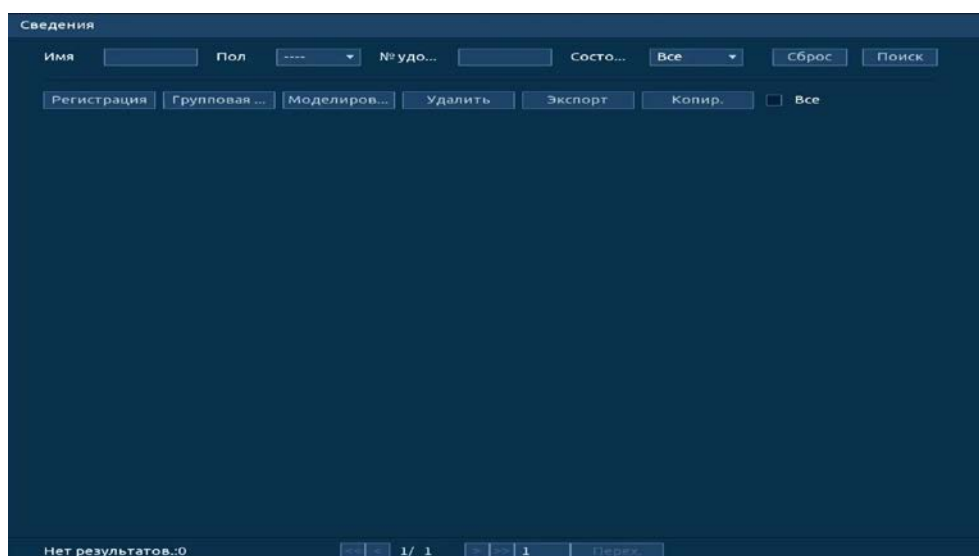
Рисунок 20.102 – Настройка
