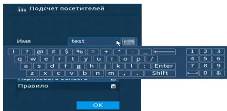
Рисунок 20.73 – Настройка
