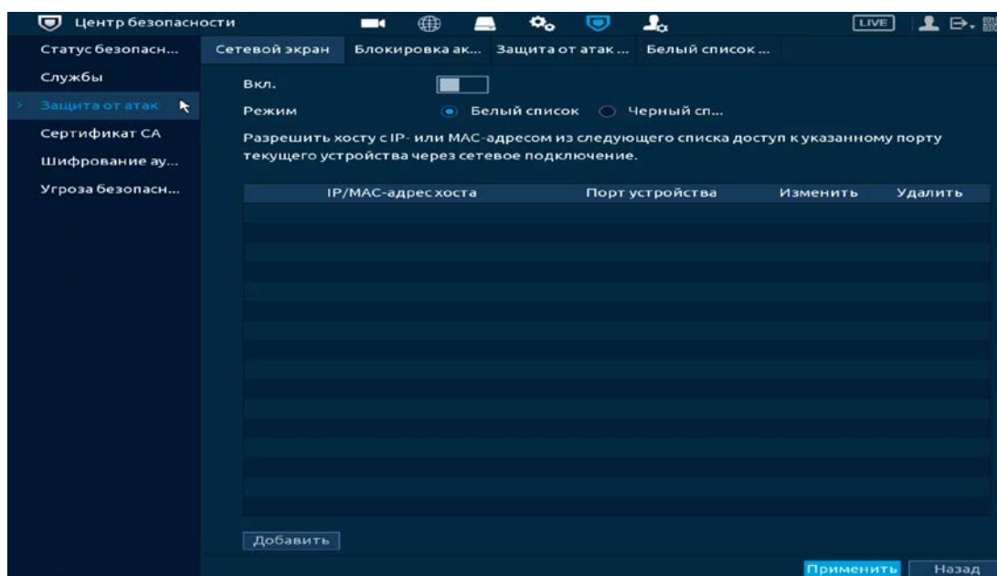
Рисунок 16.8 – Сетевой экран
