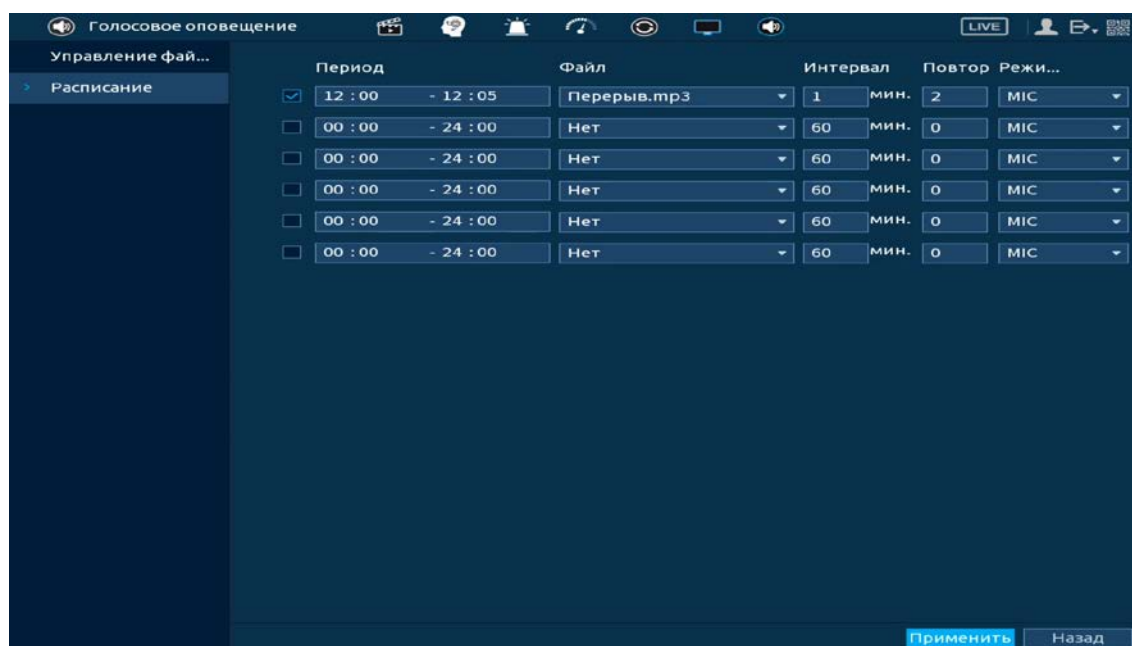
Рисунок 24.4 – Расписание
