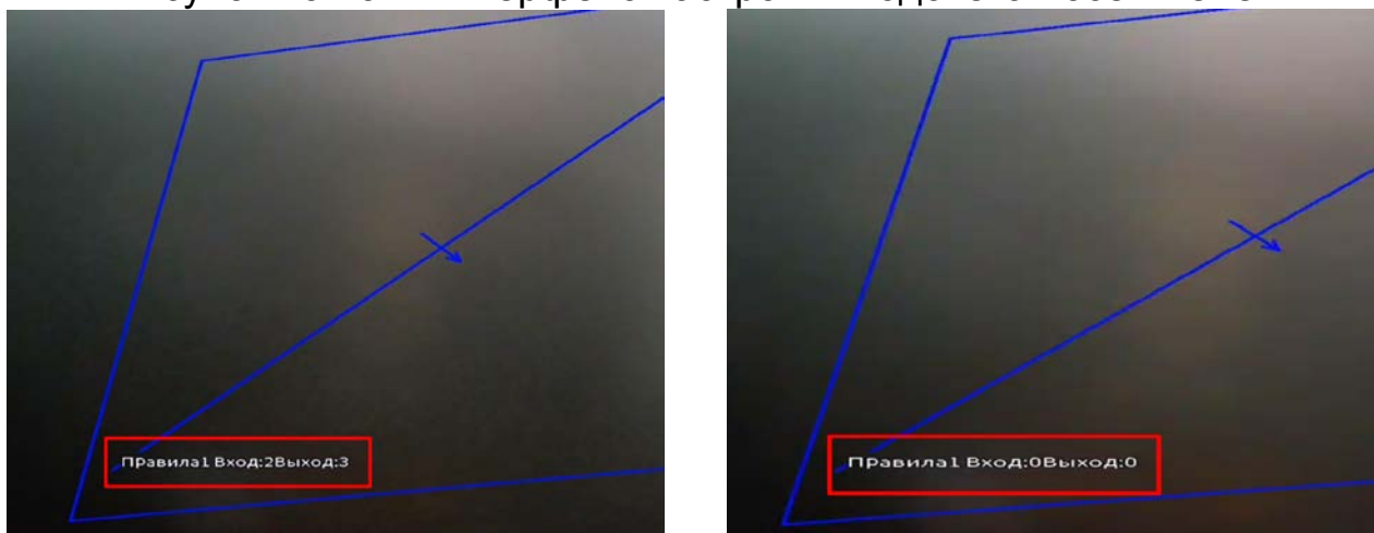
Рисунок 20.77 – Сброс
