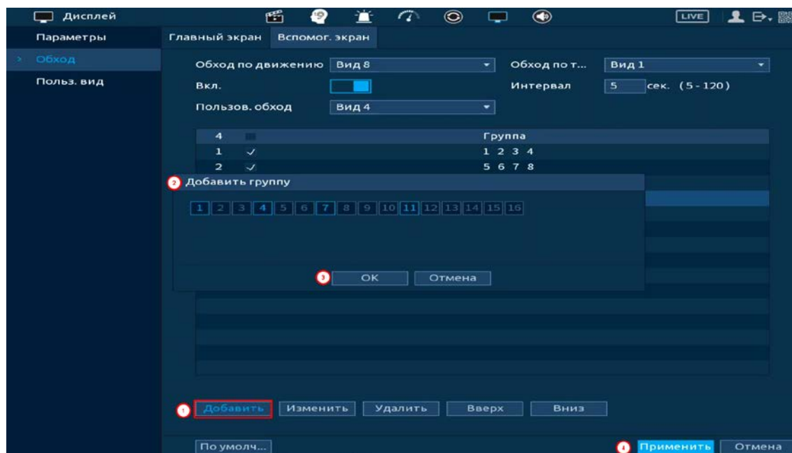
Рисунок 10.13 – Добавление группы
