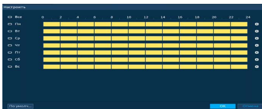
Рисунок 19.33 – Панель расписания
