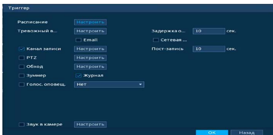
Рисунок 20.78 – Настройка параметров
