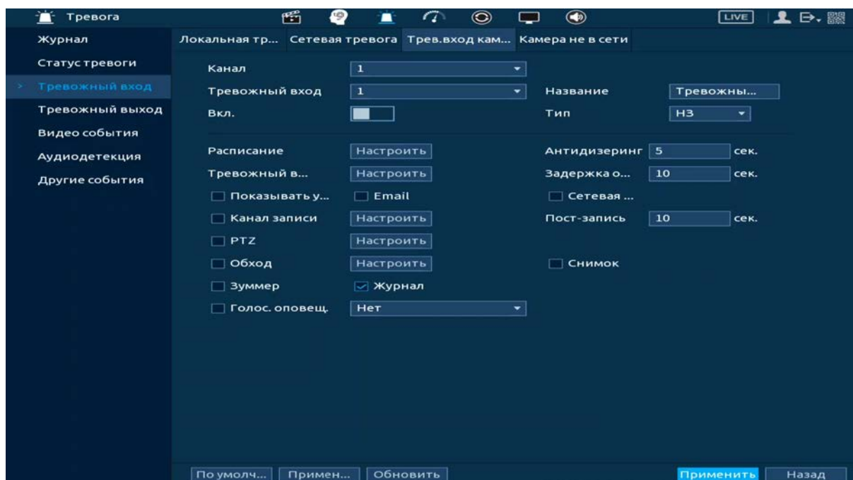
Рисунок 19.11 – Интерфейс настройки
