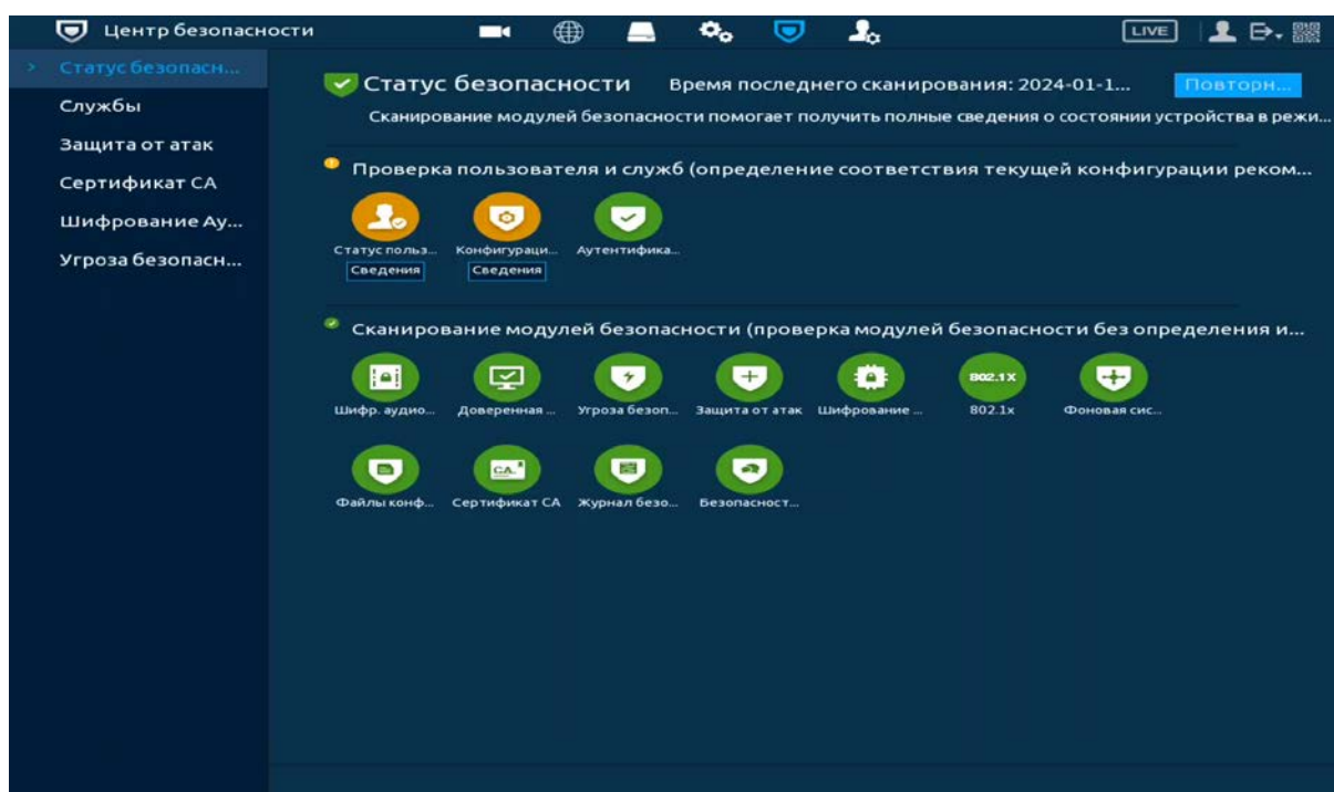
Рисунок 16.1 – Статус безопасности
