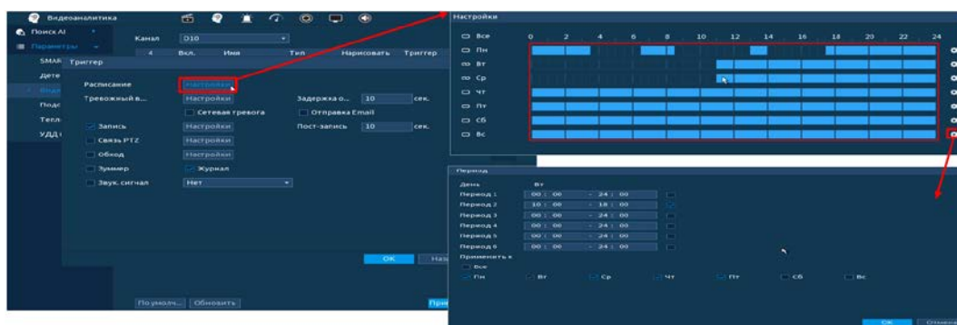
Рисунок 20.68 – Расписание
