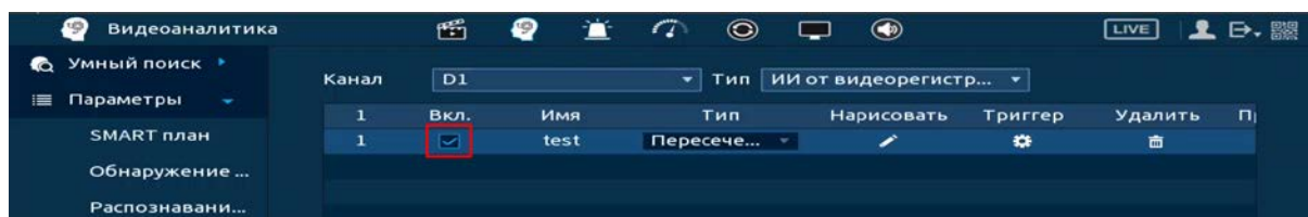
Рисунок 20.27 – Настройка
