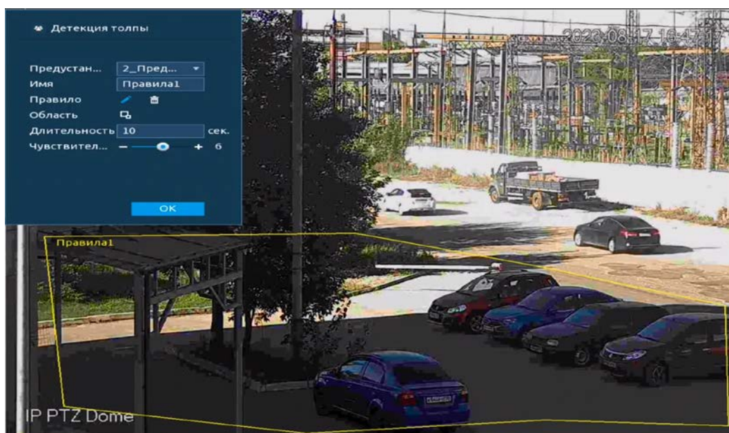
Рисунок 20.61 – Настройка правила
