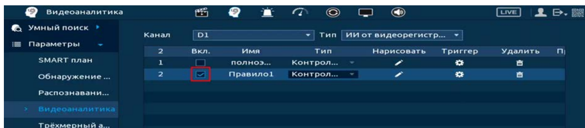
Рисунок 20.35 – Настройка
