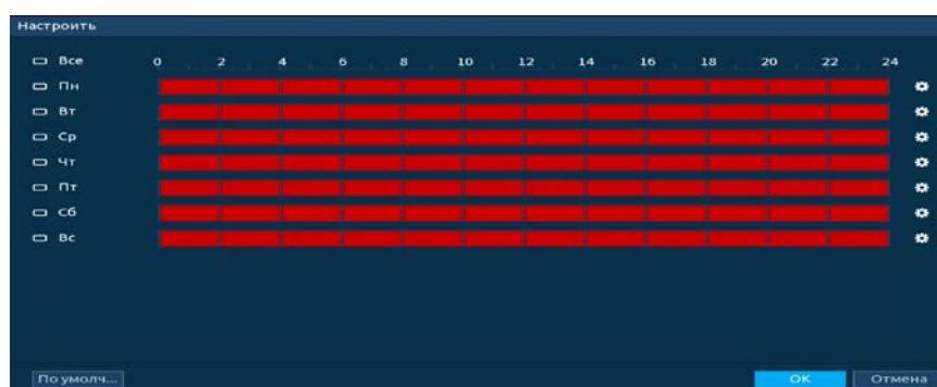
Рисунок 19.4 – Панель расписания
