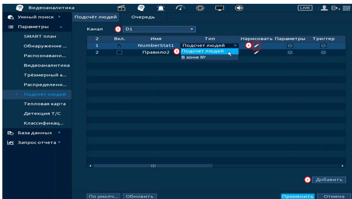
Рисунок 20.72 – Настройка
