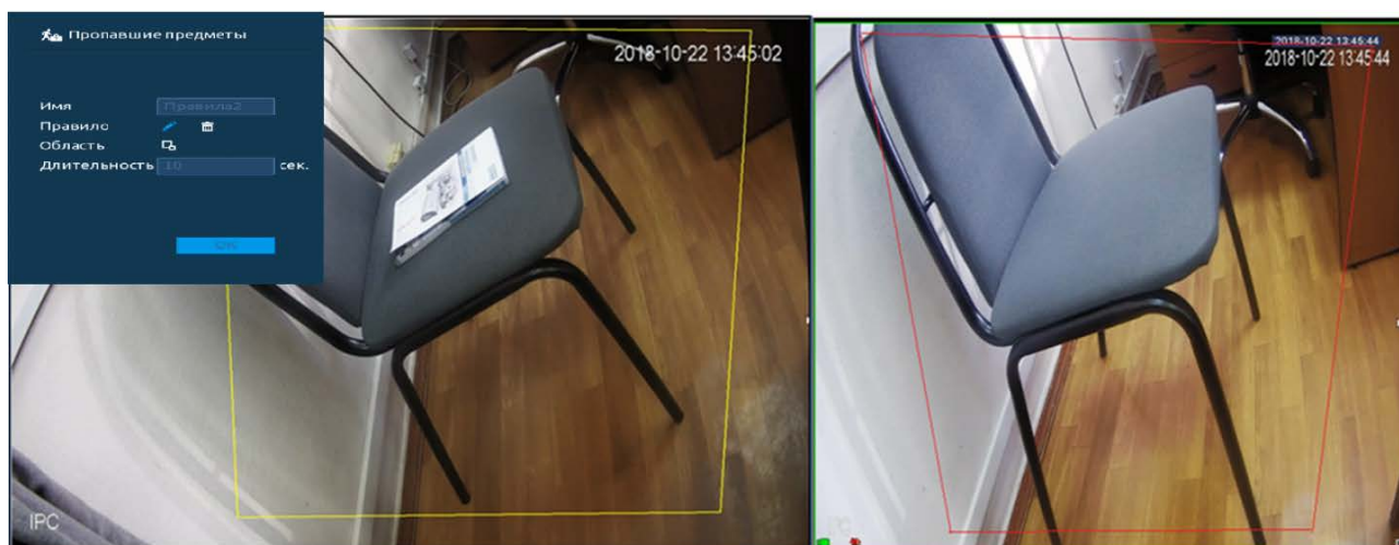
Рисунок 20.46 – Настройка функции
