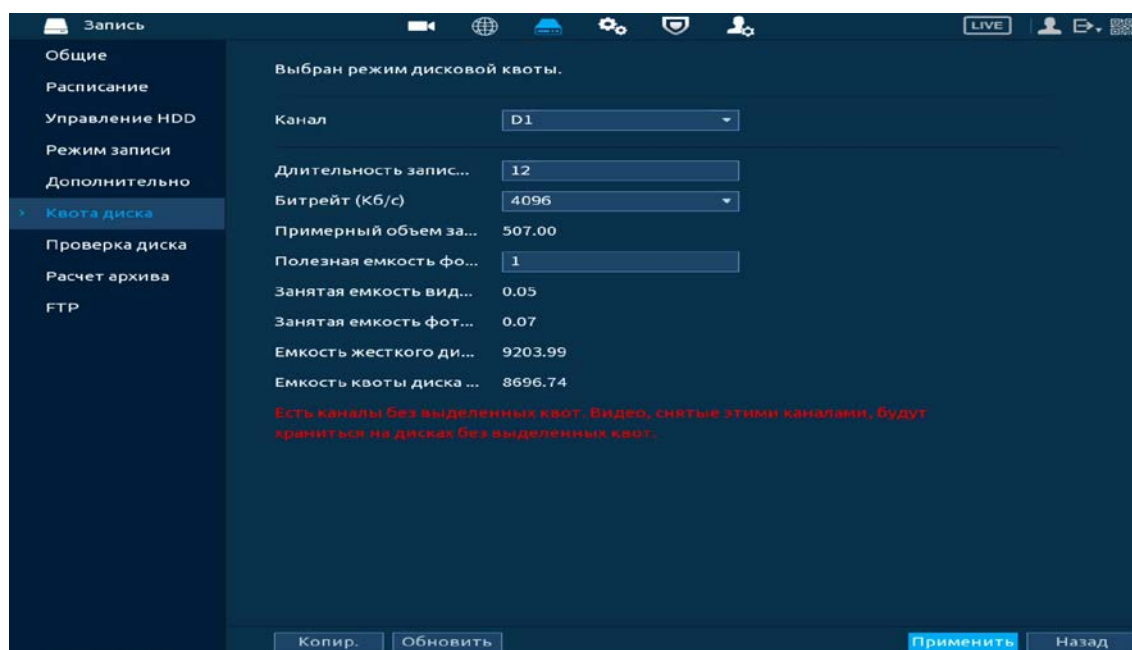
Рисунок 14.22 – Квота диска
