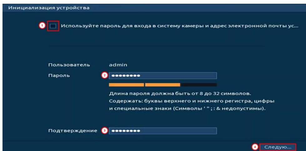
Рисунок 12.12 – Инициализация
