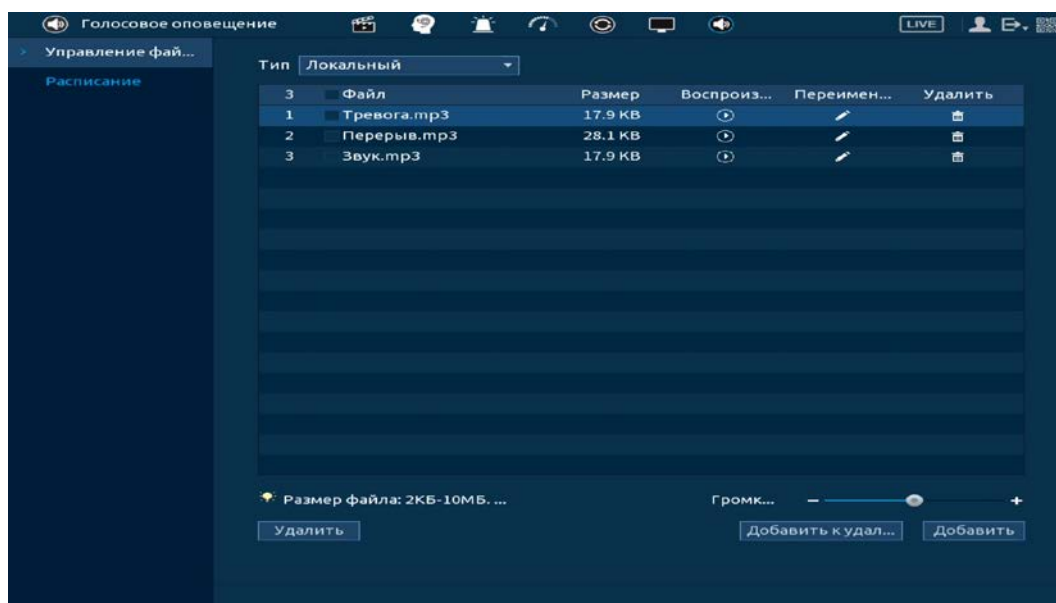
Рисунок 24.1 – Управление файлами
