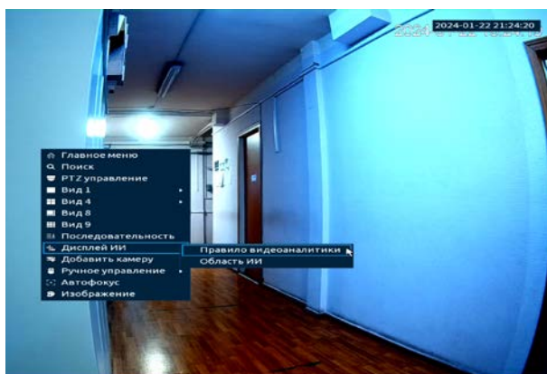
Рисунок 8.9 – Отображение видеоаналитики
