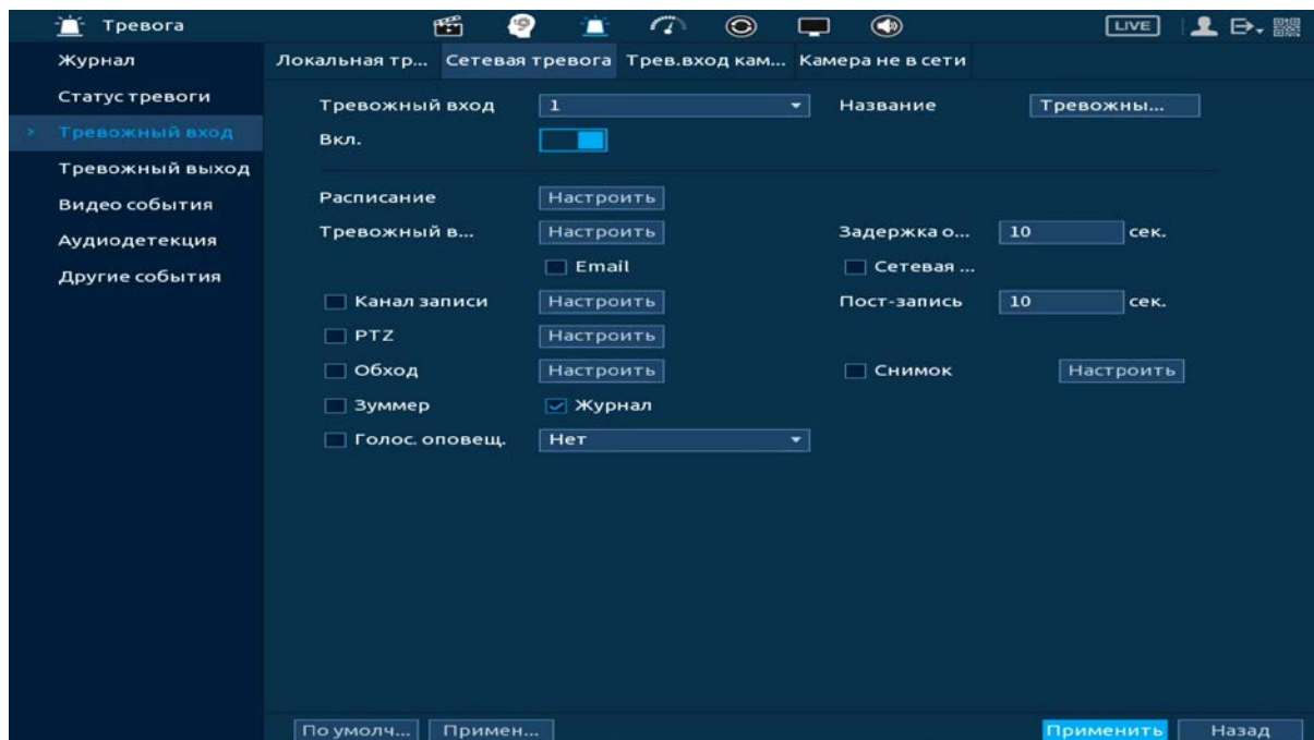
Рисунок 19.7 – Интерфейс настройки
