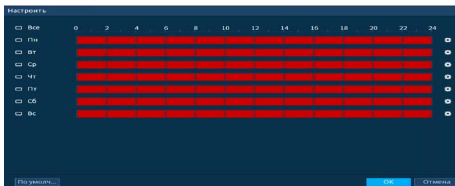
Рисунок 19.8 – Панель расписания
