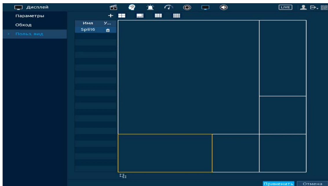
Рисунок 23.22 – Создание раскладки
