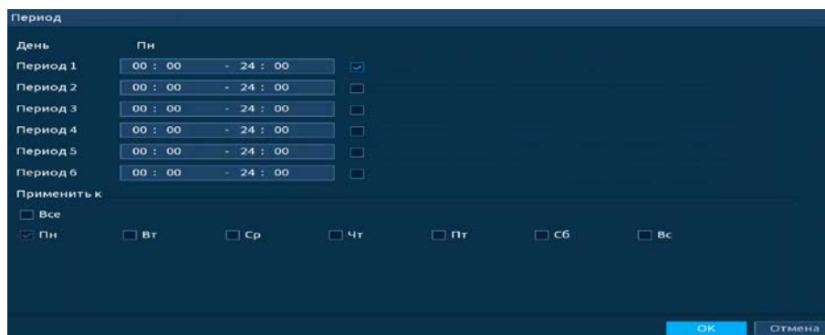
Рисунок 19.34 – Расписание
