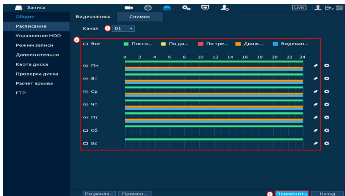
Рисунок 14.12 – Настройка расписания снимка на устройстве
