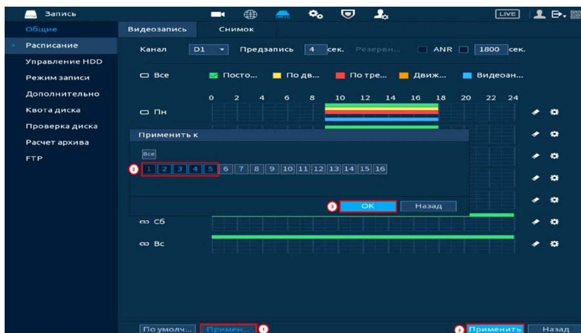
Рисунок 14.10 – Копирование настроек на другие каналы
