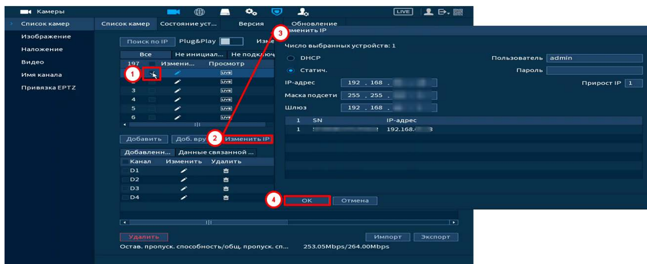
Рисунок 12.21 – Изменения сетевых настроек IP-камер через регистратор
