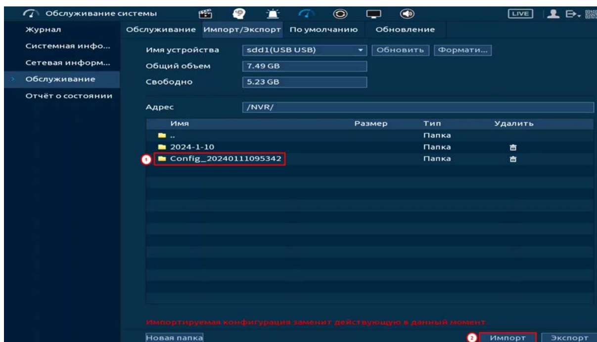
Рисунок 21.15 – Импорт настроек на регистратор
