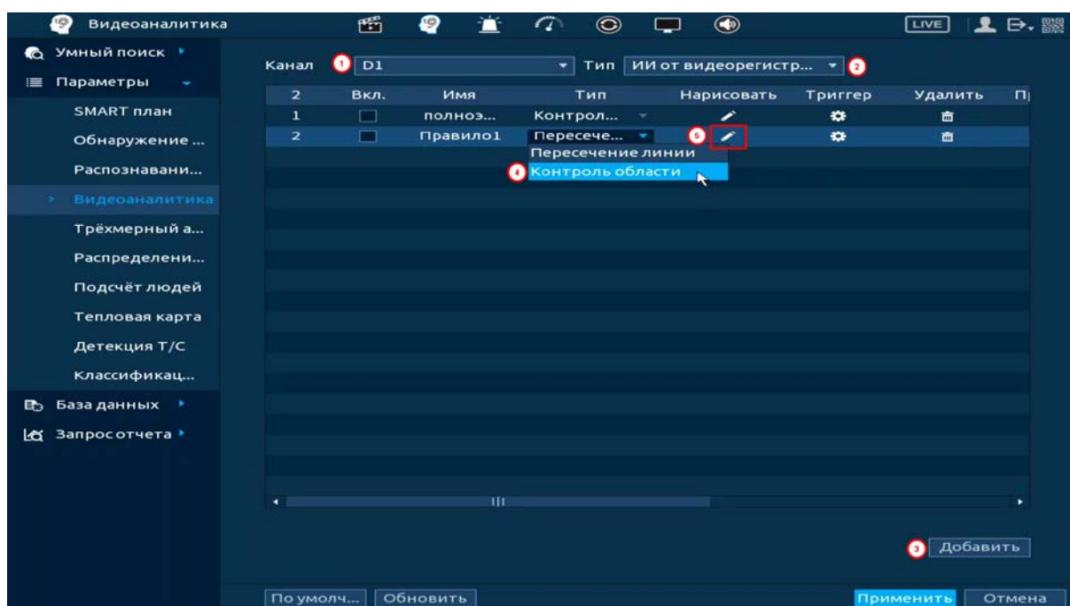
Рисунок 20.32 – Функция видеоаналитики «Контроль области»
