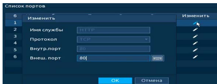
Рисунок 13.9 – Интерфейс настройки «UPnP»
