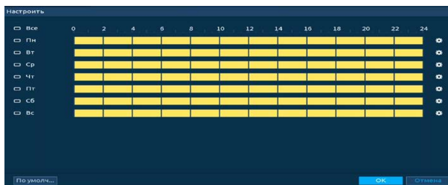
Рисунок 19.36 – Панель расписания
