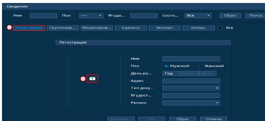
Рисунок 20.103 – Регистрация
