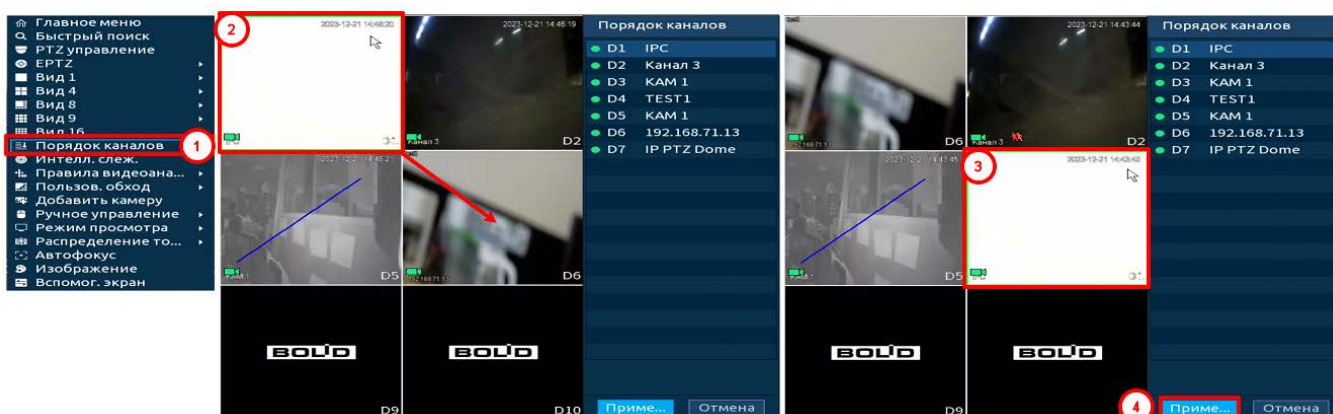
Рисунок 8.7 – Изменение раскладки
