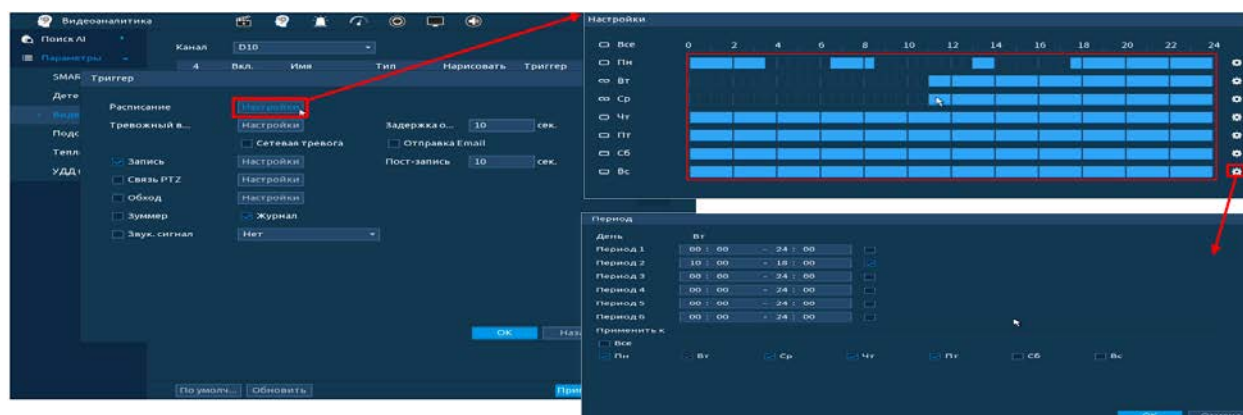
Рисунок 20.63 – Расписание
