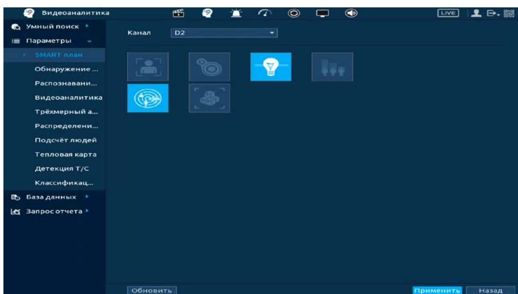
Рисунок 20.6 – Выбор функции
