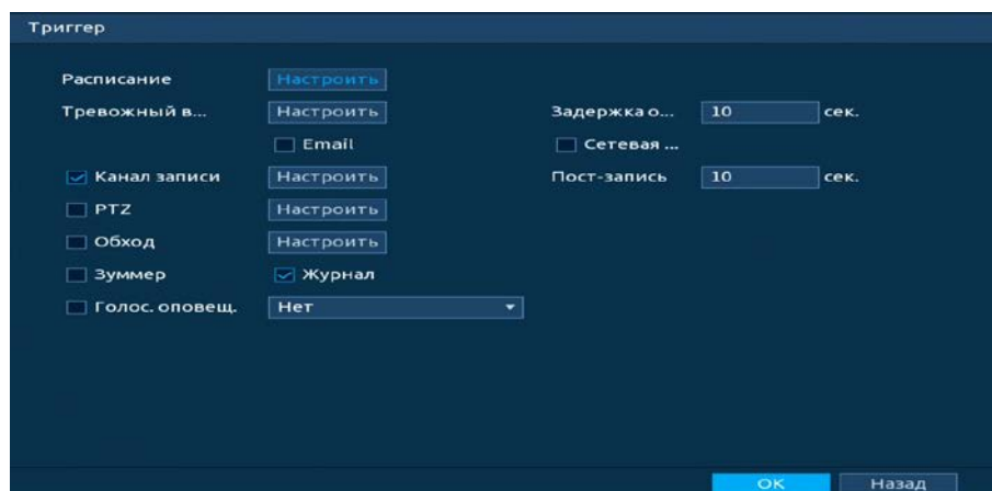
Рисунок 20.92 – Настройка параметров
