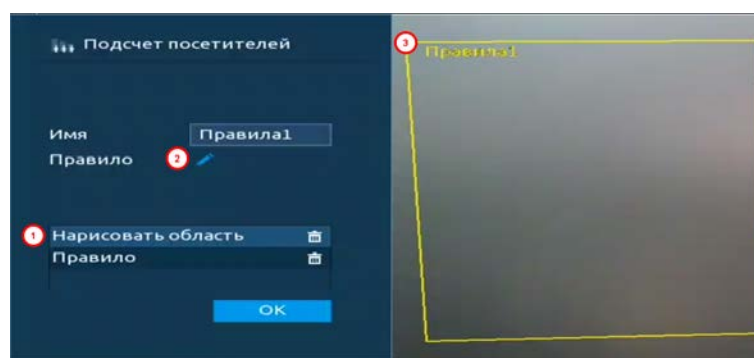
Рисунок 20.74 – Нарисовать область
