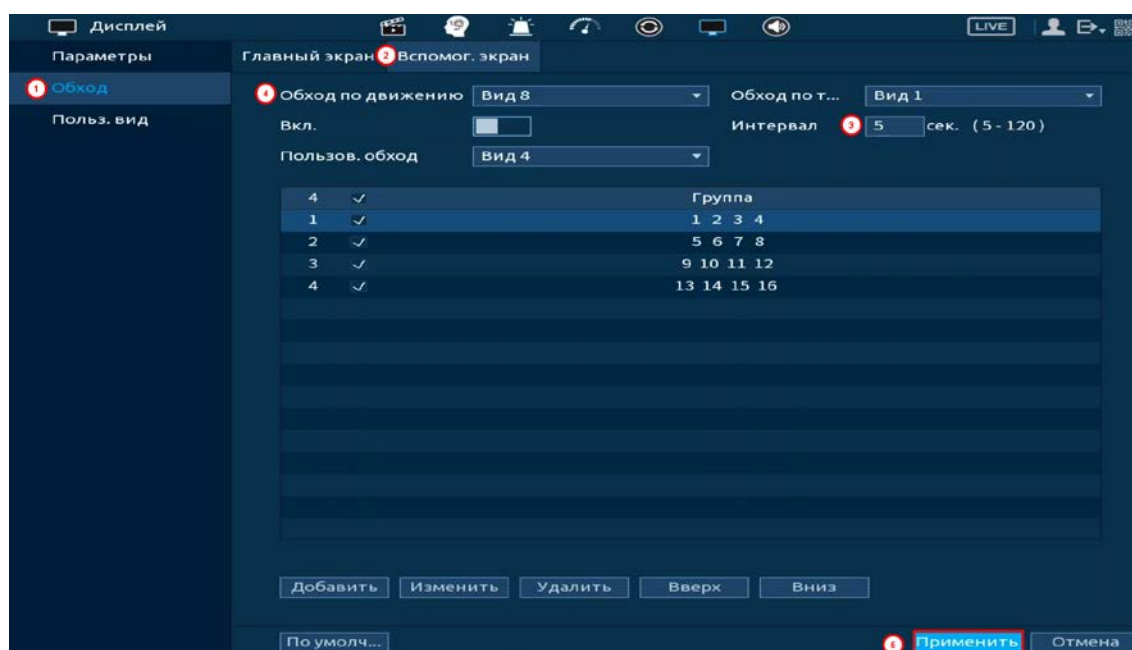
Рисунок 23.14 – Пример настройки
