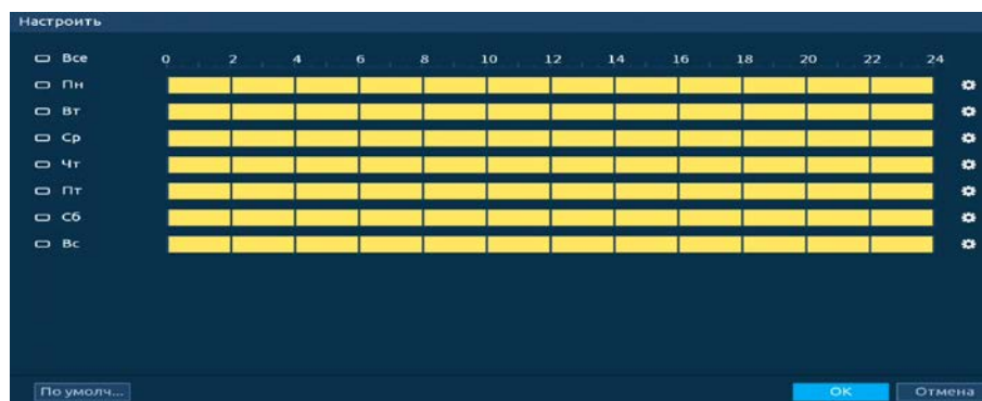
Рисунок 19.21 – Расписание
