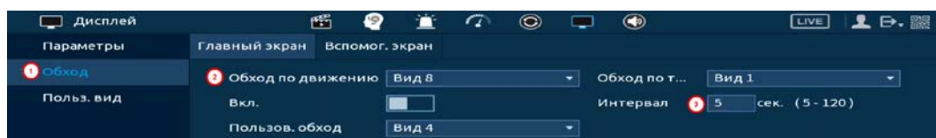
Рисунок 23.4 – Пример настройки
