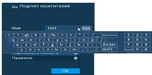
Рисунок 20.82 – Настройка
