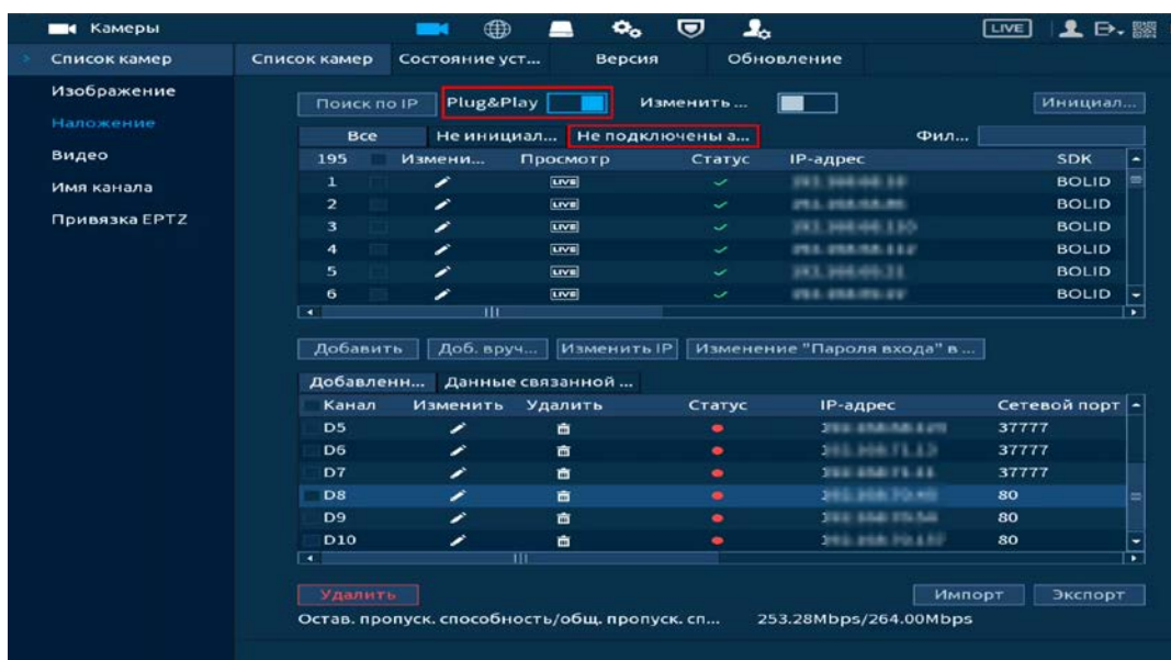
Рисунок 12.6 – Plug&Play
