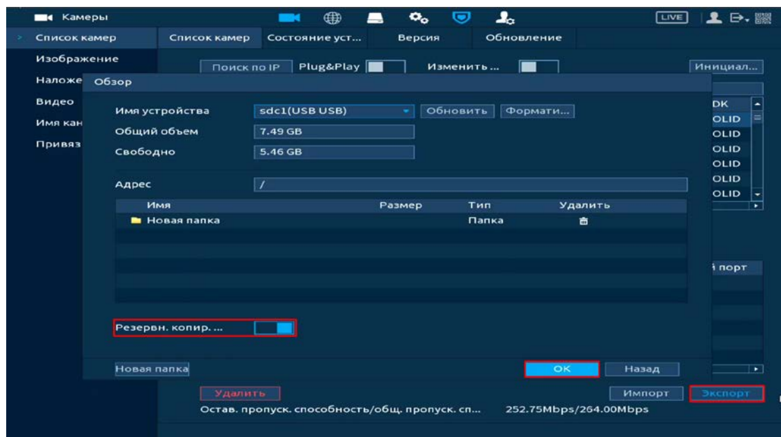
Рисунок 12.22 – Экспорт
