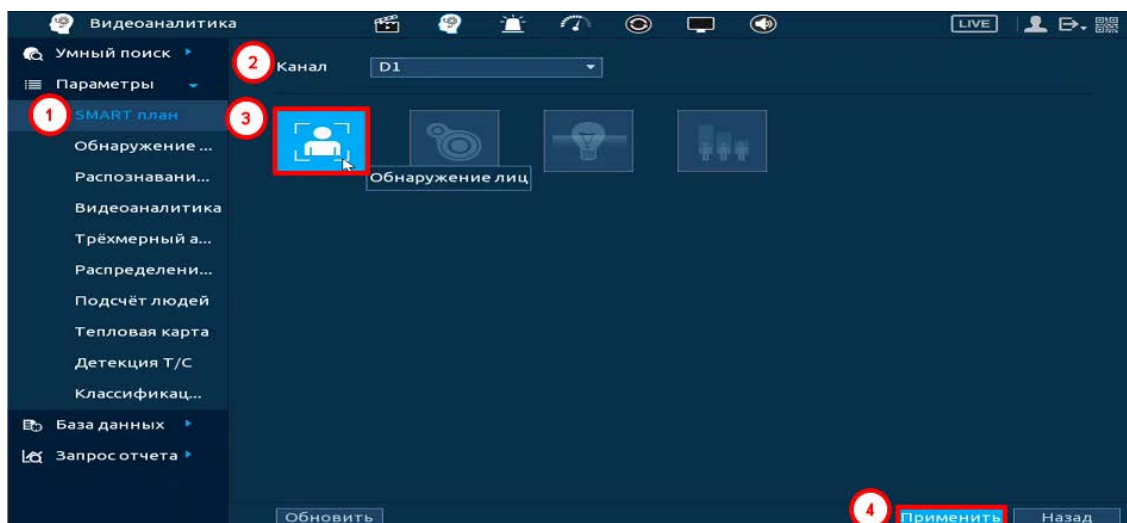
Рисунок 20.9 – Настройка
