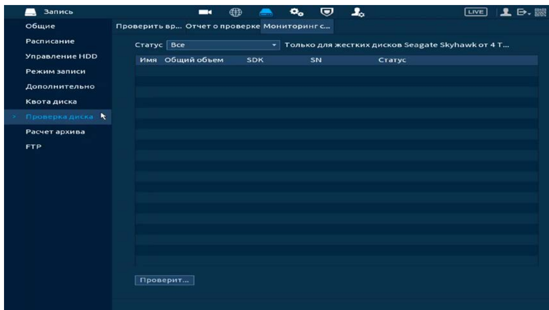
Рисунок 14.25 – Мониторинг состояния
