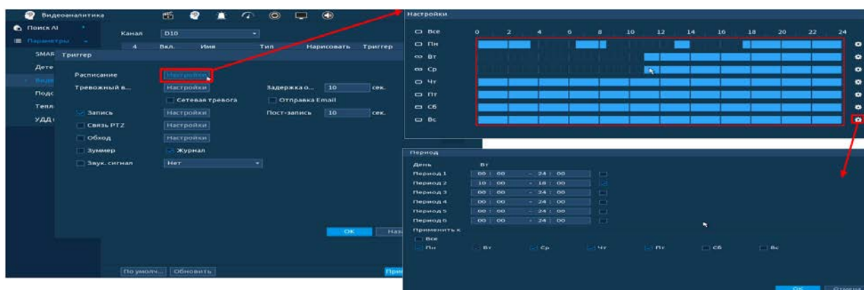
Рисунок 20.53 – Расписание
