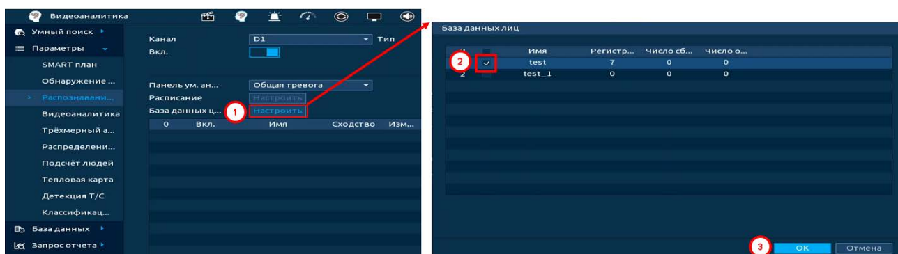
Рисунок 20.15 – Настройка
