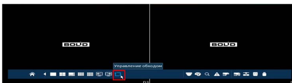
Рисунок 23.12 – Выключение/включение обхода
