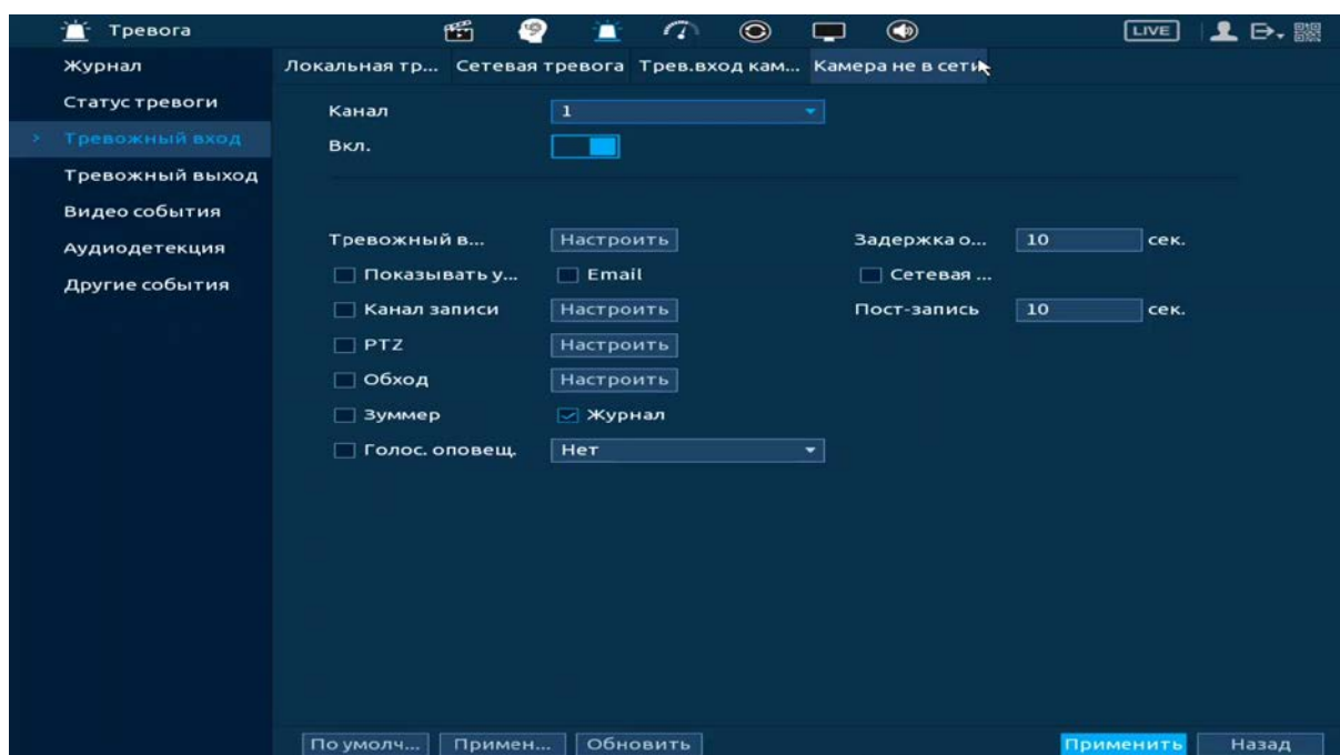
Рисунок 19.15 – Интерфейс настройки
