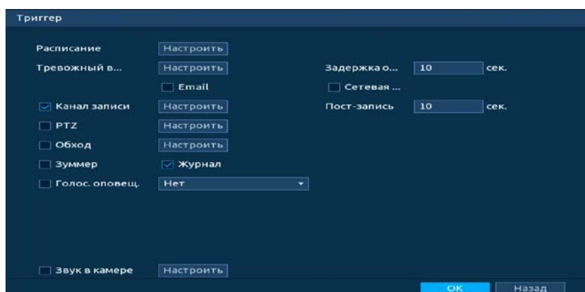
Рисунок 20.67 – Настройка параметров
