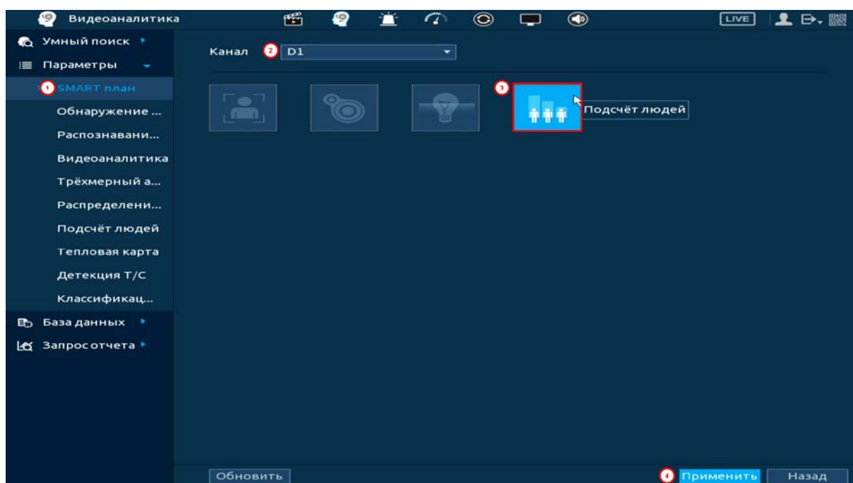
Рисунок 20.87 – Настройка
