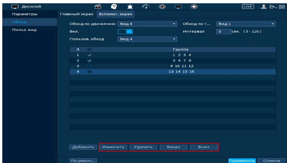
Рисунок 23.19 – Расположение групп
