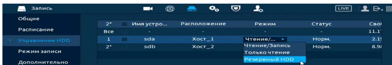
Рисунок 14.4 – Управление HDD
