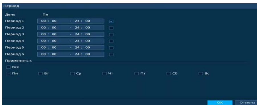
Рисунок 19.9 – Расписание
