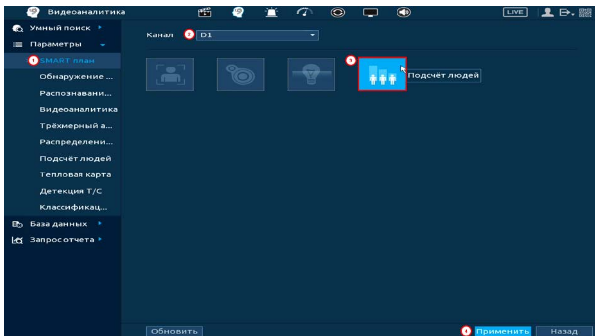
Рисунок 20.71 – Настройка
