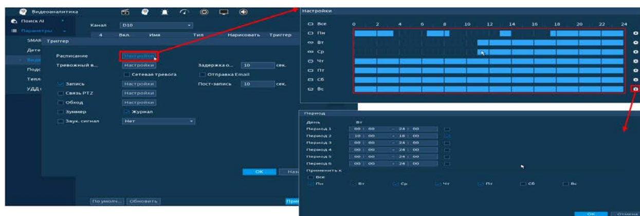
Рисунок 20.93 – Расписание
