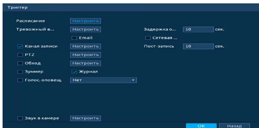
Рисунок 20.85 – Настройка параметров
