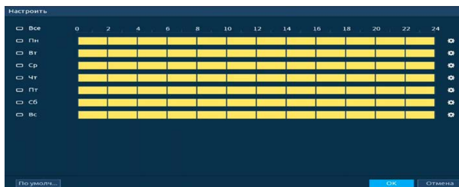
Рисунок 19.29 – Панель расписания
