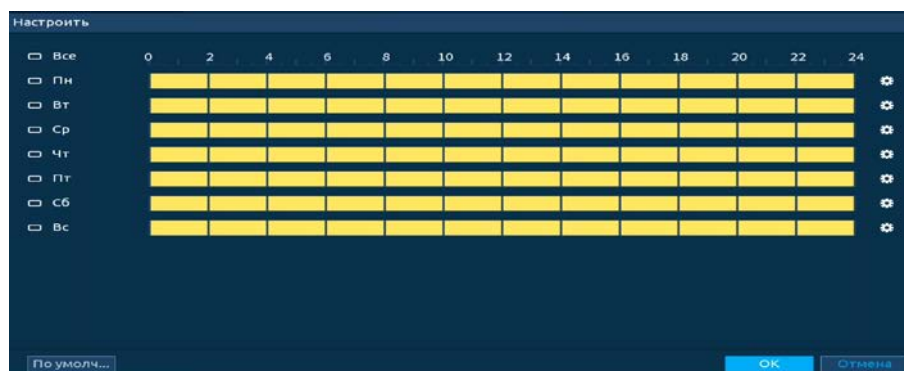
Рисунок 19.39 – Панель расписания
