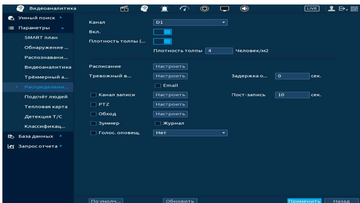
Рисунок 20.69 – Распределение толпы
