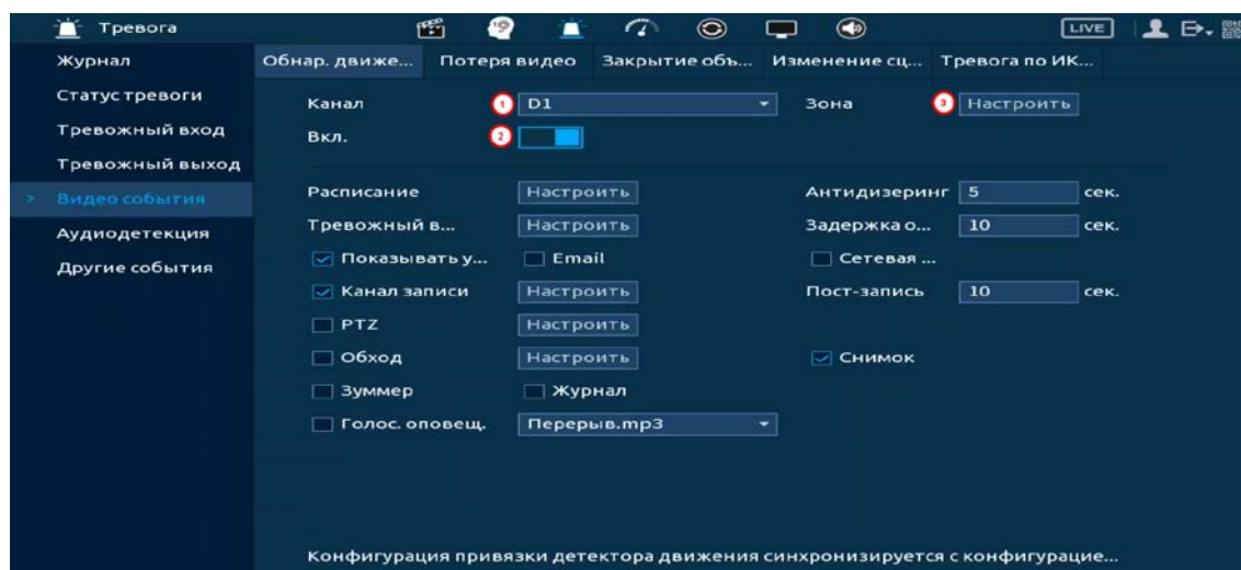
Рисунок 19.19 – Настройка события
