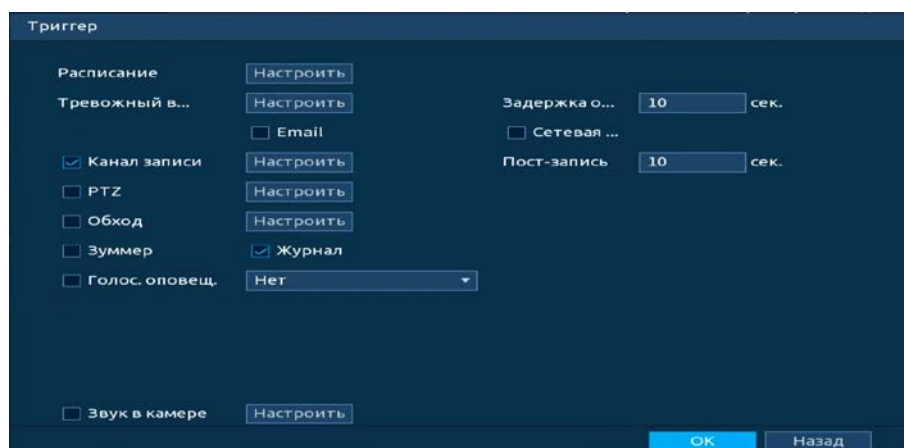
Рисунок 20.57 – Настройка параметров
