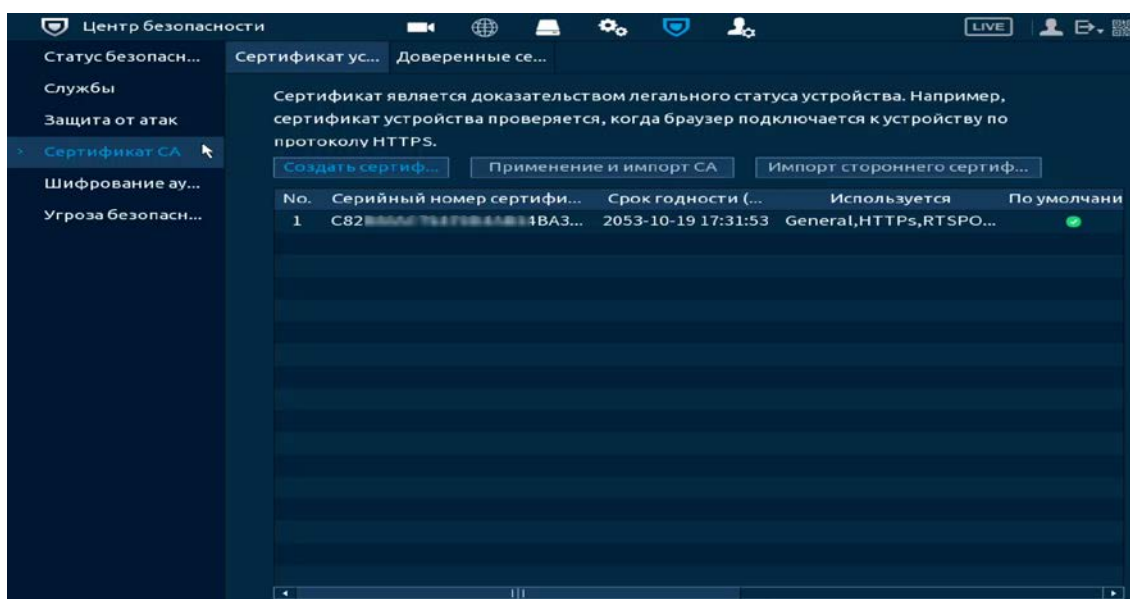
Рисунок 16.16 – Сертификат устройства
