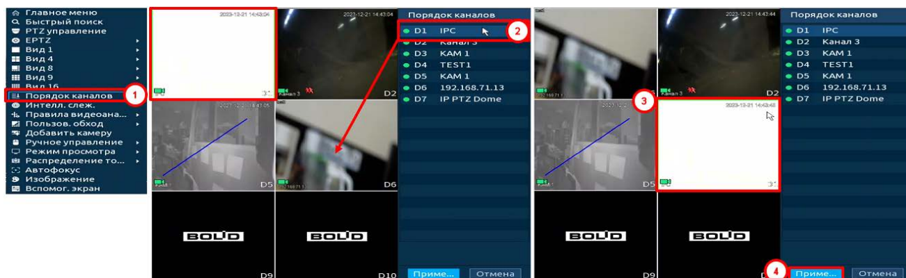
Рисунок 8.6 – Изменение раскладки
