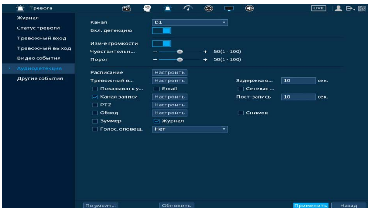
Рисунок 19.38 – Настройка аудиодетекции
