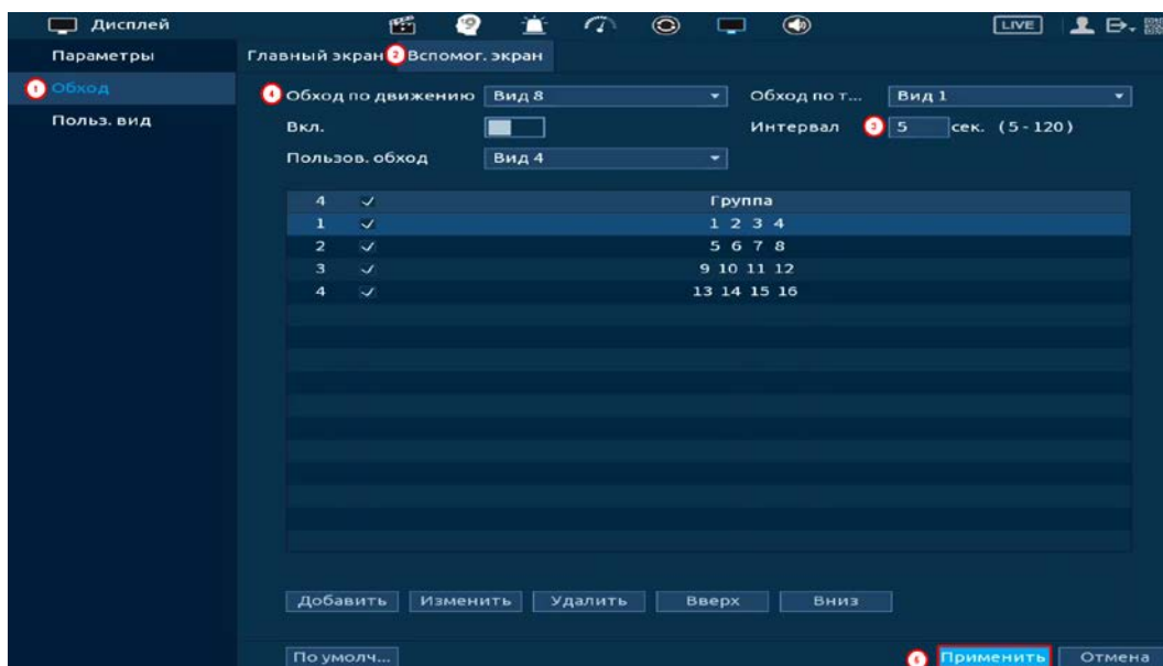
Рисунок 10.7 – Пример настройки
