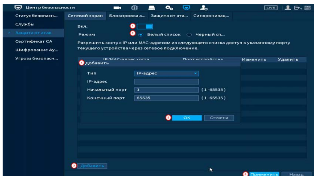
Рисунок 16.9 – Добавить
