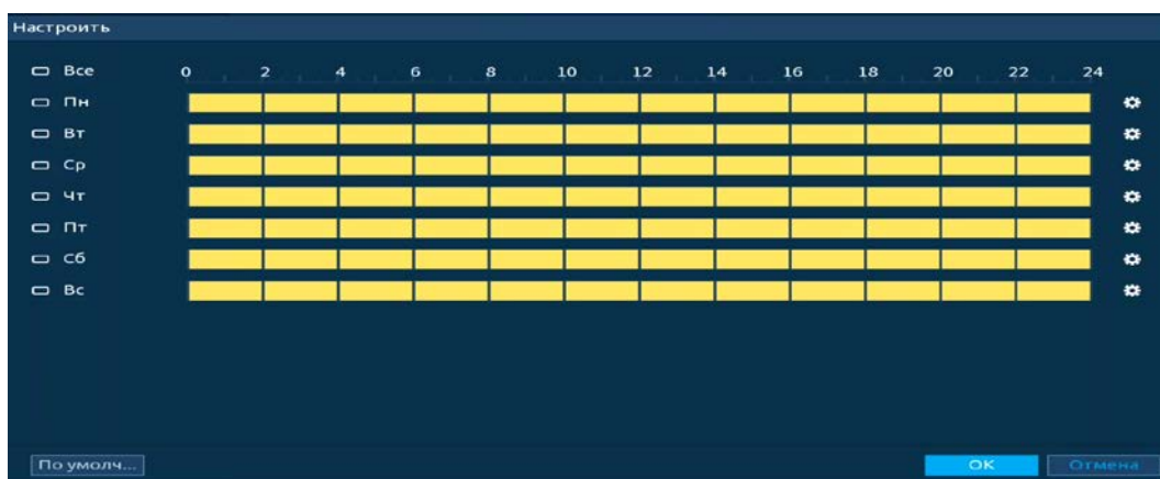
Рисунок 19.25 – Панель расписания
