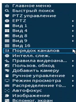
Рисунок 8.5 – Контекстное меню
