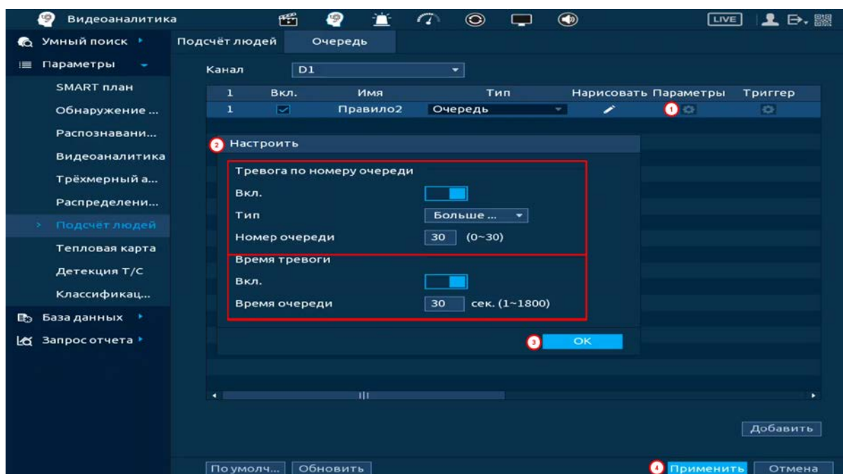
Рисунок 20.91 – Настройка параметров
