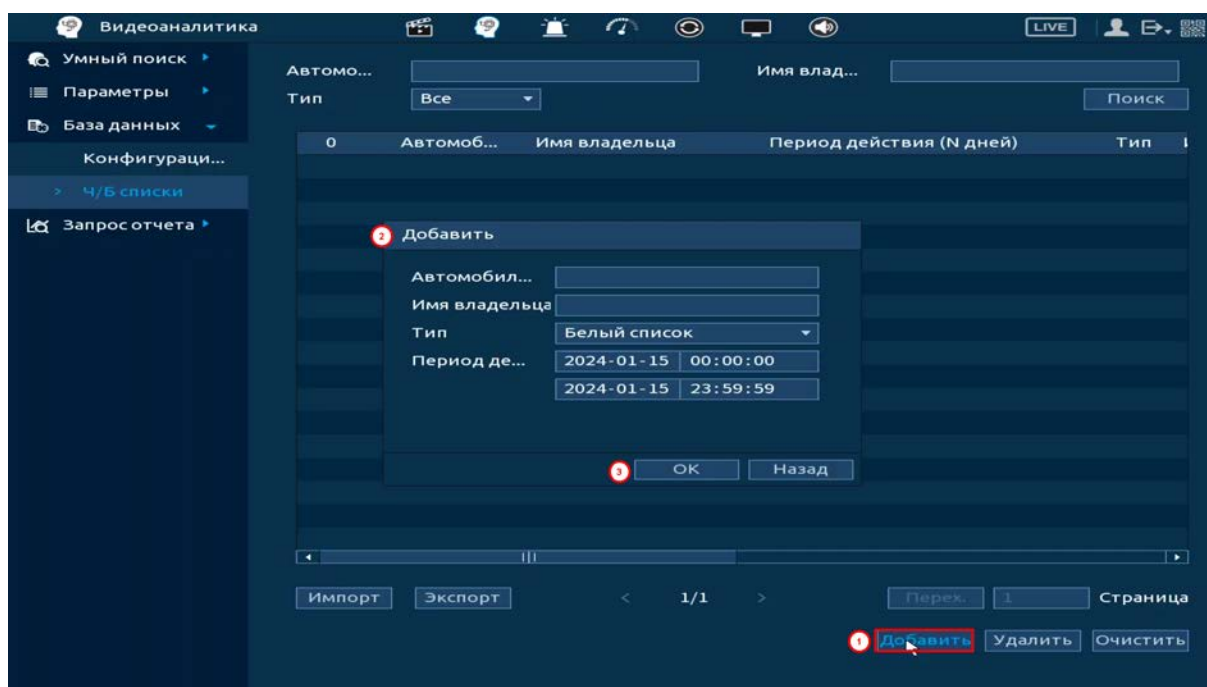
Рисунок 20.107 – Ч/Б список
