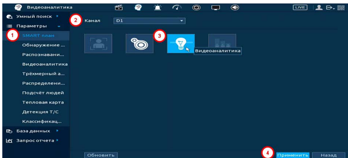
Рисунок 20.64 – Настройка
