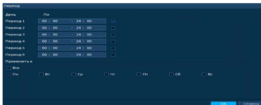
Рисунок 19.40 – Расписание
