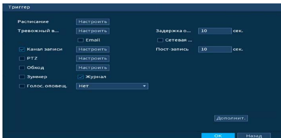
Рисунок 20.36 – Настройка
