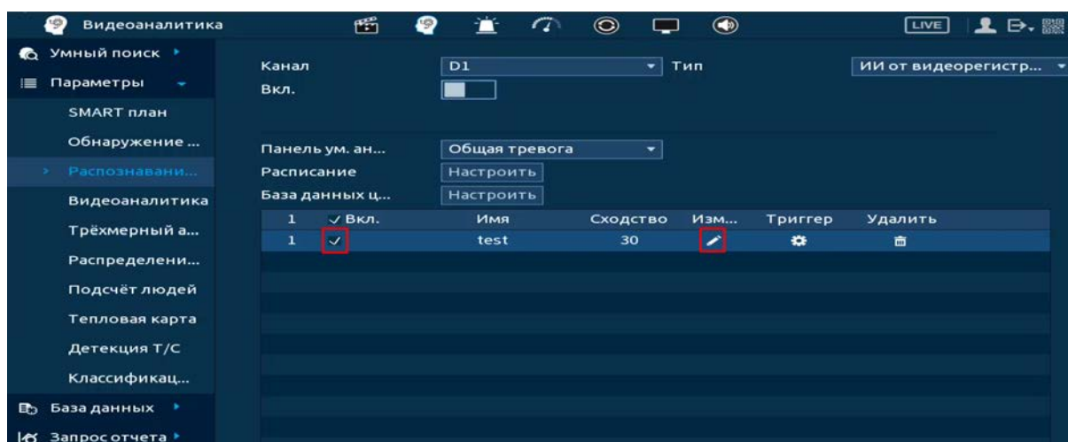
Рисунок 20.16 – Настройка
