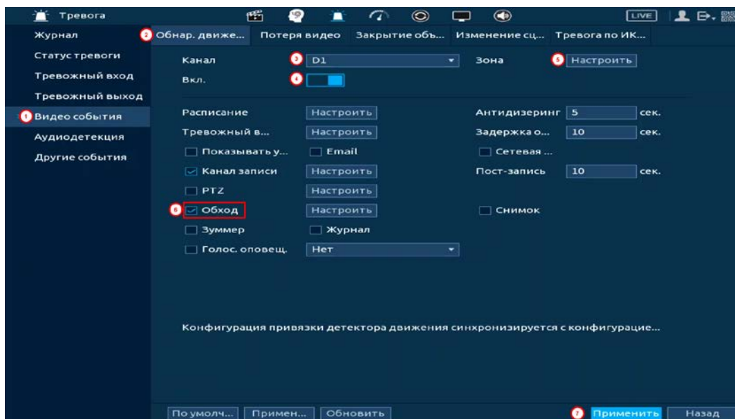
Рисунок 23.15 – Пример настройки
