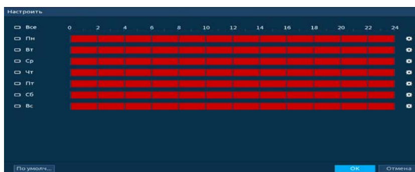
Рисунок 19.12 – Панель расписания
