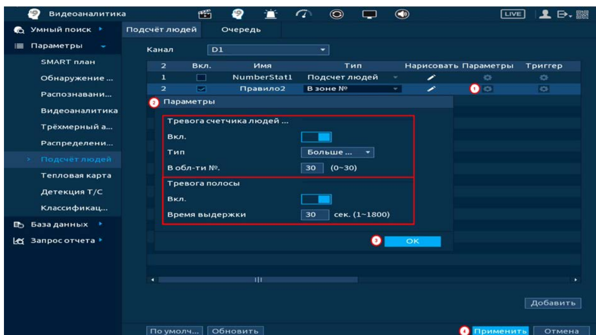
Рисунок 20.84 – Настройка параметров
