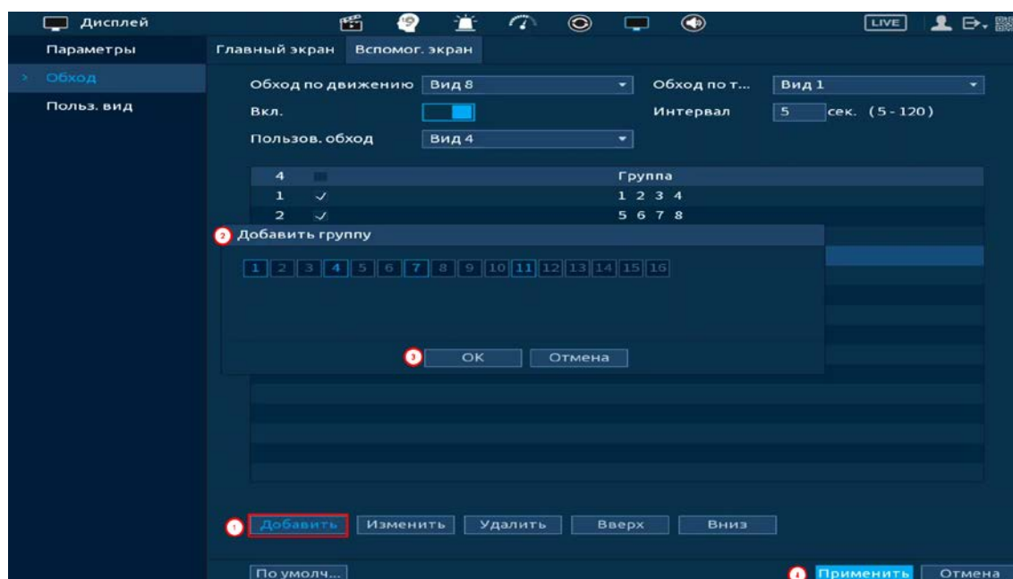
Рисунок 23.20 – Добавление группы
