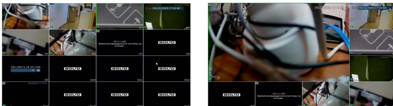
Рисунок 23.16 – Пример настройки
