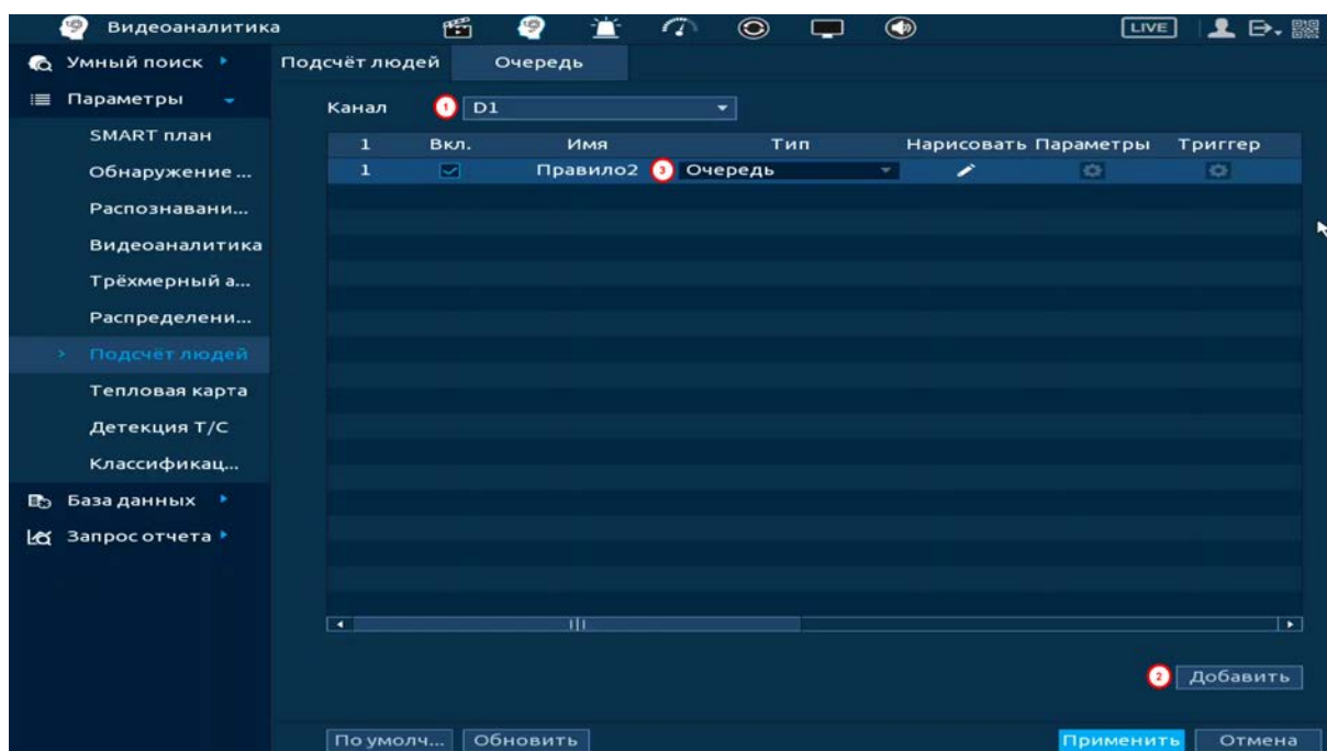
Рисунок 20.88 – Настройка
