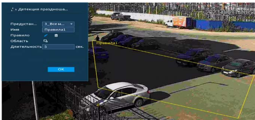
Рисунок 20.66 – Настройка правила
