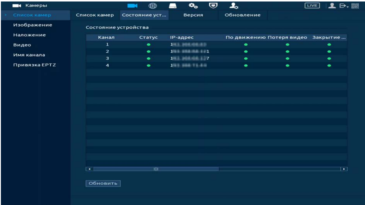
Рисунок 12.23 – Интерфейс просм
