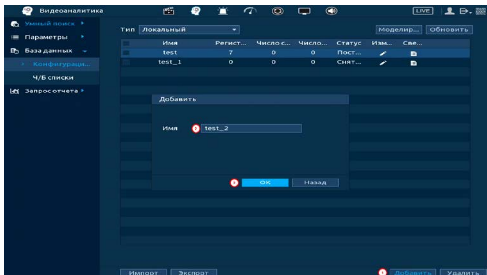
Рисунок 20.101 – Настройка
