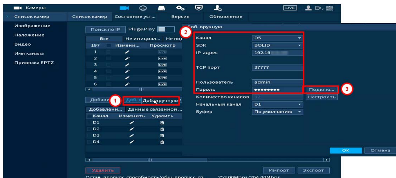
Рисунок 12.18 – Добавление видеопотока с другого регистратора
