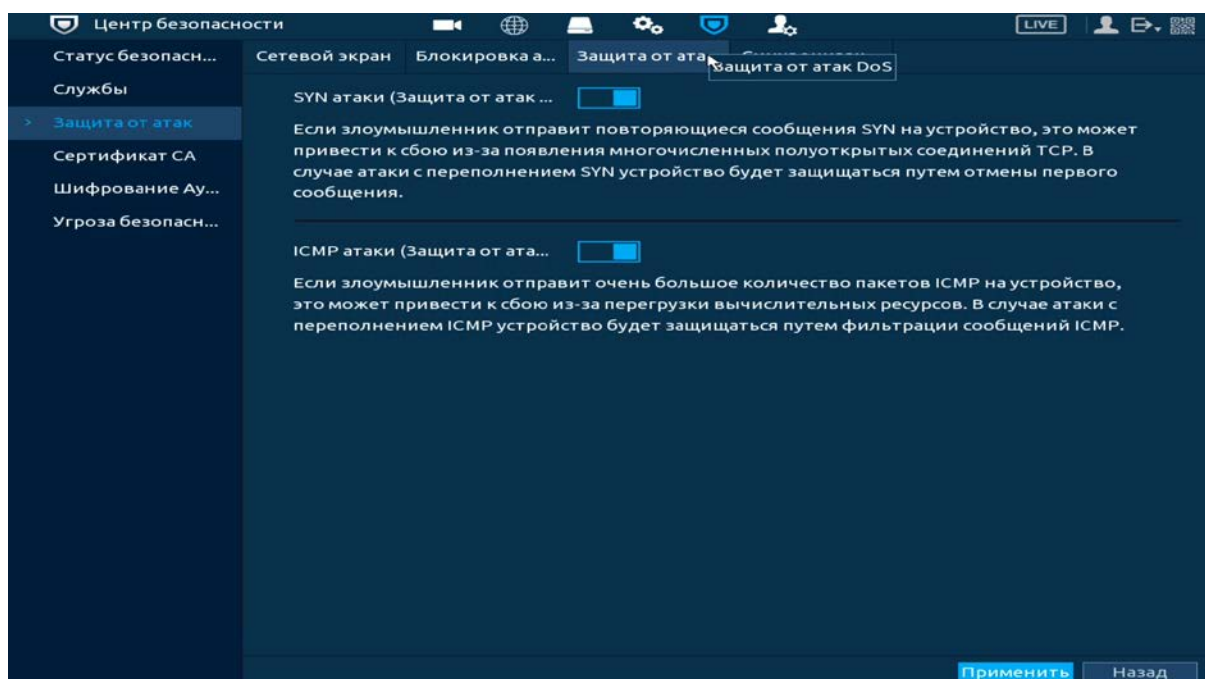
Рисунок 16.14 – Включение защиты от DoS атак
