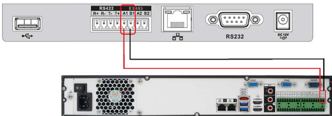
Рисунок 14.4 – Схема RS-485
