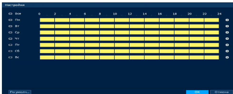
Рисунок 19.39 – Панель расписания
