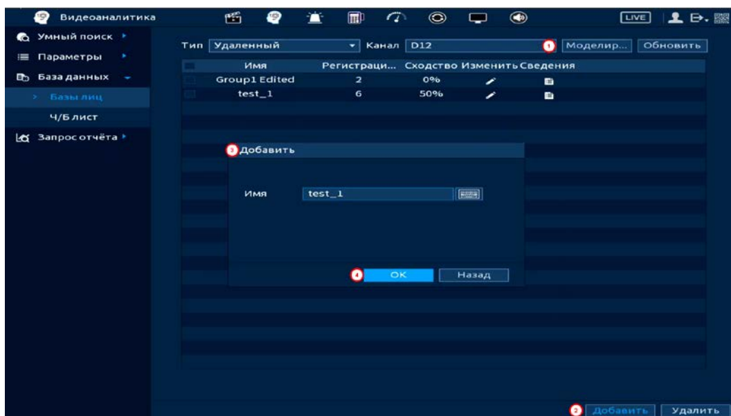
Рисунок 20.2 – Настройка
