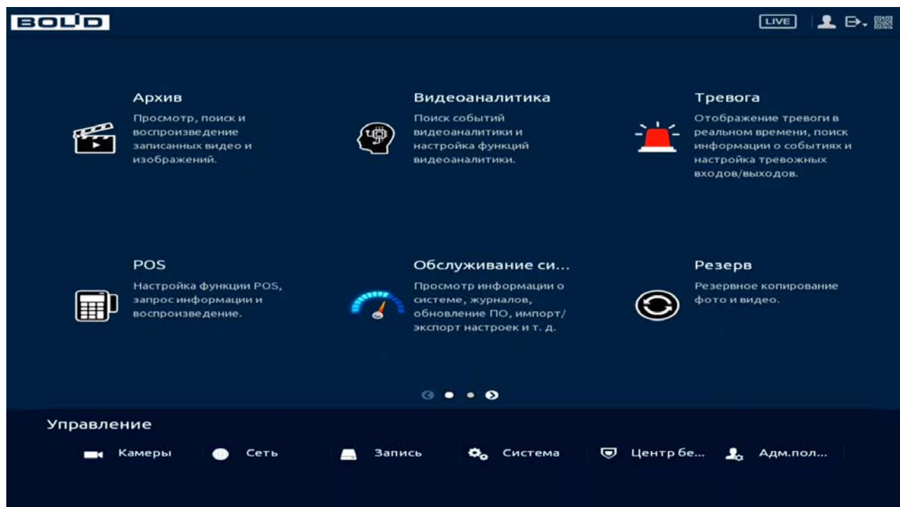
Рисунок 11.1 – Главное меню
