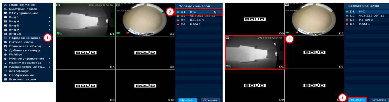
Рисунок 8.6 – Изменение раскладки
