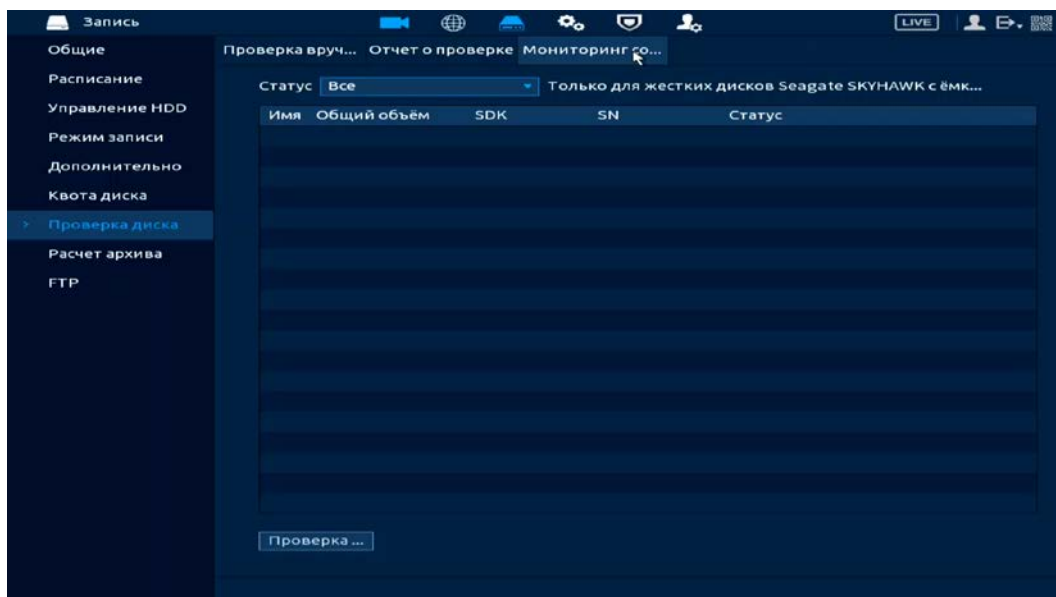
Рисунок 14.24 – Мониторинг состояния
