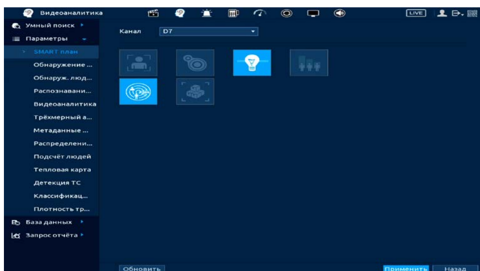
Рисунок 20.9 – Выбор функции
