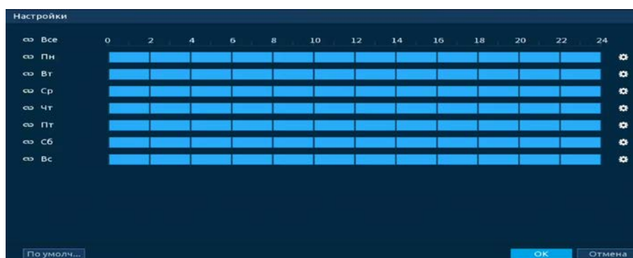
Рисунок 20.14 – Расписание
