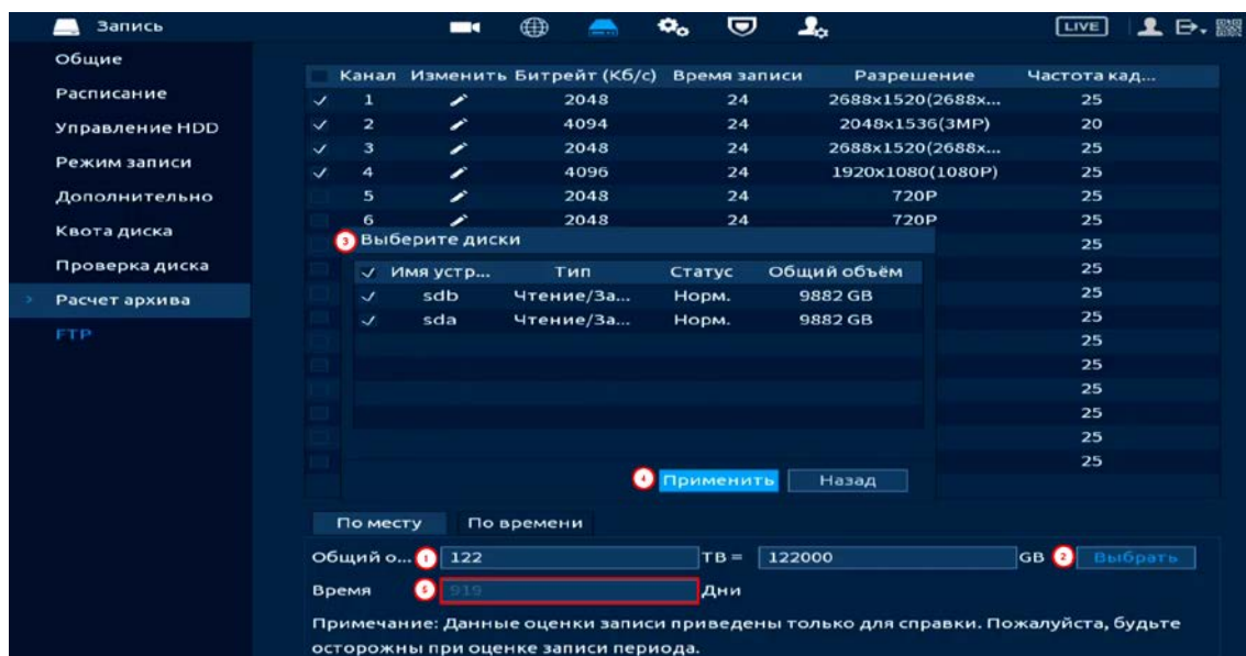
Рисунок 14.26 – Настройка
