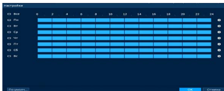
Рисунок 20.52 – Расписание
