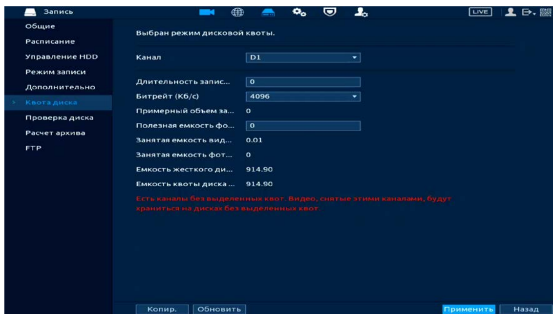
Рисунок 14.21 – Квота диска
