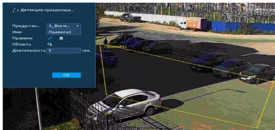
Рисунок 20.68 – Настройка правила
