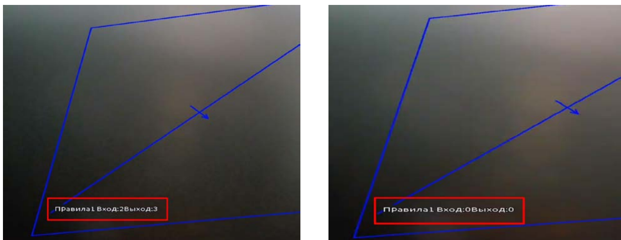
Рисунок 20.86 – Сброс
