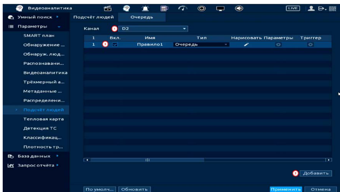
Рисунок 20.99 – Настройка
