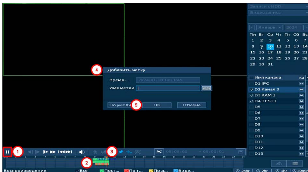
Рисунок 18.11 – Создание метки
