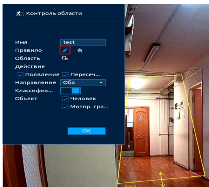
Рисунок 20.30 – Настройка
