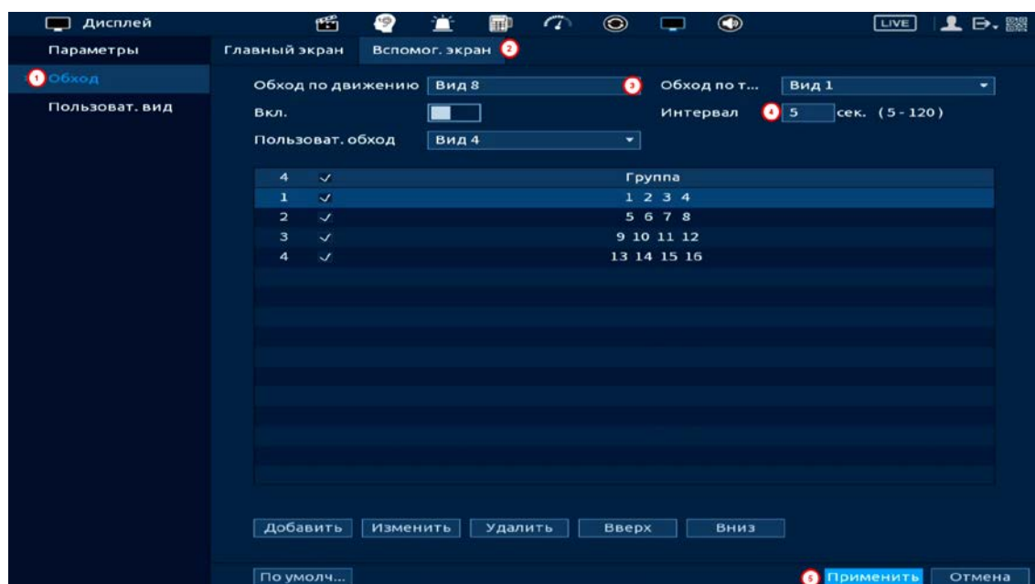
Рисунок 10.7 – Пример настройки
