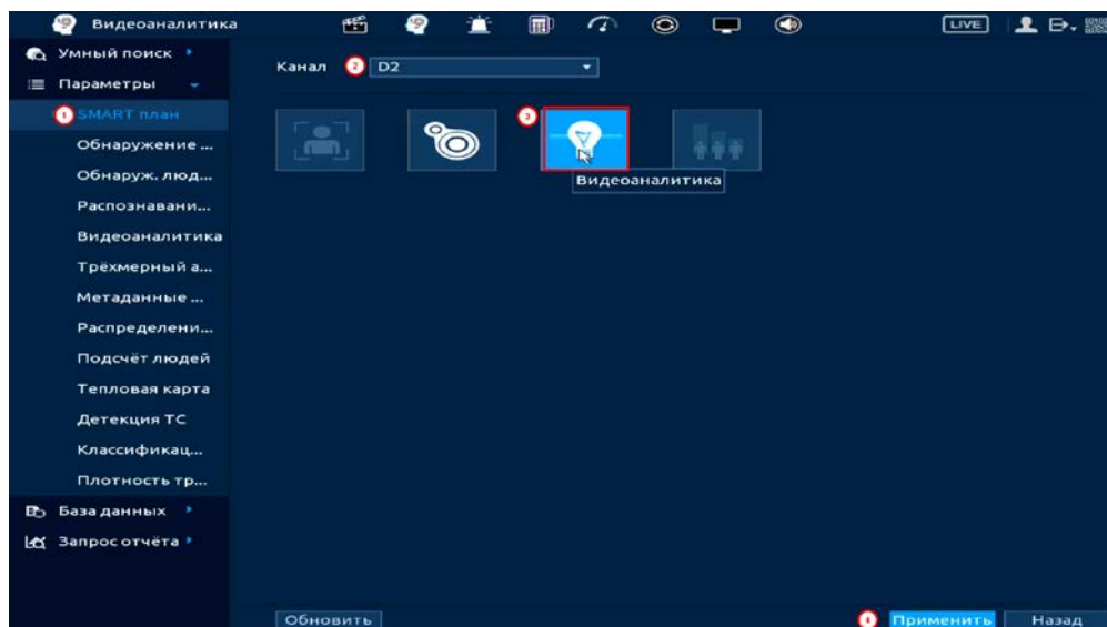
Рисунок 20.48 – Настройка
