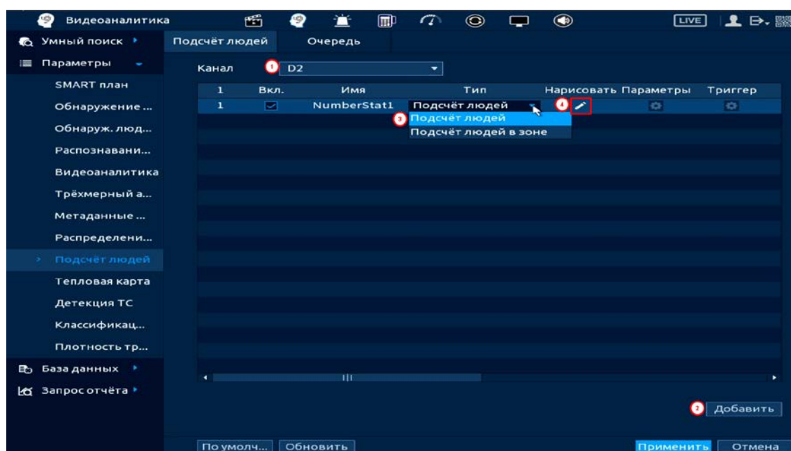
Рисунок 20.81 – Настройка
