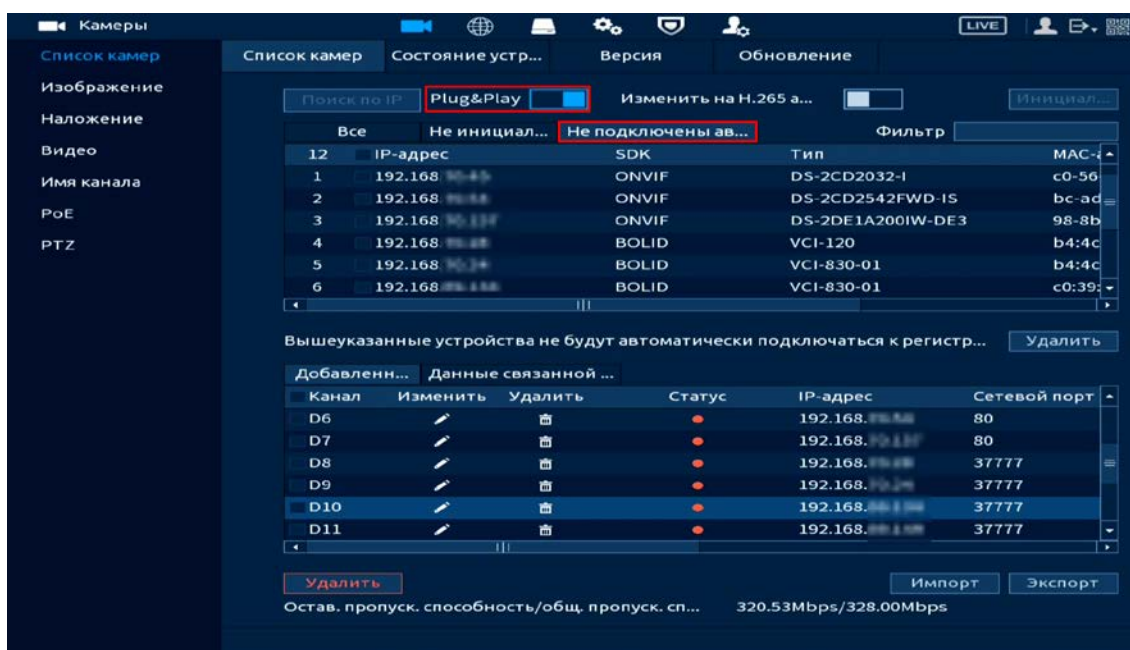
Рисунок 12.6 – Plug&Play
