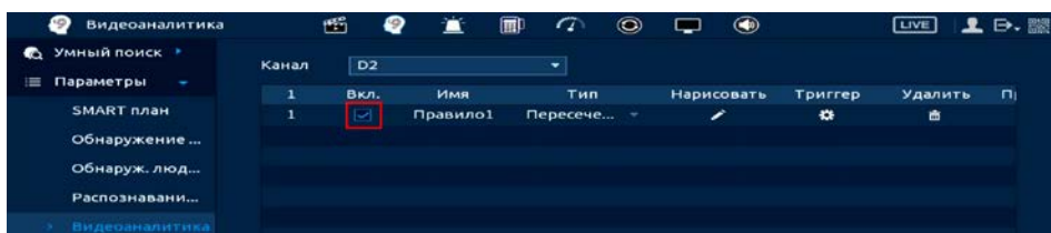
Рисунок 20.24 – Настройка
