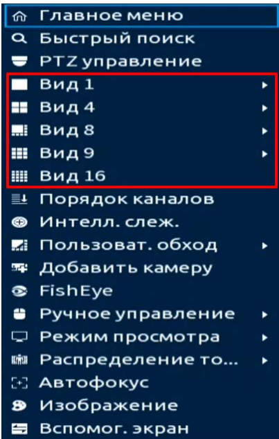
Рисунок 8.1 – Контекстное меню
