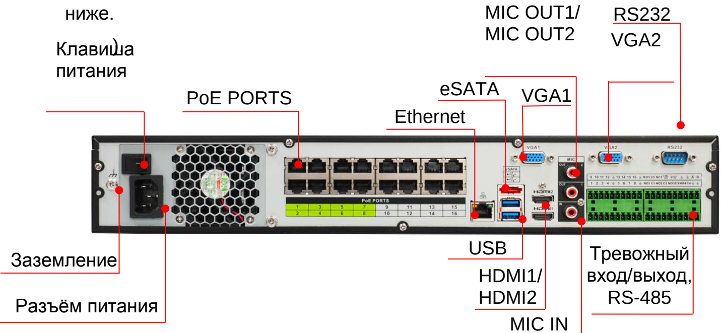
Рисунок 3.2 – Внешний вид задней панели
