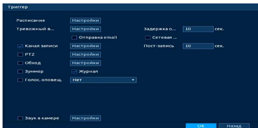
Рисунок 20.39 – Настройка
