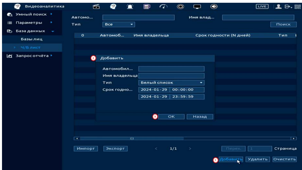
Рисунок 20.8 – Ч/Б список
