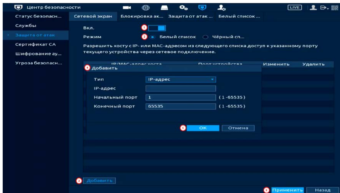
Рисунок 16.8 – Добавить
