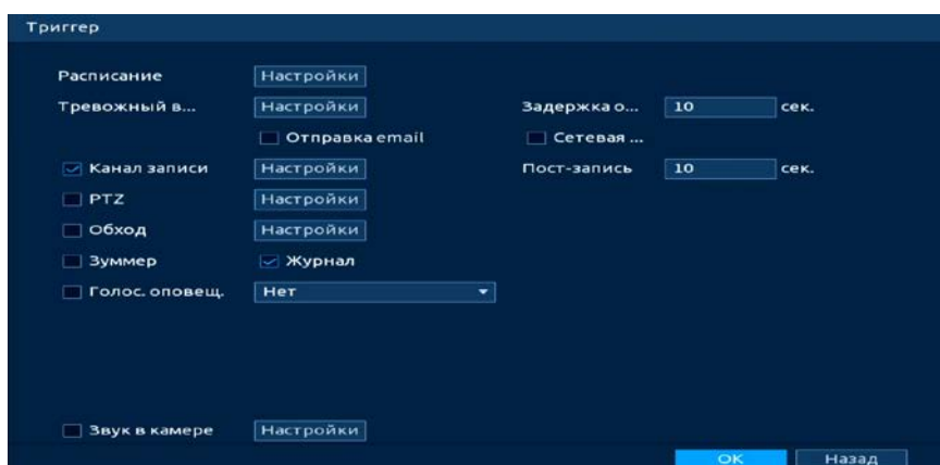
Рисунок 20.51 – Настройка
