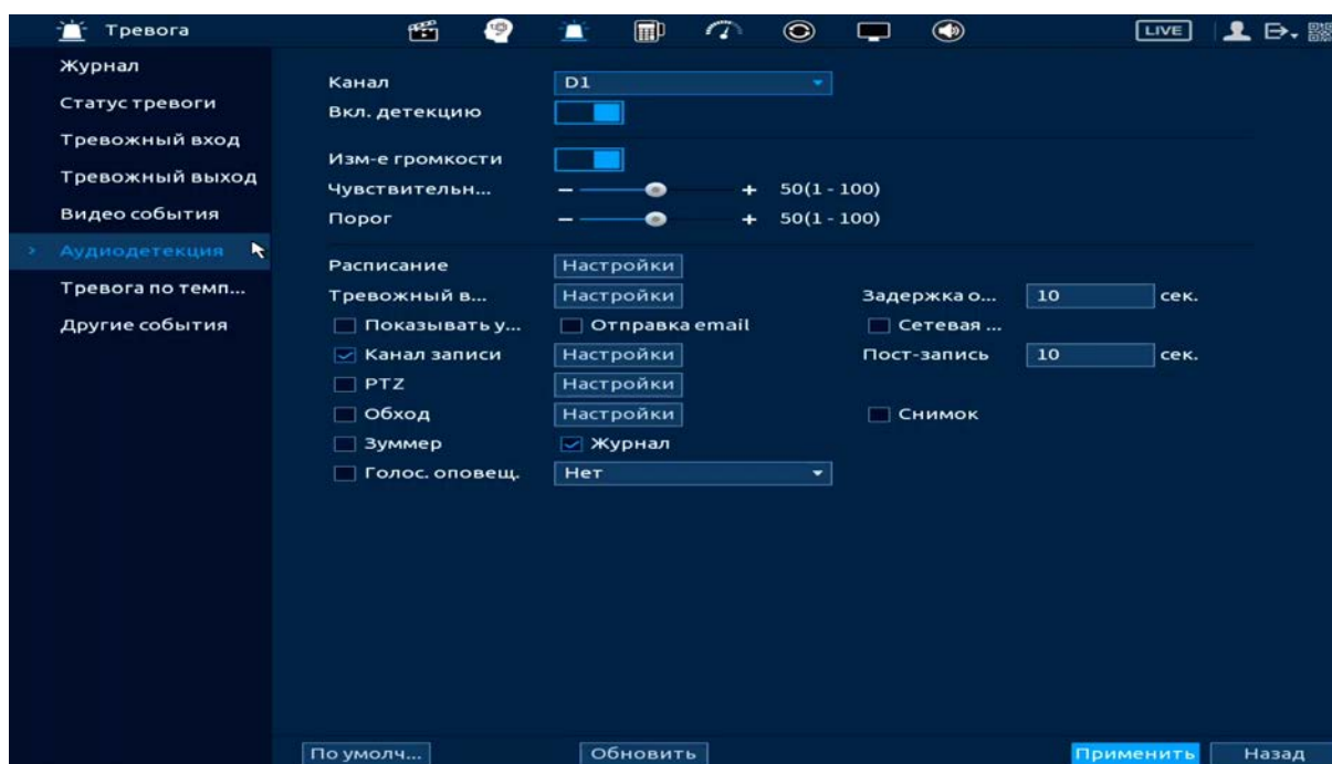
Рисунок 19.38 – Настройка аудиодетекции
