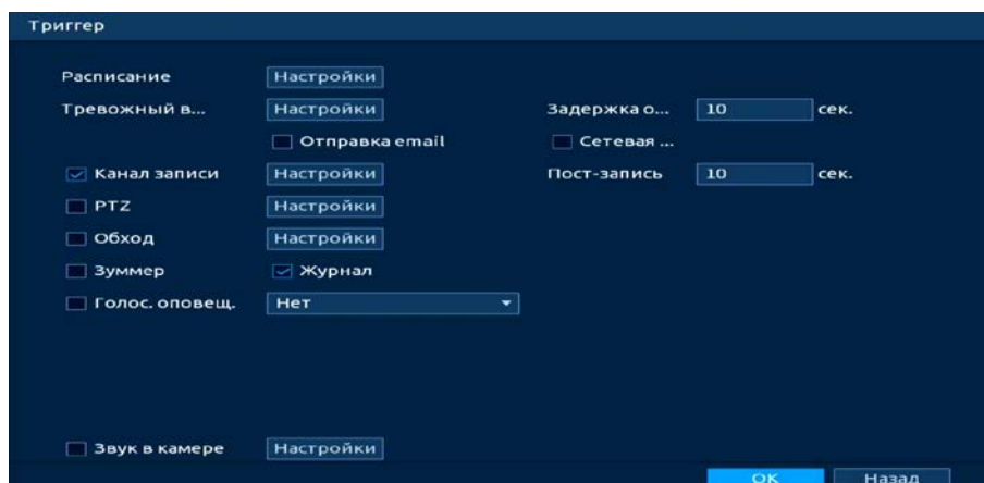
Рисунок 20.63 – Настройка
