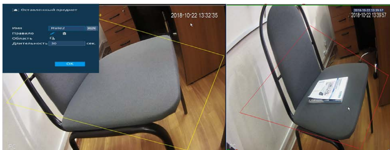
Рисунок 20.38 – Настройка функции
