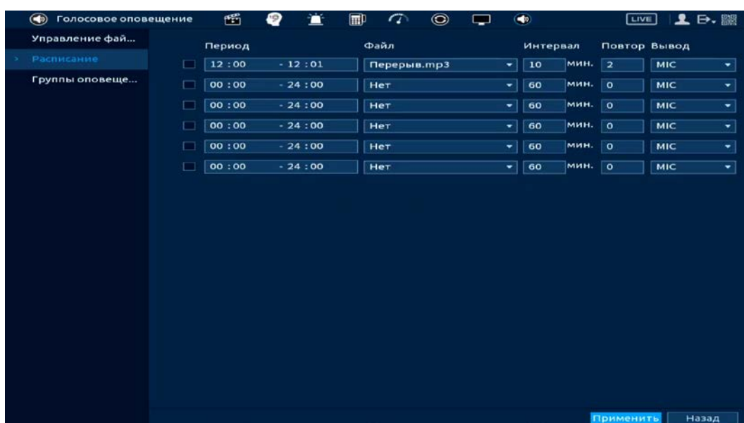
Рисунок 25.6 – Расписание
