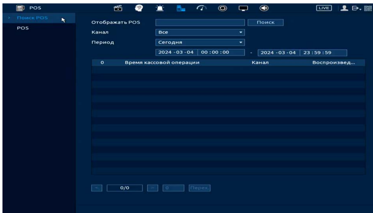
Рисунок 22.1 – POS поиск
