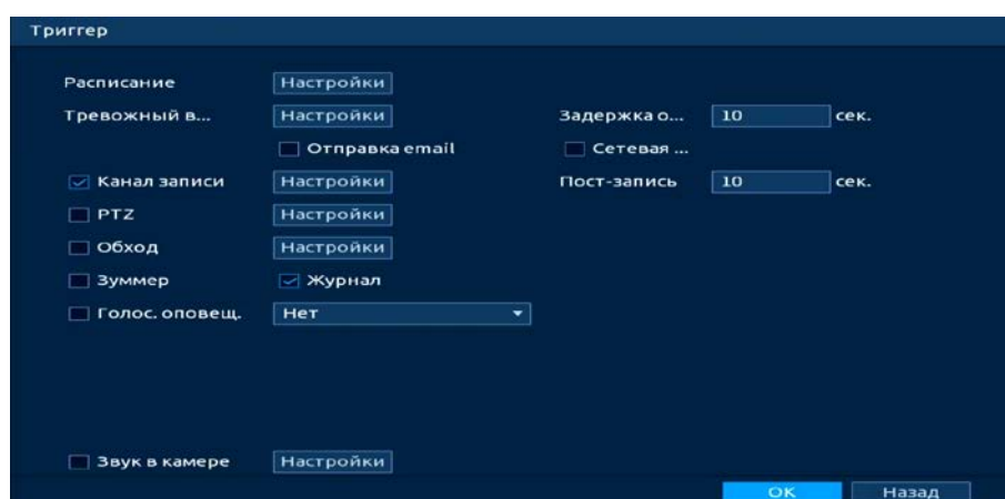
Рисунок 20.45 – Настройка
