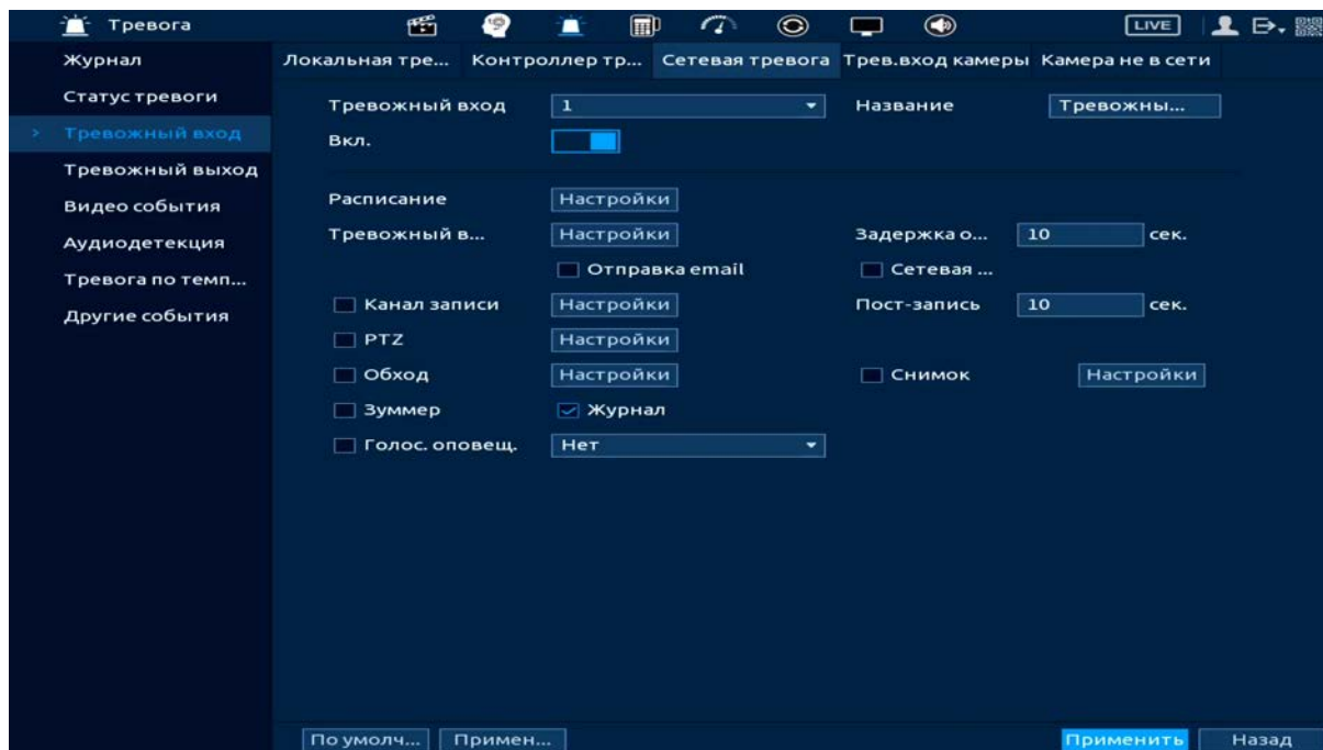
Рисунок 19.7 – Интерфейс настройки
