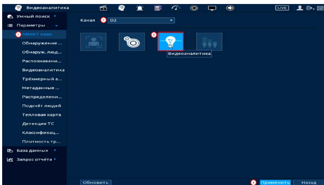
Рисунок 20.36 – Настройка
