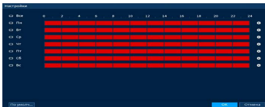
Рисунок 19.8 – Панель расписания
