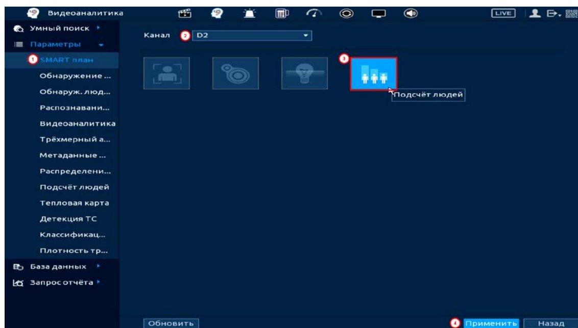
Рисунок 20.80 – Настройка
