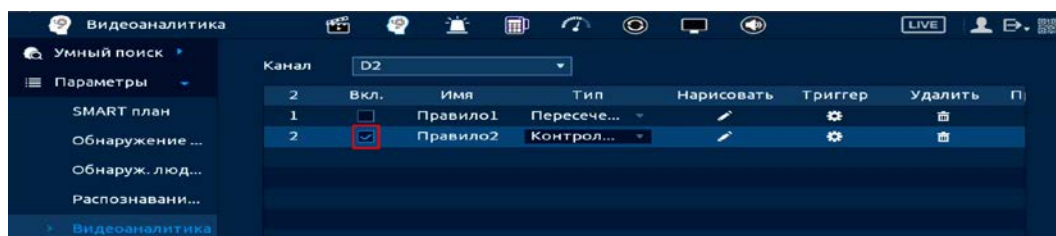
Рисунок 20.32 – Настройка
