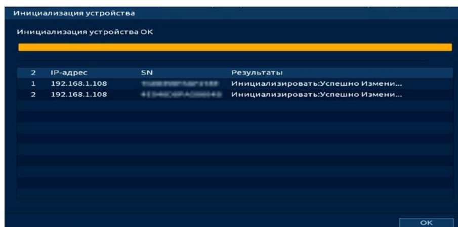
Рисунок 12.15 – Инициализация
