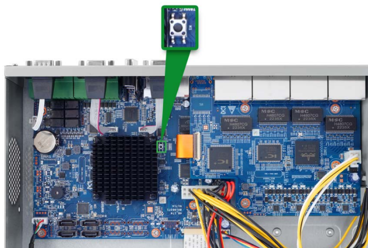
Рисунок 26.8 – Кнопка сброса
