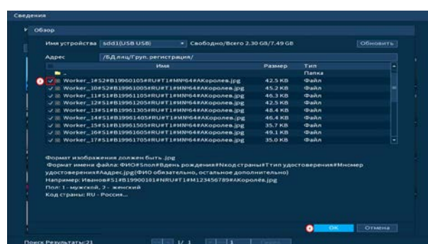
Рисунок 15.6 – Регистрация
