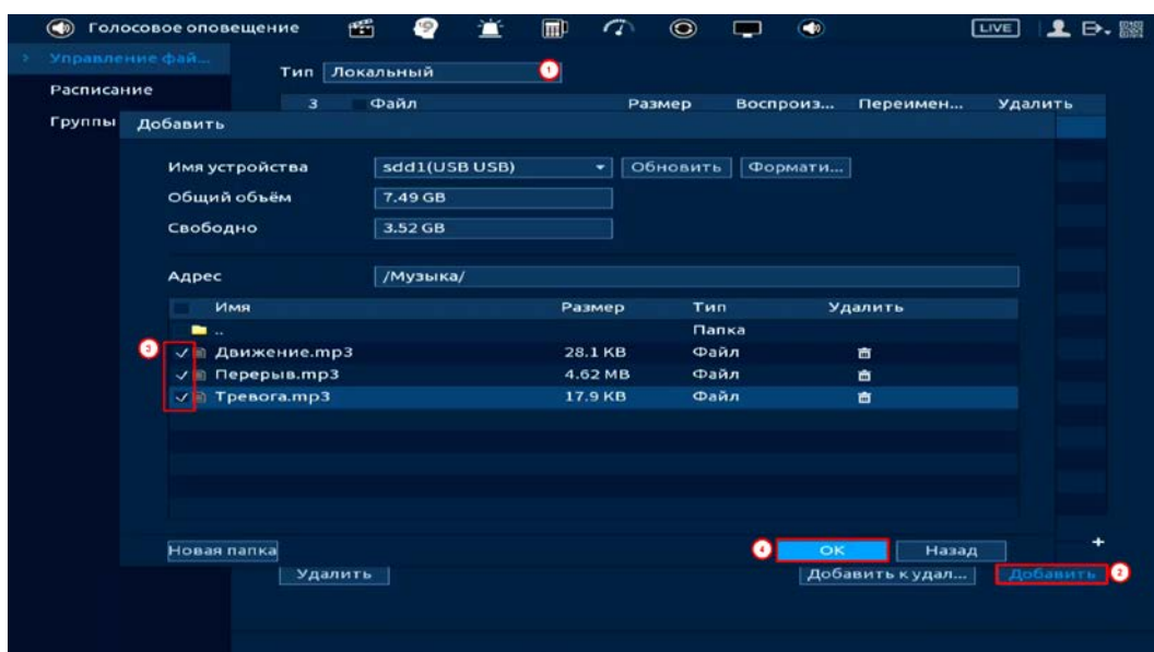
Рисунок 25.2 – Добавление
