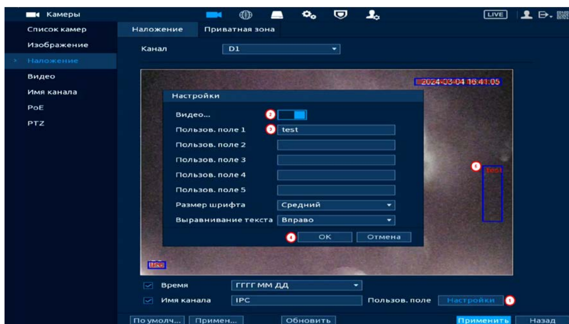
Рисунок 12.35 – Текстовое наложение
