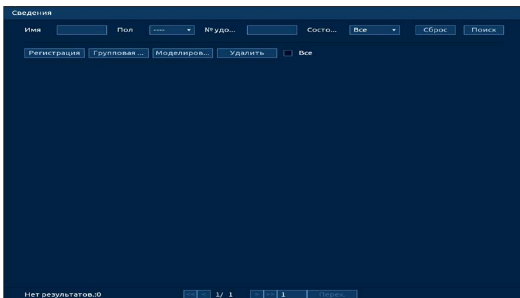
Рисунок 20.3 – Настройка
