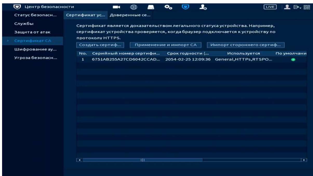
Рисунок 16.15 – Сертификат устройства
