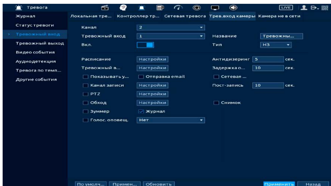
Рисунок 19.11 – Интерфейс настройки
