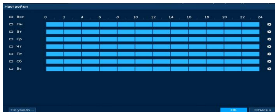
Рисунок 20.78 – Расписание
