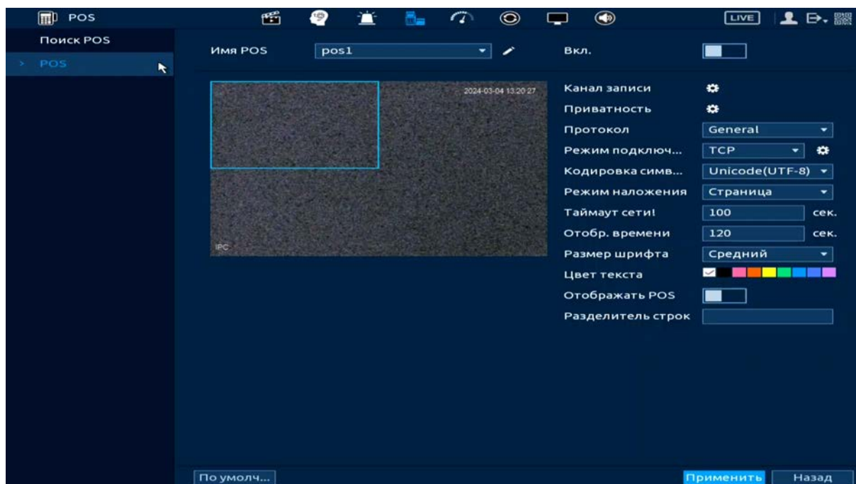
Рисунок 22.2 – POS функция
