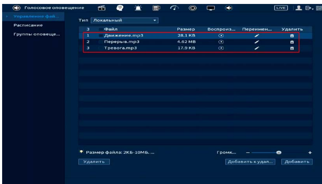
Рисунок 25.3 – Добавление
