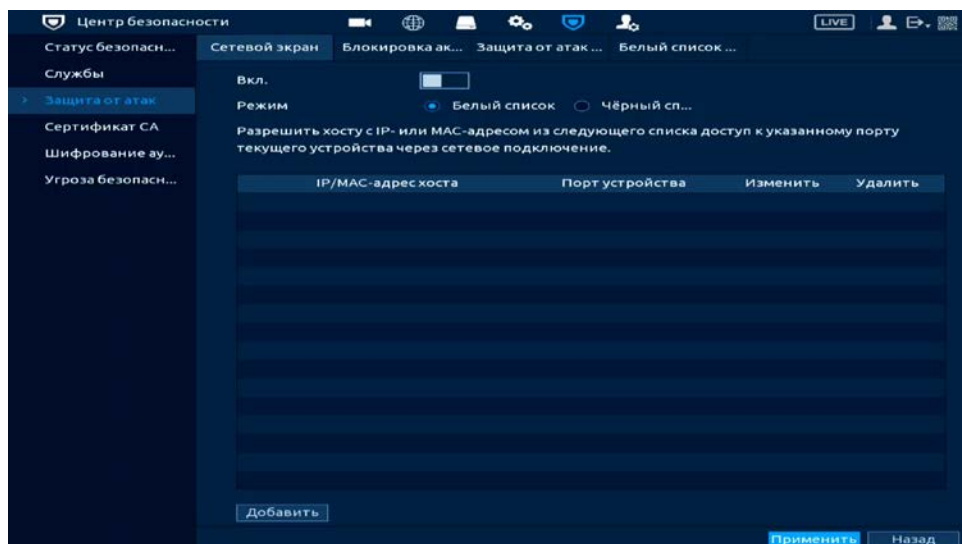
Рисунок 16.7 – Сетевой экран
