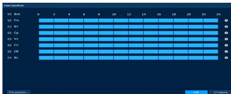
Рисунок 20.70 – Расписание
