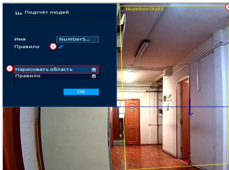
Рисунок 20.83 – Нарисовать область
