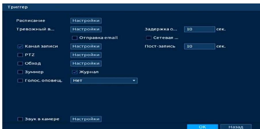
Рисунок 20.87 – Настройка
