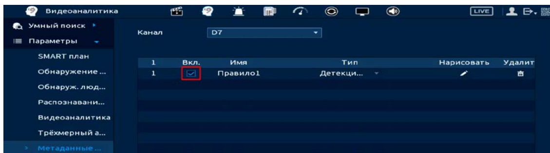
Рисунок 20.76 – Настройка
