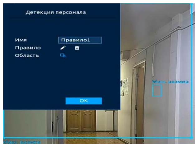
Рисунок 20.75 – Настройка
