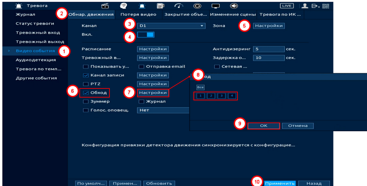
Рисунок 10.8 – Пример настройки
