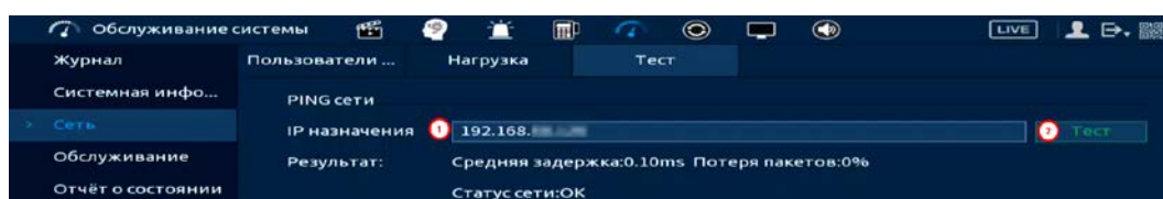
Рисунок 21.9 – Проверка IP-адреса
