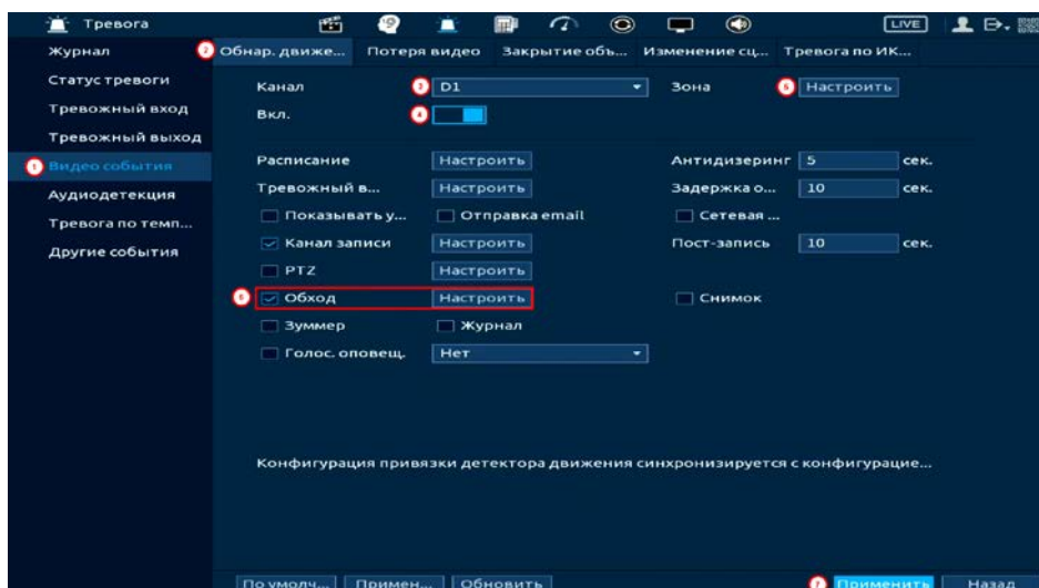
Рисунок 24.5 – Пример настройки
