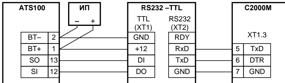
Рисунок 2. Подключение радиопередатчика ATС100
