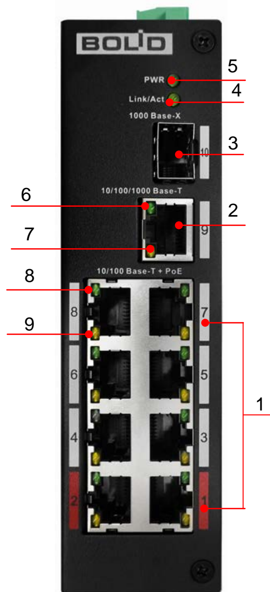
Рисунок 5.2 – Передняя панель
