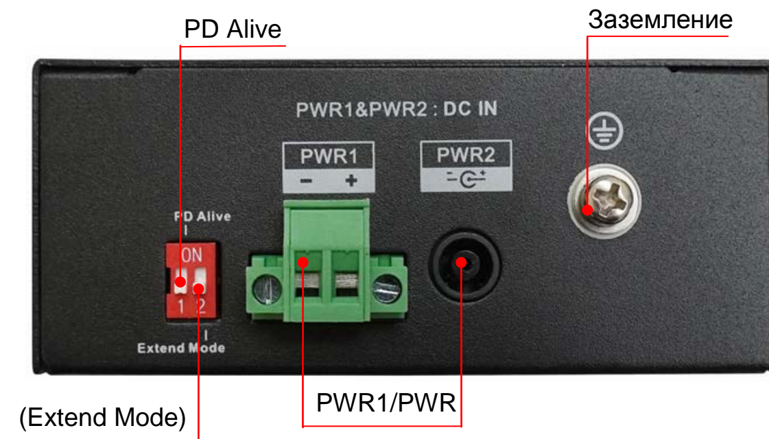
Рисунок 5.1 – Верхняя панель
