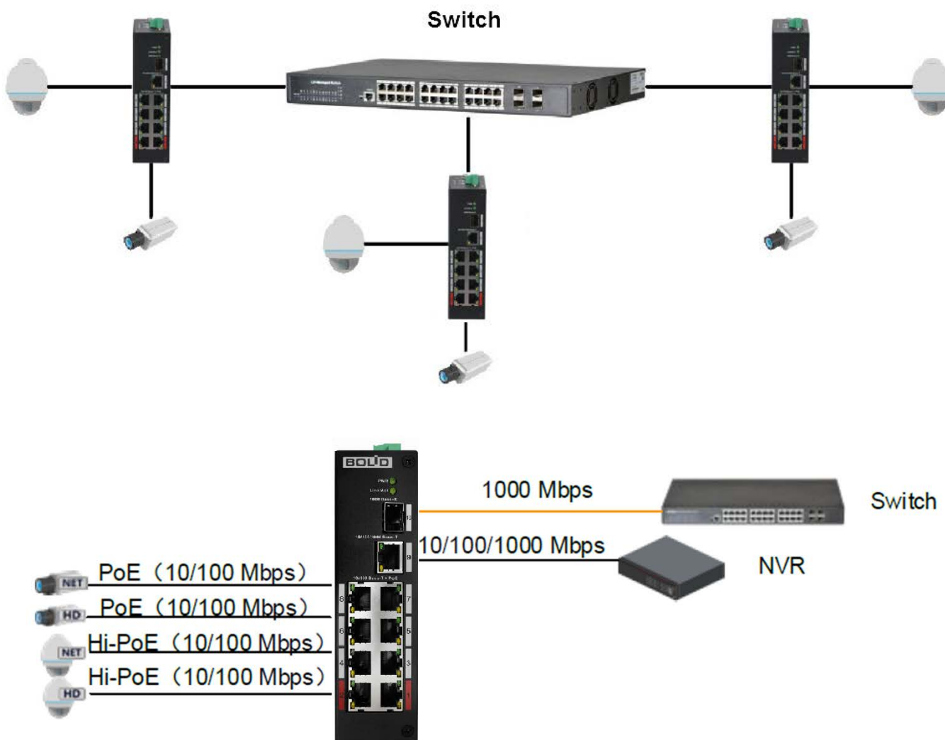
Рисунок 1.1 – Сетевое соединение
