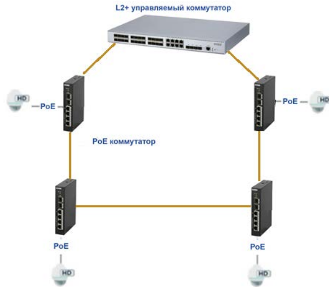
Рисунок 1.2 – Кольцевое соединение
