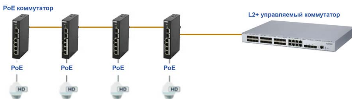
Рисунок 1.1 – Каскадное соединение
