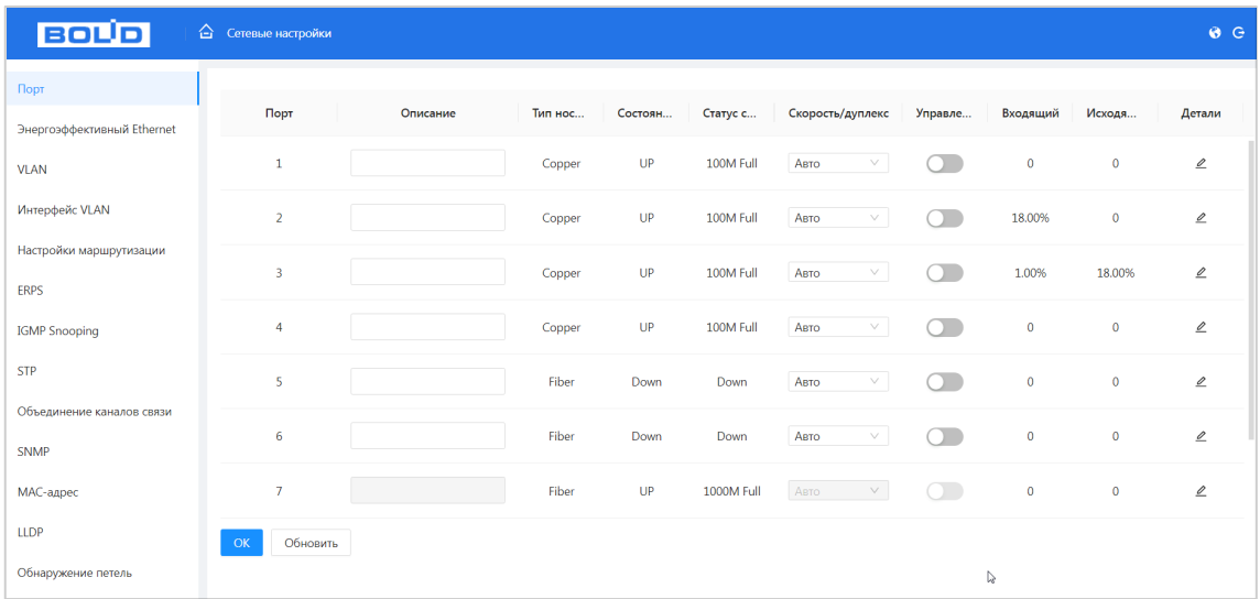
Рисунок 10.1 – Настройка портов
