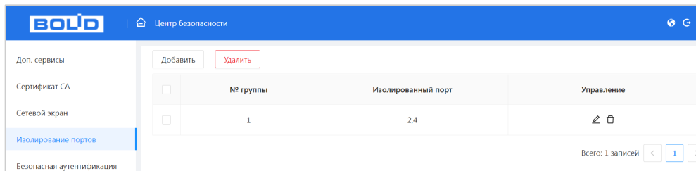
Рисунок 12.15 – Изолирование портов
