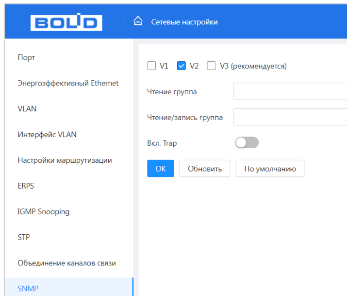
Рисунок 10.20 – Настройки SNMP
