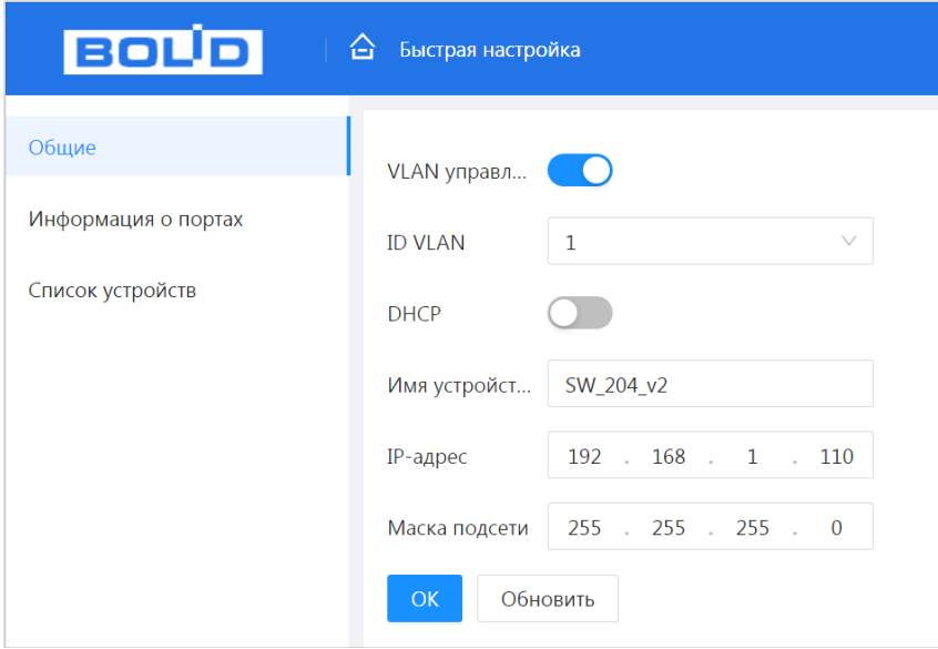
Рисунок 6.5 – Сетевые настройки
