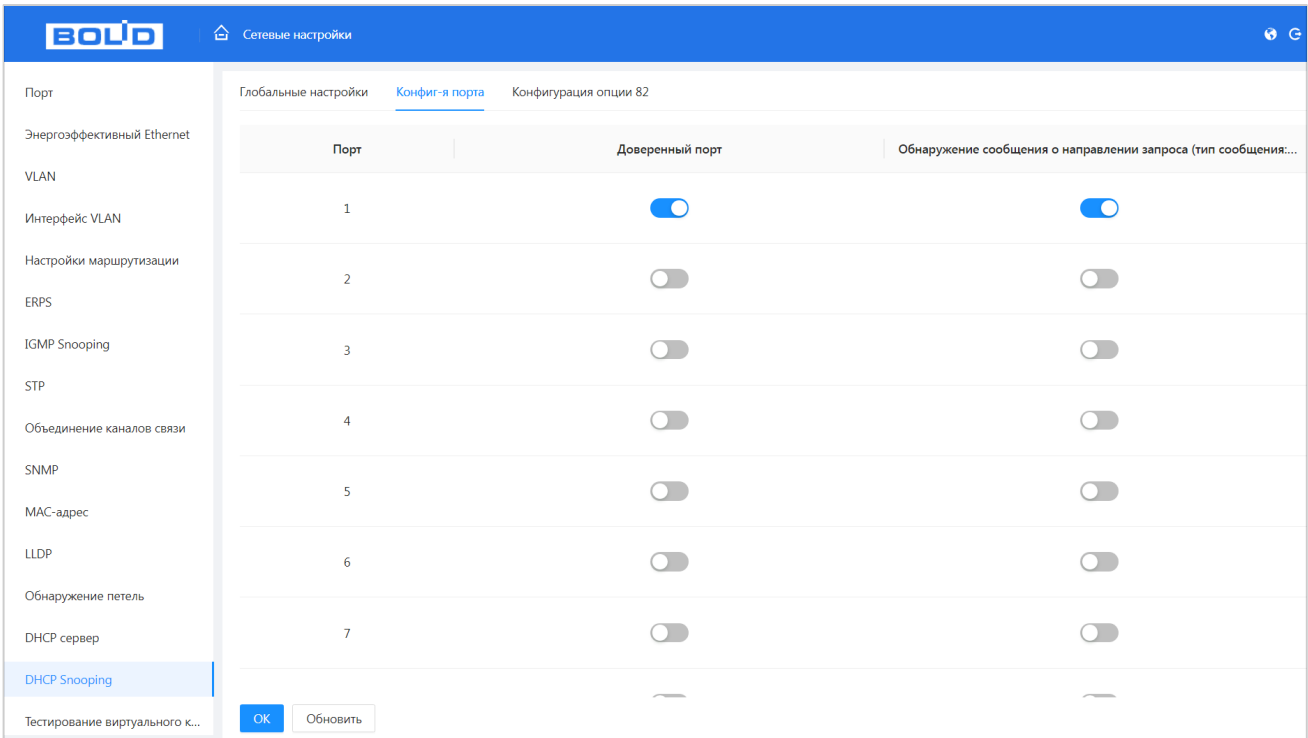
Рисунок 10.33 – Настройка портов
