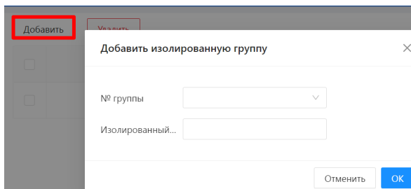
Рисунок 12.16 – Добавление группы
