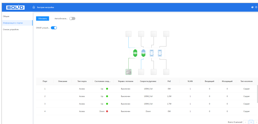
Рисунок 8.2 – Информационная панель
