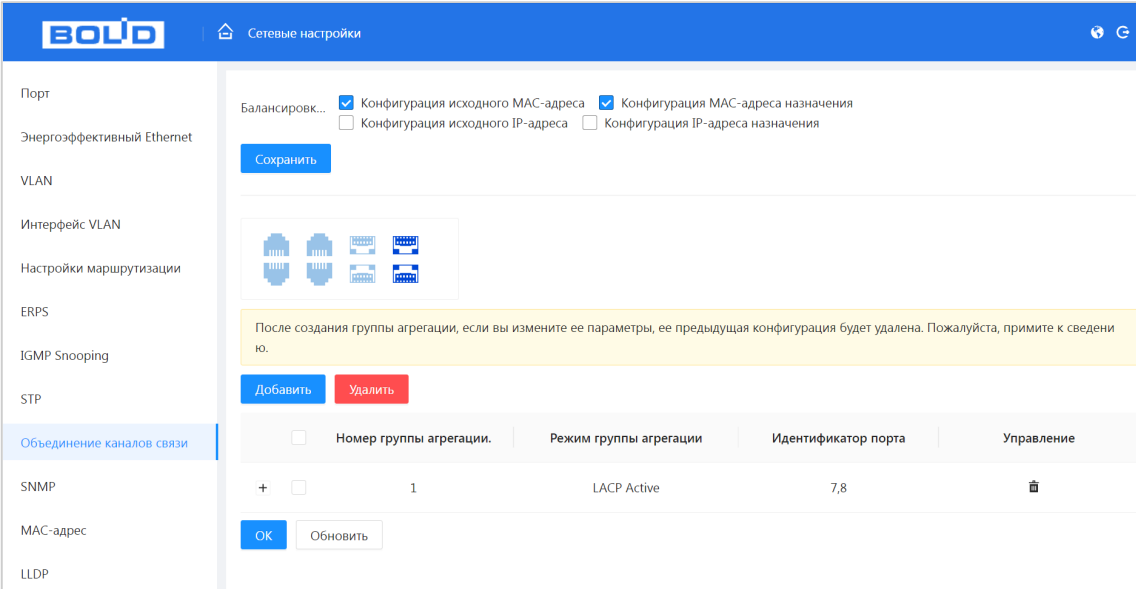
Рисунок 10.17 – Агрегация каналов
