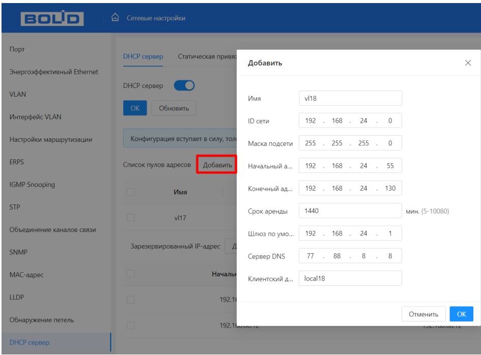
Рисунок 10.27 – Добавить пул
