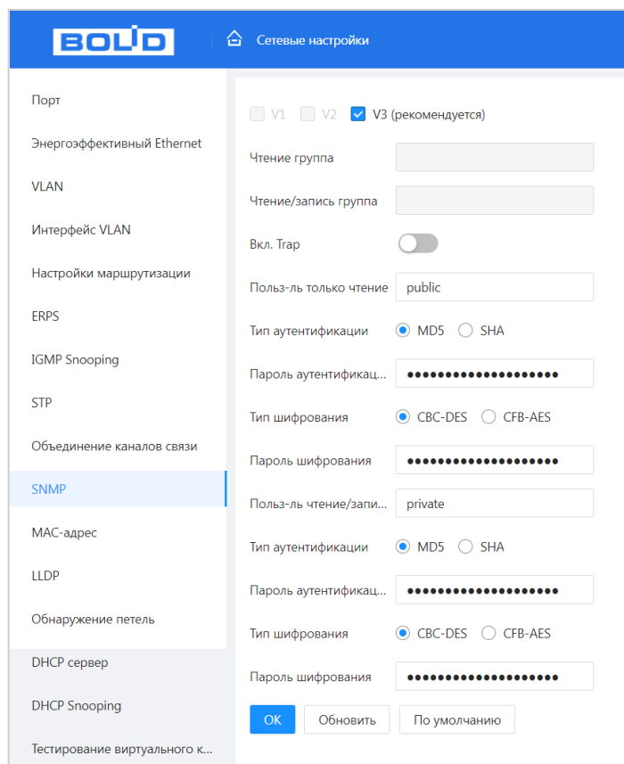
Рисунок 10.21 – Настройки SNMPv3
