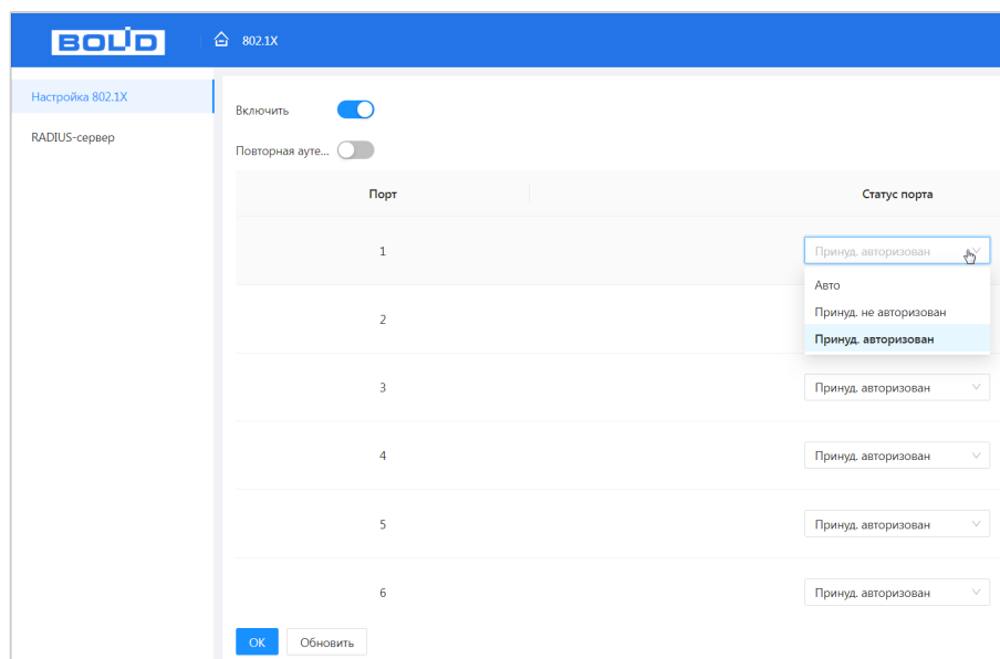
Рисунок 14.1 – Настройки NSA
