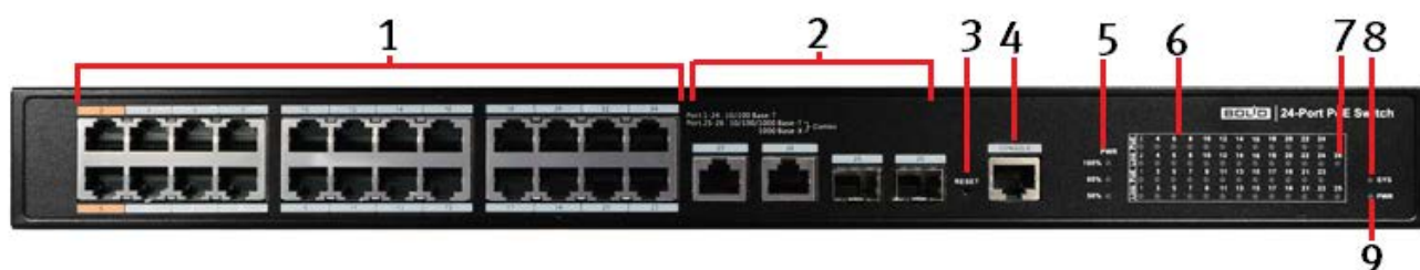
Рисунок 4.1 – Передняя панель конструкции
