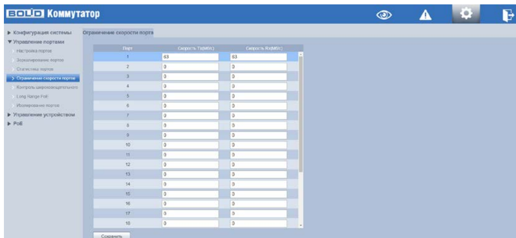
Рисунок 8.15 – Ограничение скорости
