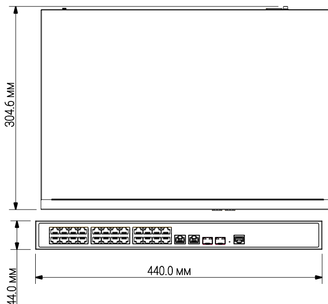
Рисунок 5.1 – Габаритные размеры
