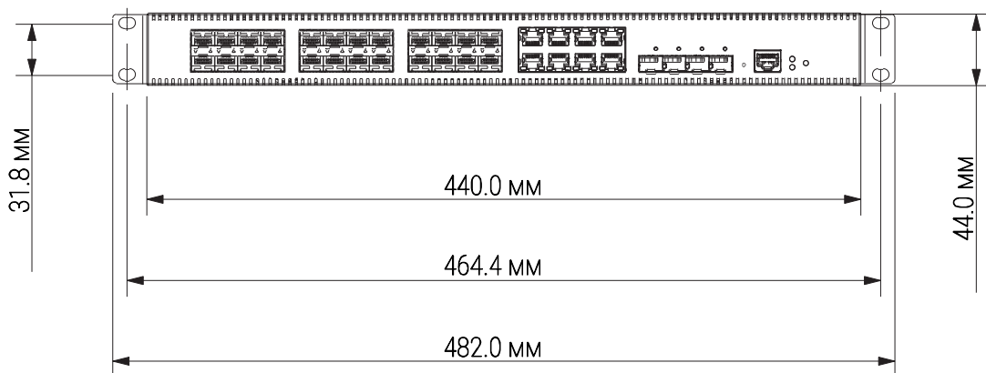
Рисунок 5.2 – Габаритные размеры
