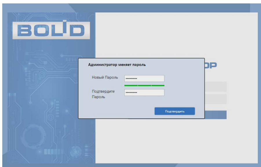
Рисунок 6.2 – Установка пароля
