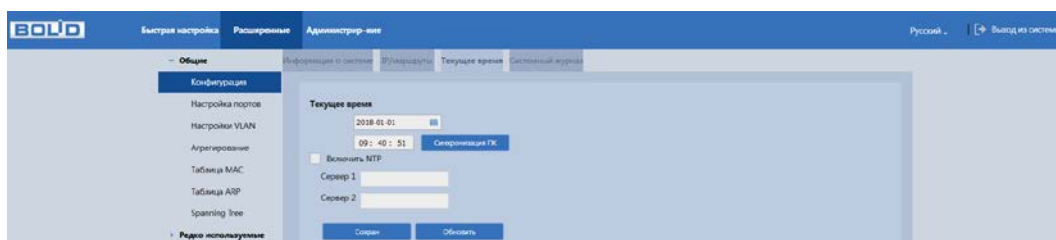
Рисунок 8.2 – Настройка/синхронизация времени
