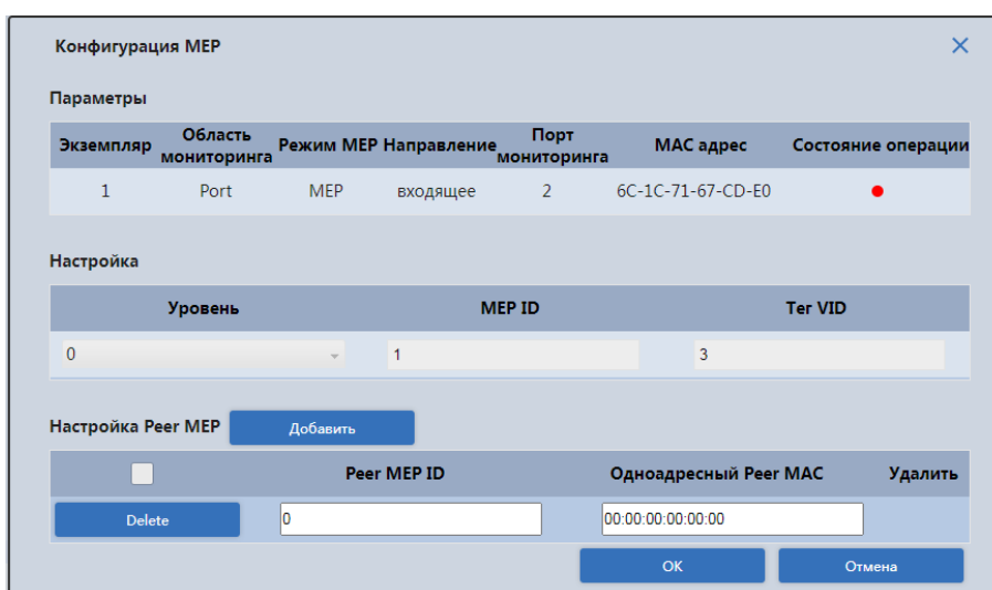
Рисунок 11.6 – Конфигурация MEP
