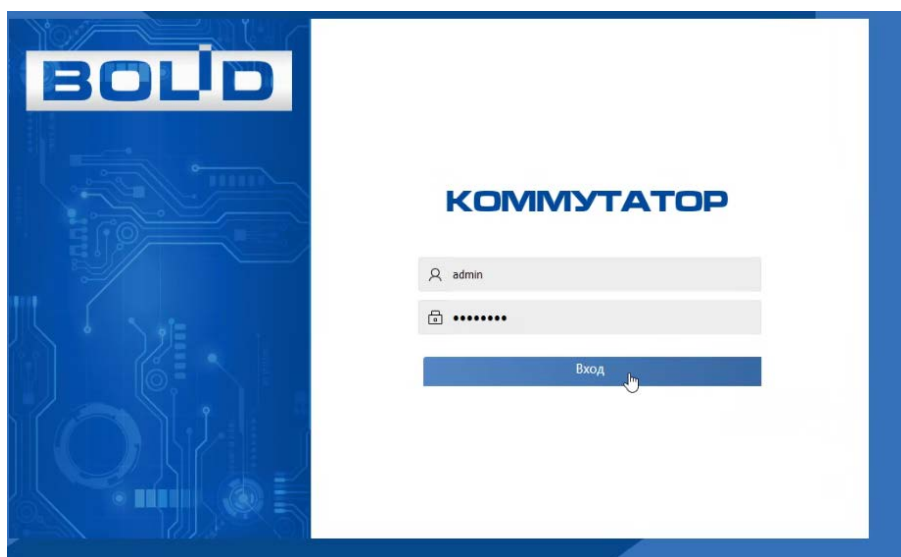
Рисунок 6.3 – Вход
