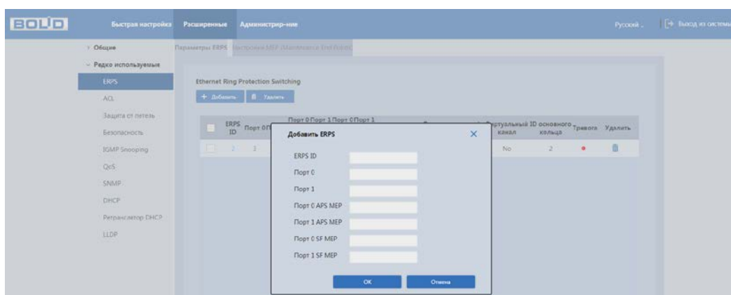
Рисунок 11.7 – Добавление ERPS
