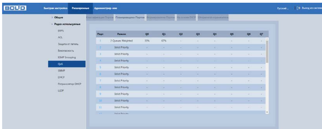
Рисунок 9.17 – Планировщик портов
