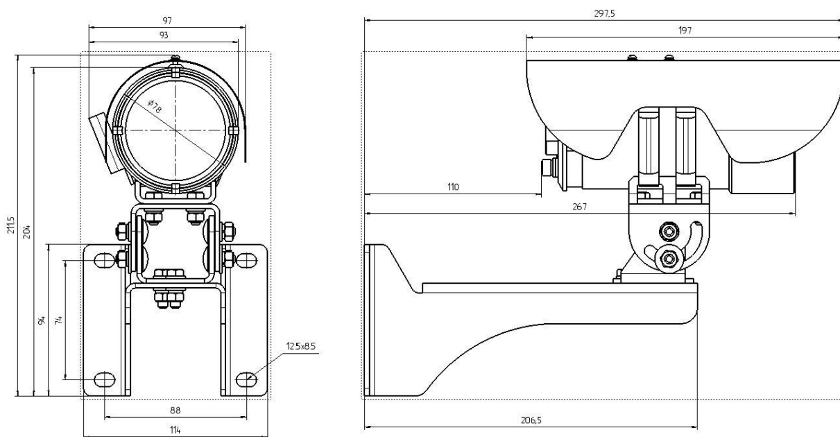
Рисунок 4.2 – Габаритные размеры термокожуха (мм)
