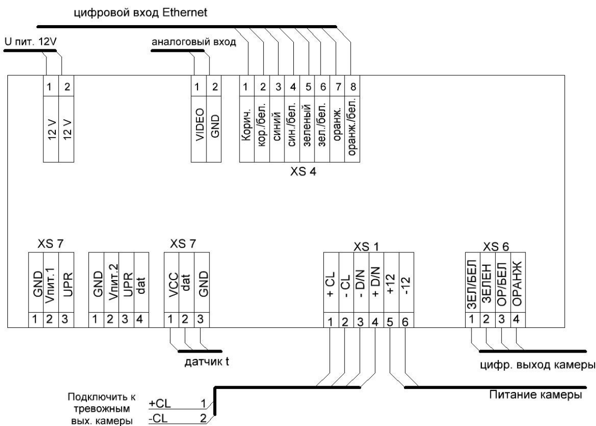
Рисунок 4.5 – Схема подключения термокожуха с напряжением 12 В постоянного тока
