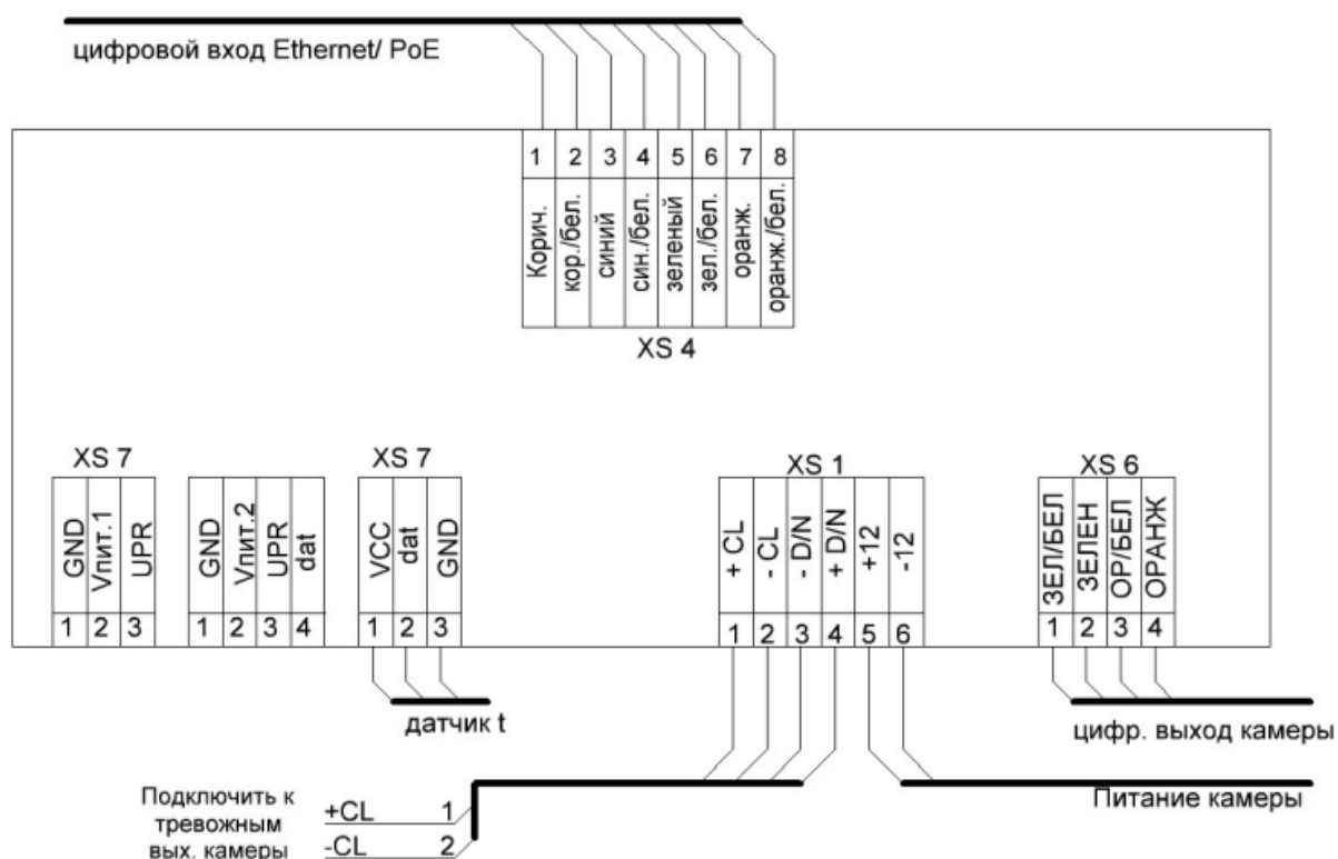
Рисунок 4.3 – Схема подключения термокожуха с напряжением питания по PoE
