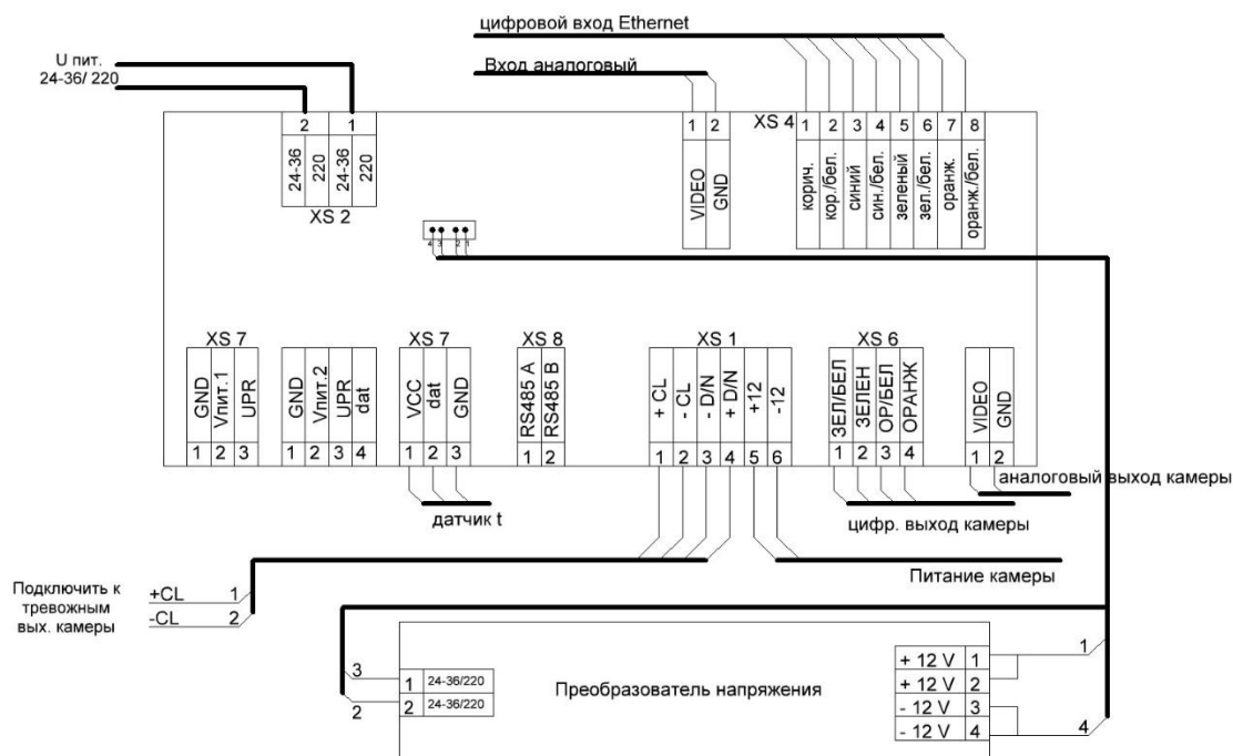
Рисунок 4.4 – Схема подключения термокожуха с напряжением питания 24–36 постоянного/переменного тока или 220 В переменного тока
