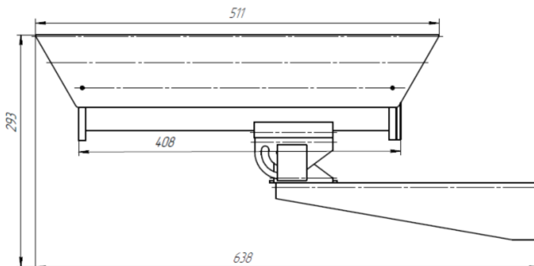
Рисунок 4.2 – Габаритные размеры термокожуха (мм)
