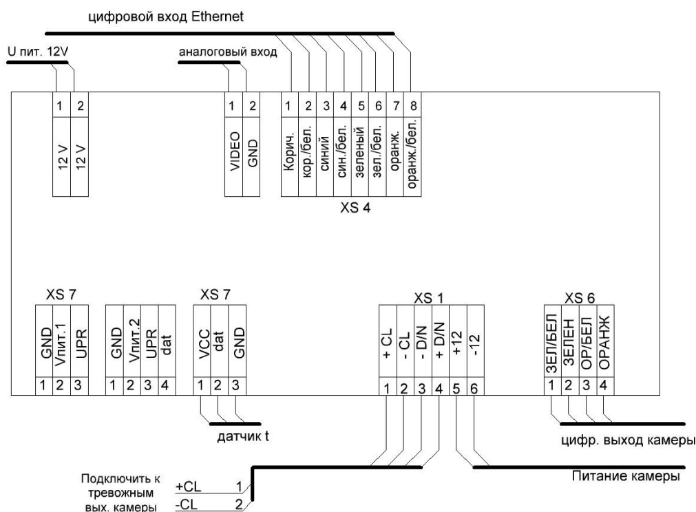
Рисунок 4.4 – Схема подключения термокожуха с напряжением
