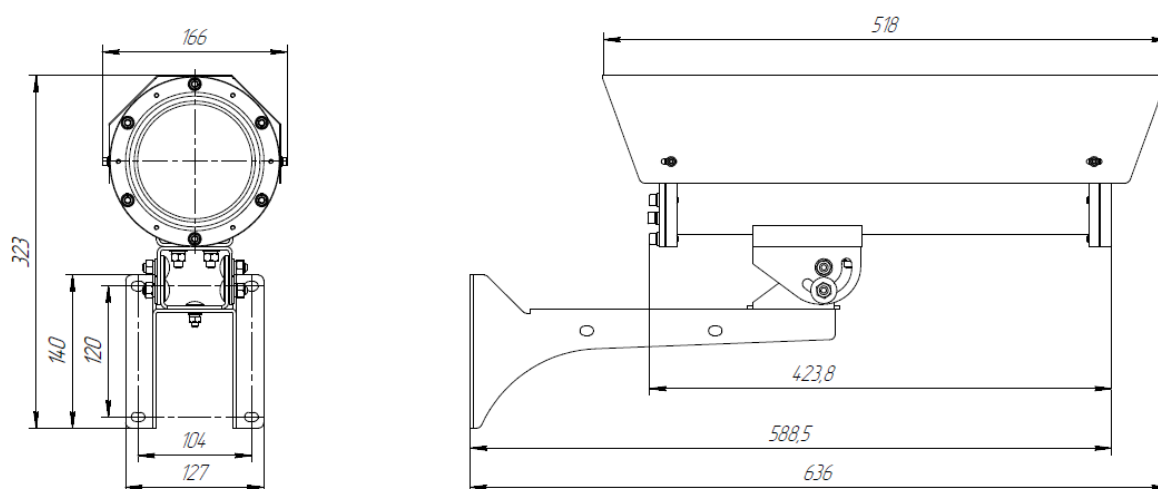
Рисунок 4.2 – Габаритные размеры термокожуха (мм)
