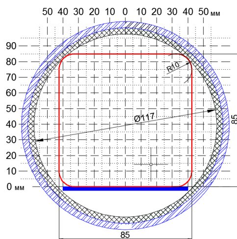
Рисунок 4.4 – Сечение термокожуха
