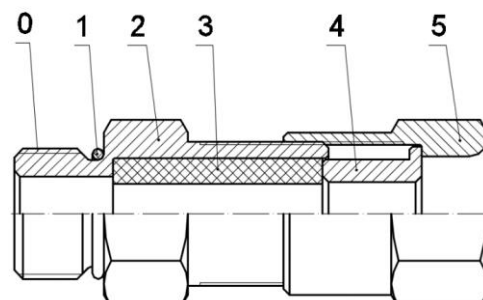
КВН – для монтажа открытого кабеля
