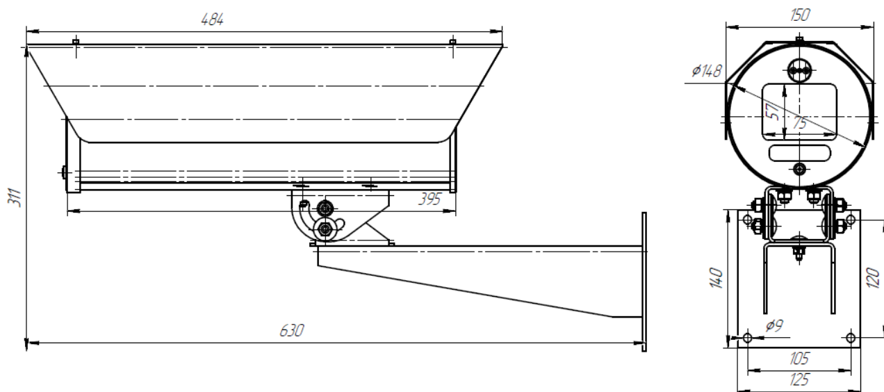
Рисунок 4.2 – Габаритные размеры термокожуха (мм)
