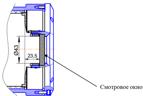
Рисунок 4.3 – Внутреннее пространство смотрового окна
