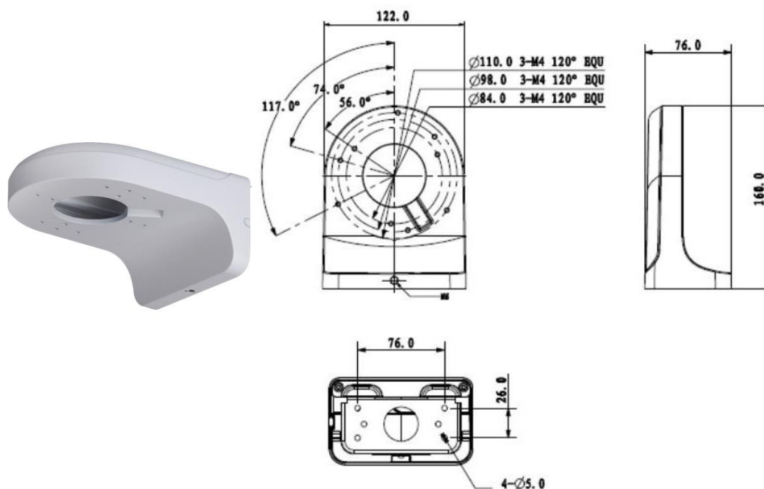
Рисунок 5.4 - Внешний вид и габаритные размеры кронштейна BR-105
