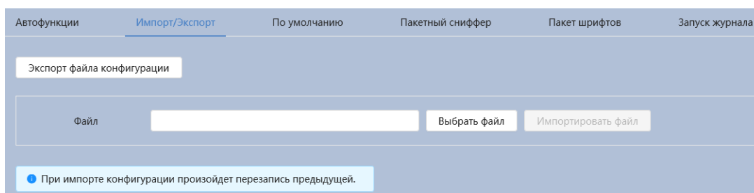
Рисунок 7.117 – Вкладка «Импорт/Экспорт»
