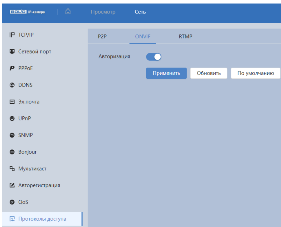
Рисунок 8.20 – Вкладка «ONVIF»
