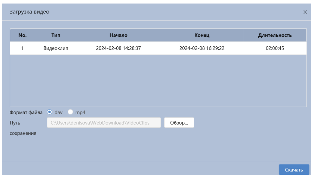
Рисунок 7.126 – Загрузка видео
