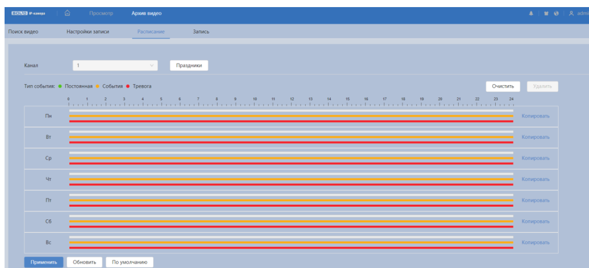
Рисунок 7.128 – Вкладка «Расписание»
