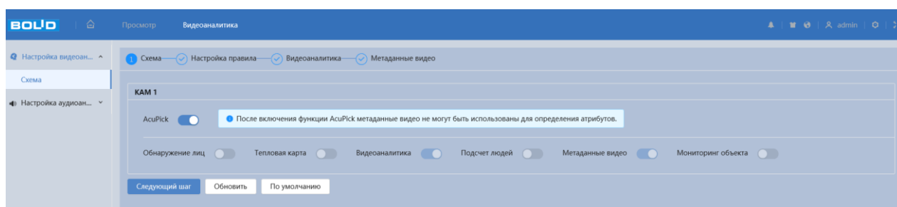
Рисунок 7.23 – Функция «AsuRisk»
