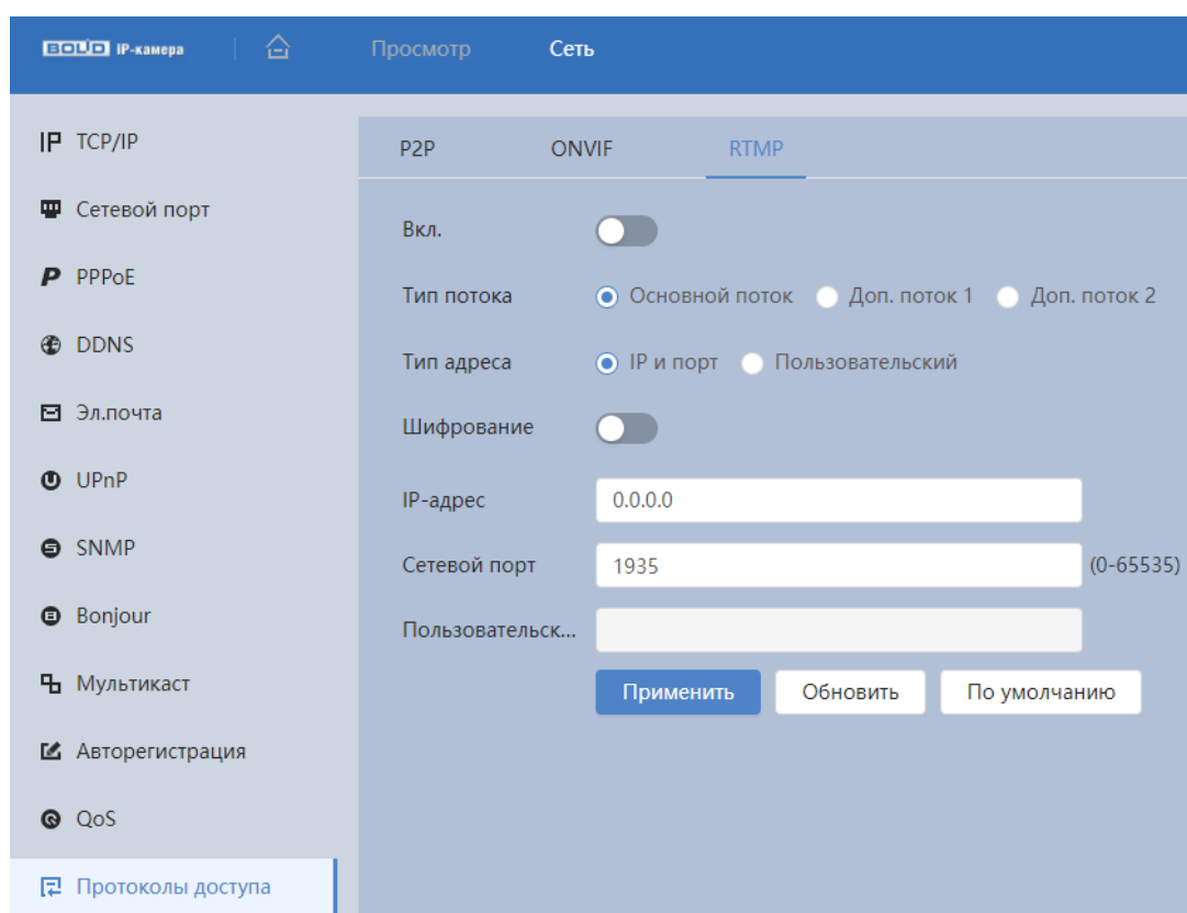
Рисунок 8.21 – Вкладка «RTMP»
