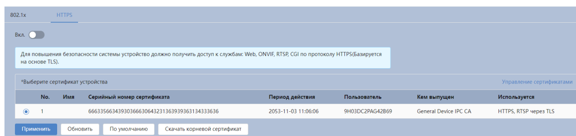
Рисунок 7.144 – Вкладка «HTTPS»
