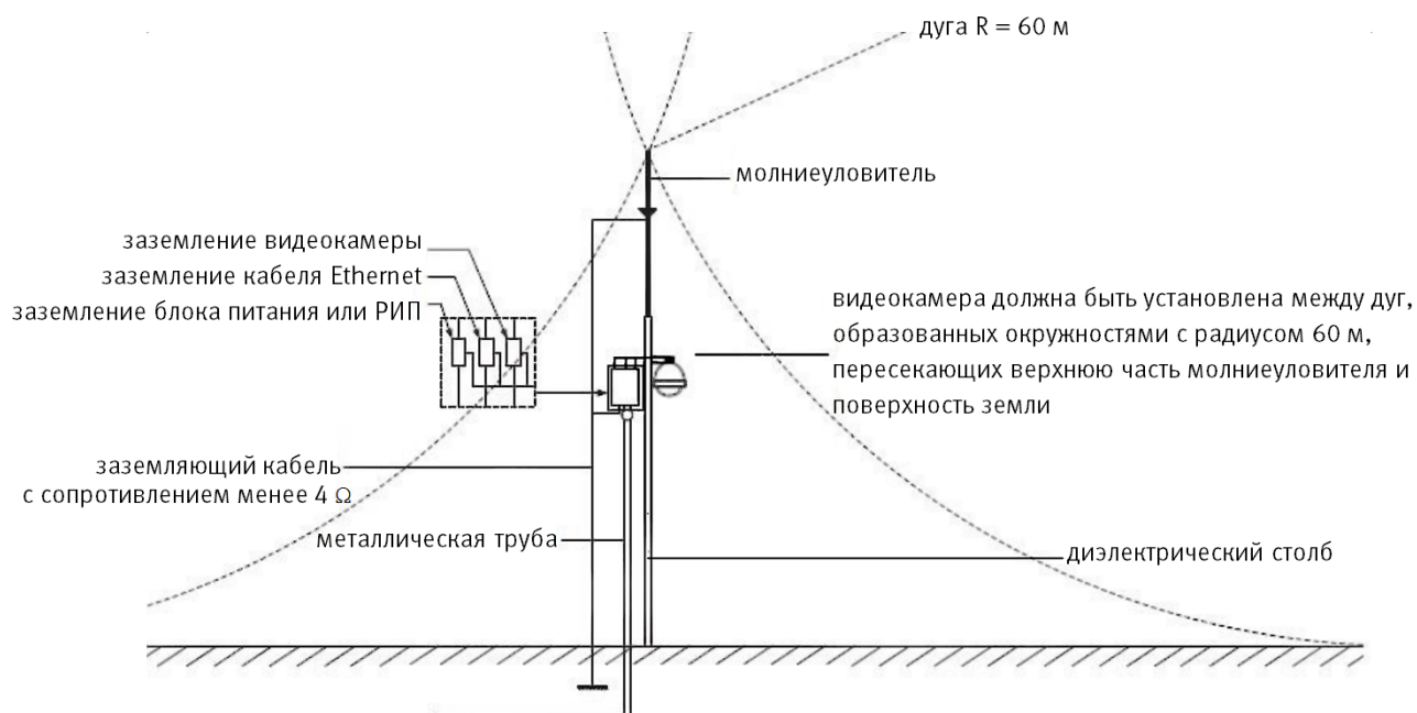
Рисунок 6.14 – Установка молниеотвода
