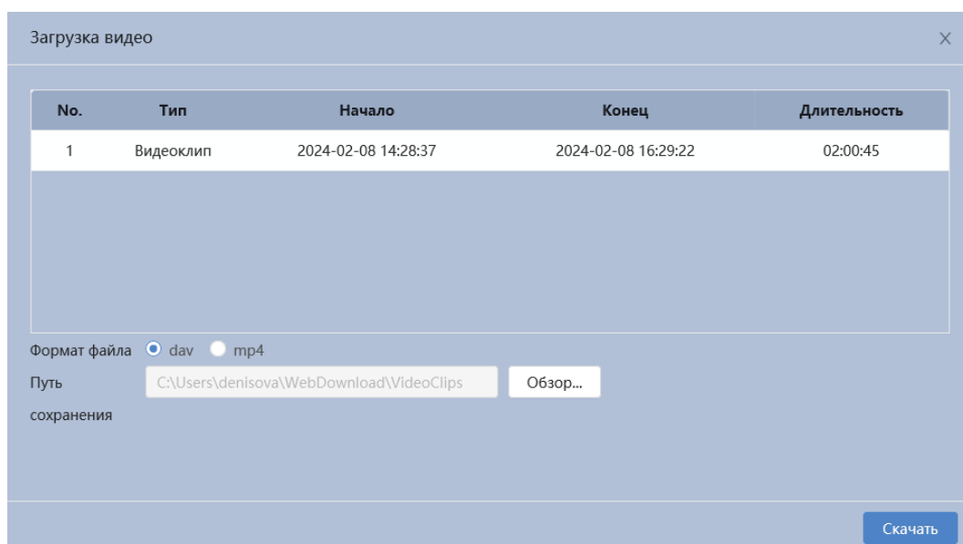
Рисунок 7.121 – Загрузка видео
