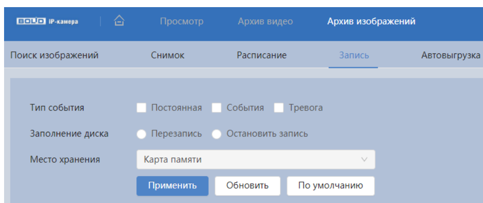
Рисунок 7.131 – Вкладка «Запись»
