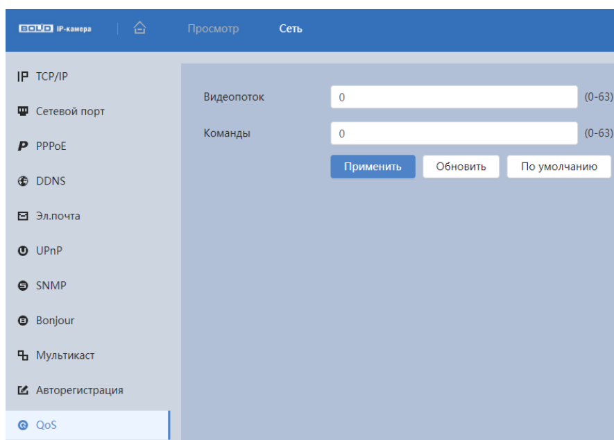
Рисунок 8.17 – Подпункт меню«QoS»
