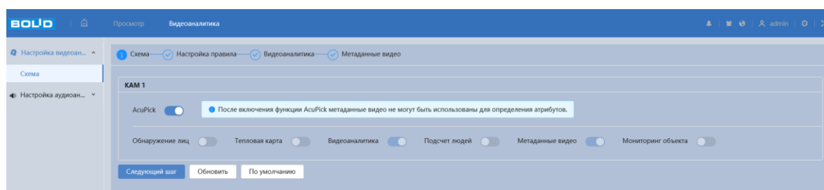
Рисунок 7.23 – Функция «АсиРиск»
