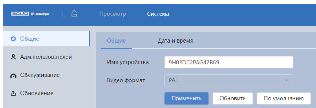
Рисунок 7.102 – Вкладка «Общие»
