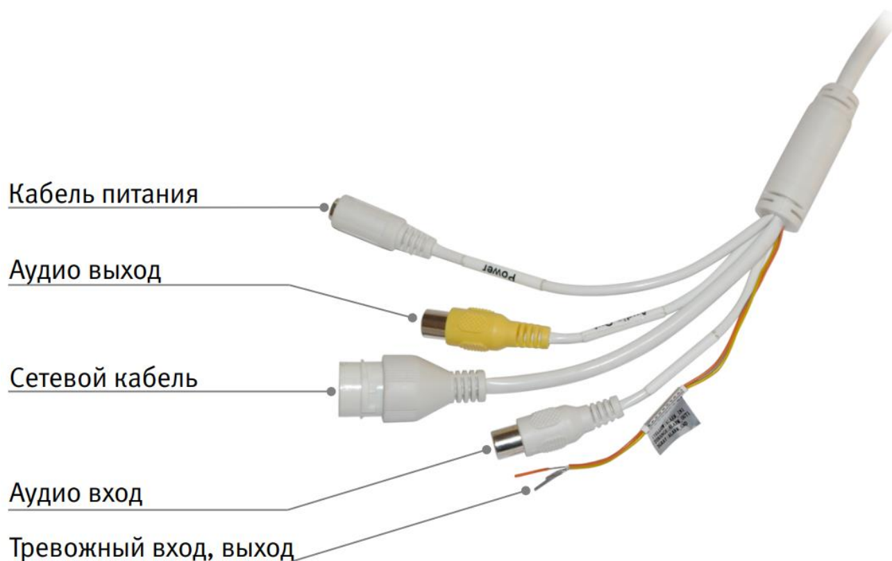
Рисунок 6.1 – Кабель видеокamеры
