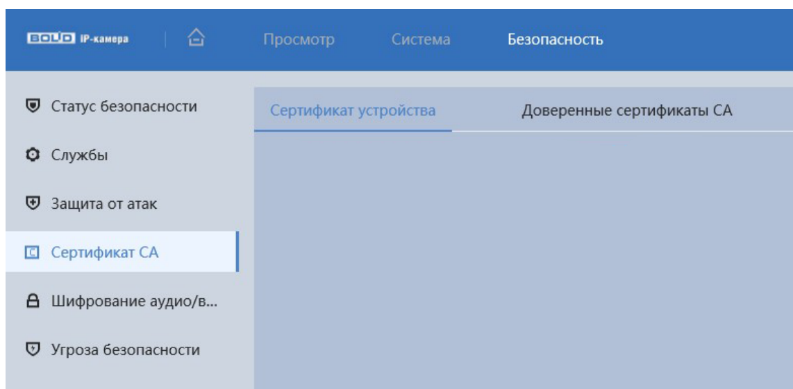
Рисунок 7.150 – Подраздел меню «Сертификат СА»
