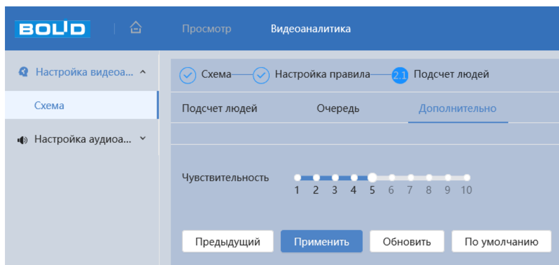
Рисунок 7.39 – Вкладка «Подсчёт людей: Дополнительно»
