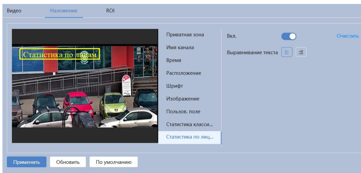
Рисунок 7.79 – Вкладка «Наложение: Статистика по лицам»
