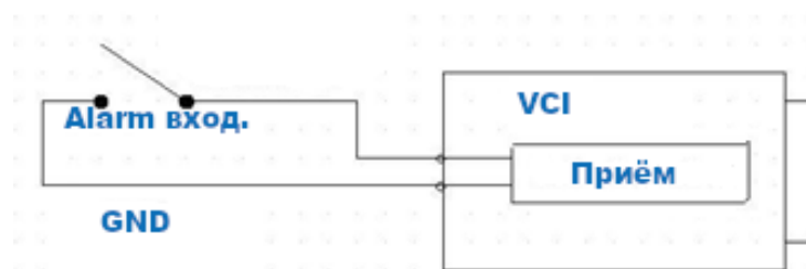
Рисунок 6.12 – Схема подключения тревожного входа
