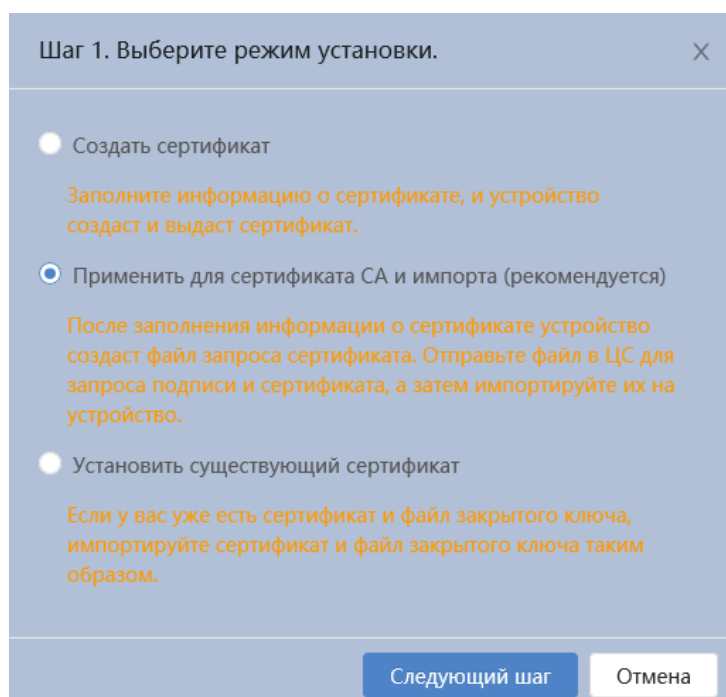
Рисунок 7.152 – Вкладка «Сертификат устройства»: Установка сертификата устройства, шаг 1
