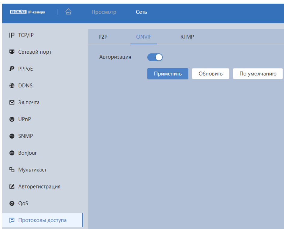
Рисунок 8.20 – Вкладка «ONVIF»
