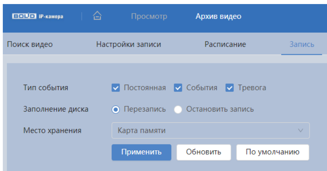
Рисунок 7.126 – Вкладка «Запись»
