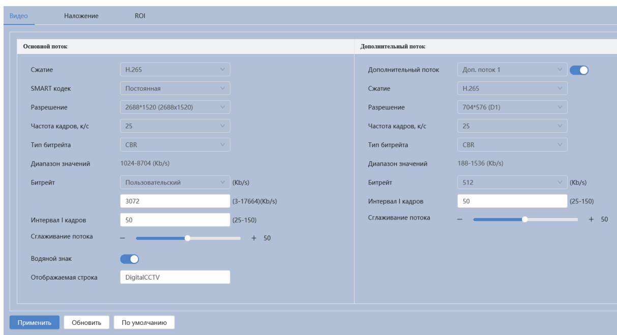
Рисунок 7.70 – Вкладка «Видео»
