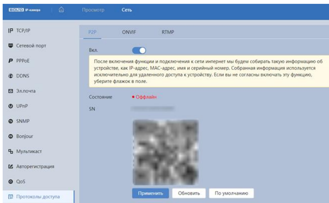
Рисунок 8.19 – Вкладка «P2P»
