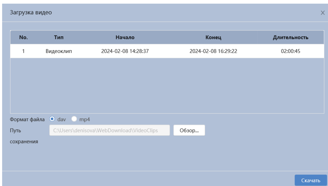
Рисунок 7.122 – Загрузка видео
