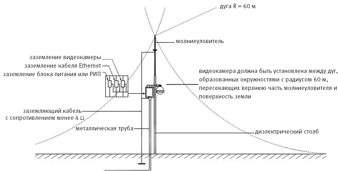
Рисунок 6.13 – Установка молниеотвода
