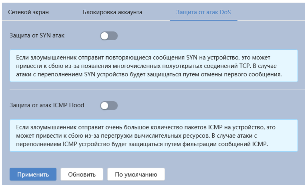
Рисунок 7.149 – Вкладка «Защита от атак DoS»
