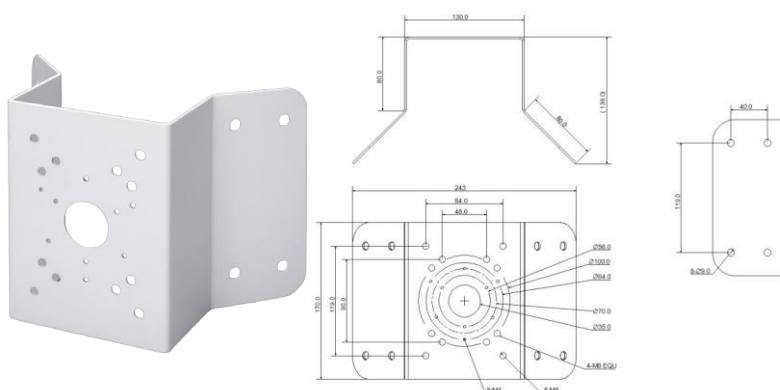
Рисунок 5.10 – Угловой кронштейн BR-102
