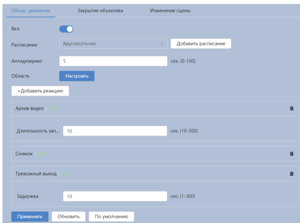
Рисунок 7.90 – Вкладка «Обнаружение движения»
