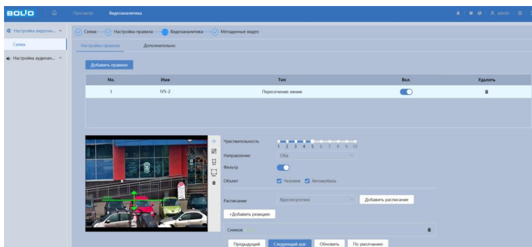
Рисунок 7.28 – Создание правила видеоаналитики «Пересечение линии»
