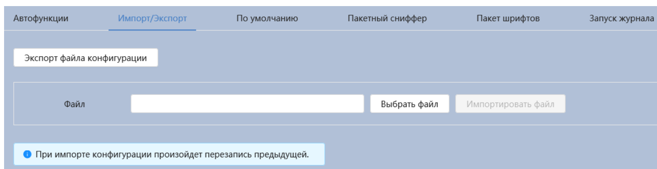
Рисунок 7.113 – Вкладка «Импорт/Экспорт»
