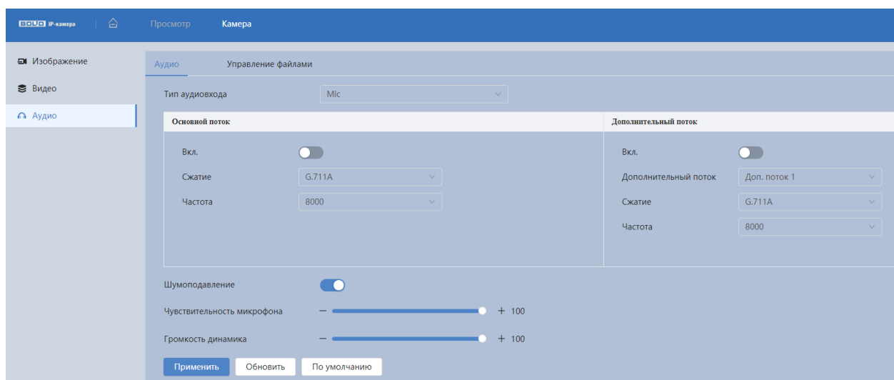
Рисунок 7.82 – Вкладка «Аудио»
