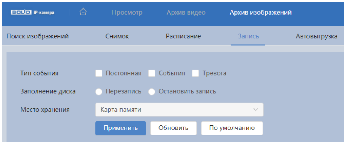
Рисунок 7.132 – Вкладка «Запись»
