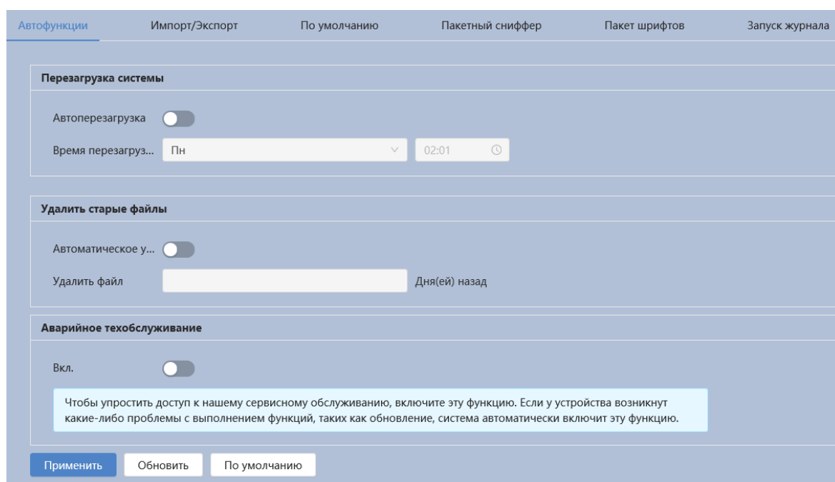
Рисунок 7.112 – Вкладка «Автофункции»
