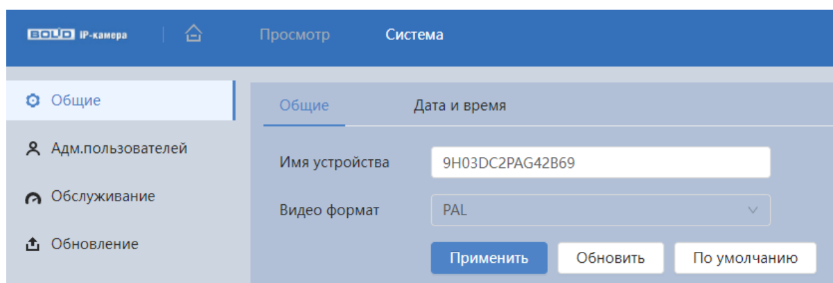
Рисунок 7.102 – Вкладка «Общие»
