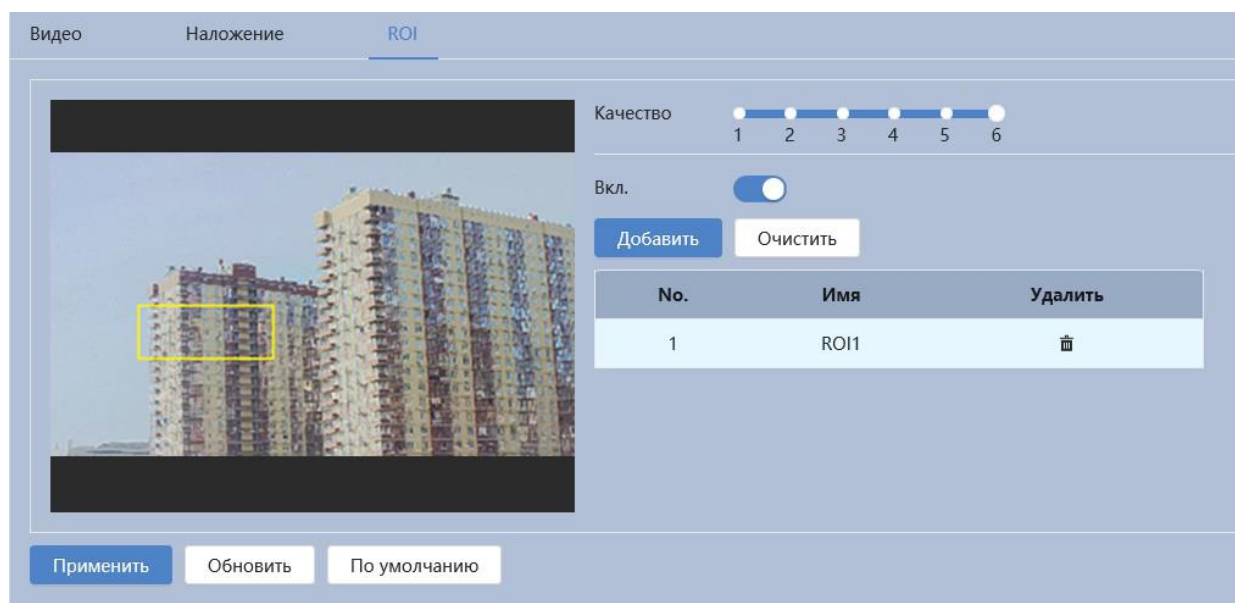
Рисунок 7.80 – Вкладка «ROI»
