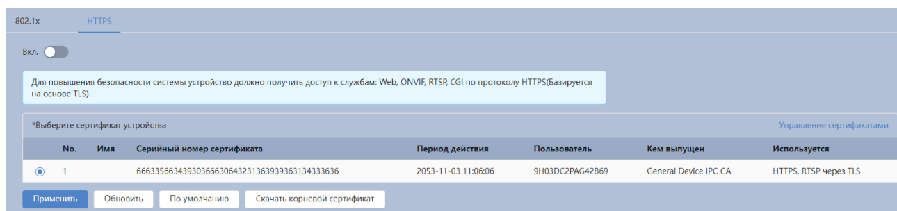
Рисунок 7.145 – Вкладка «HTTPS»
