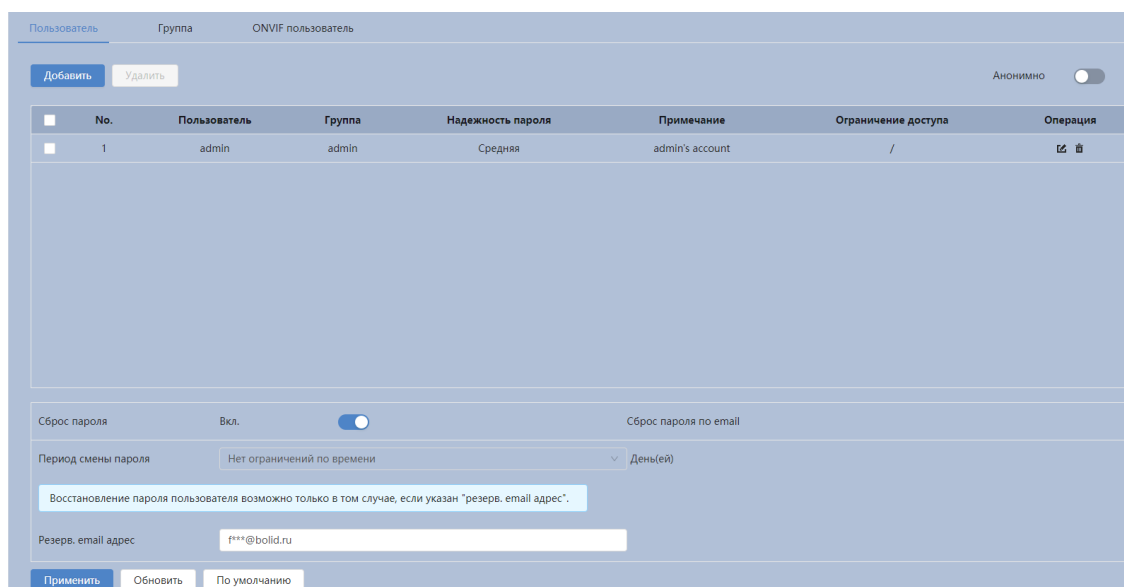
Рисунок 7.105 – Вкладка «Пользователь»
