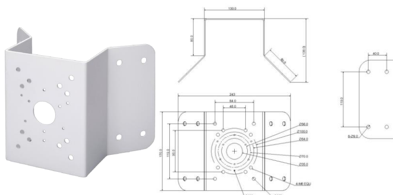
Рисунок 5.14 – Угловой кронштейн BR-102
