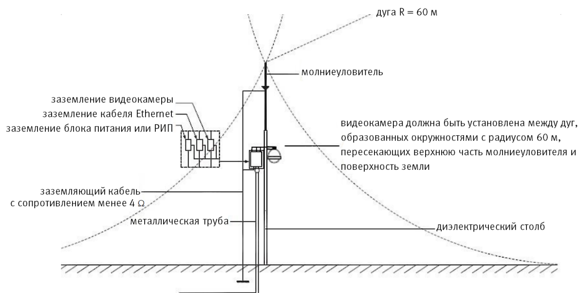
Рисунок 6.13 – Установка молниеотвода
