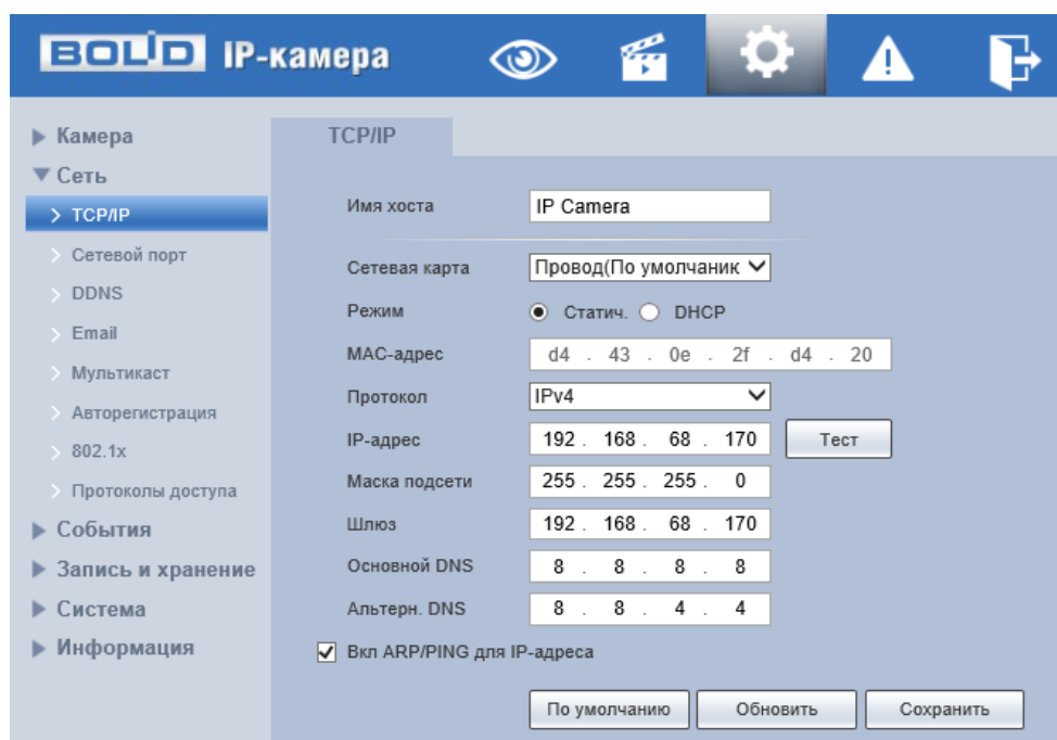
Рисунок 7.54 – Подпункт меню «TCP/IP»
