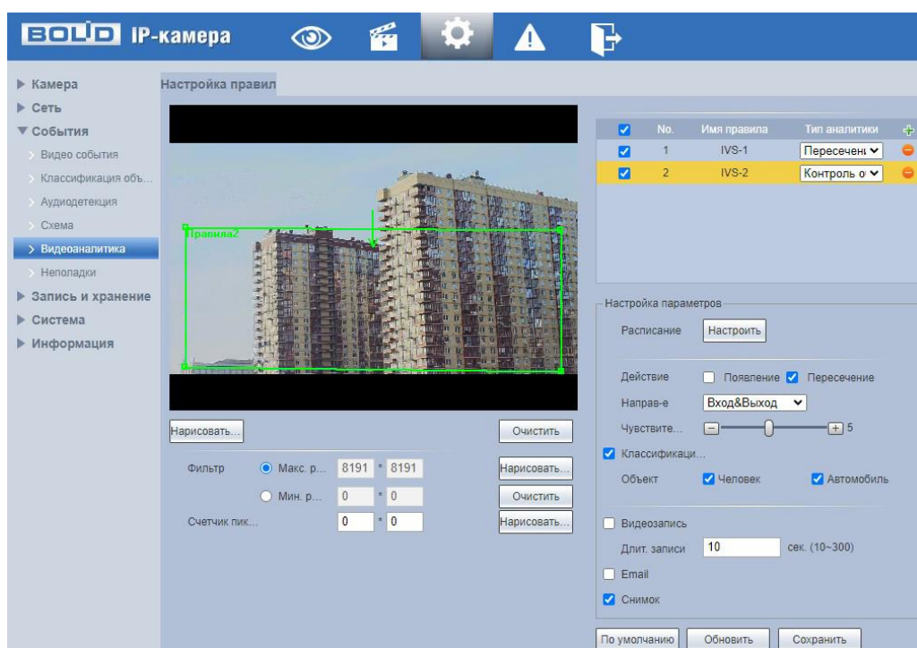
Рисунок 7.81 – Создание правила видеоаналитики «Контроль области»
