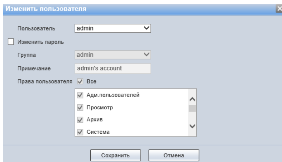
Рисунок 7.109 – Вкладка «Пользователь»: Изменить пользователя
