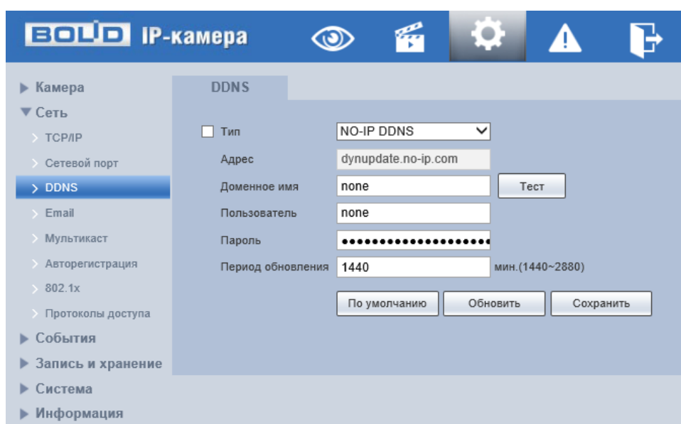
Рисунок 7.56 – Подпункт меню «DDNS»
