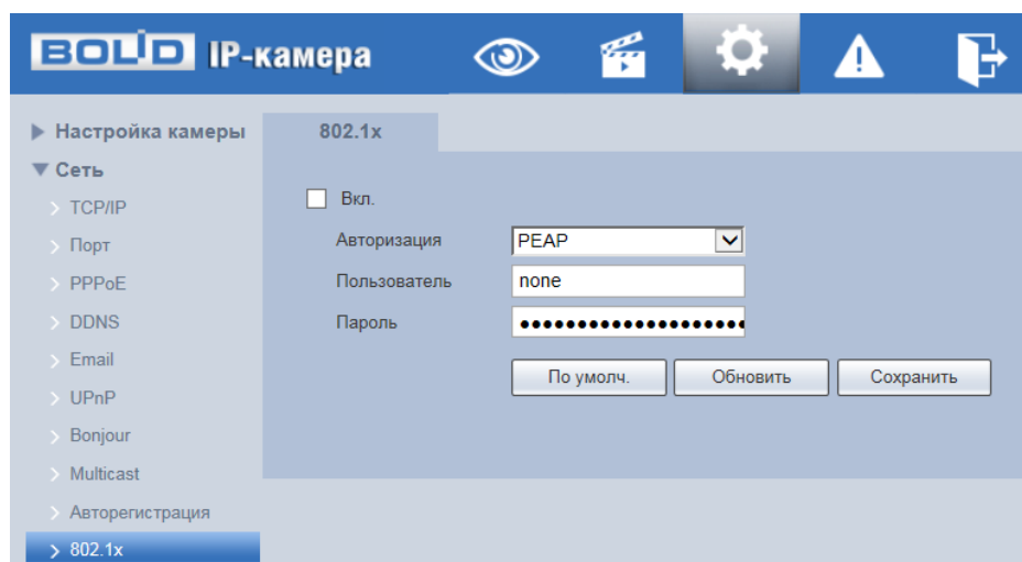
Рисунок 7.62 – Подпункт меню «802.1х»
