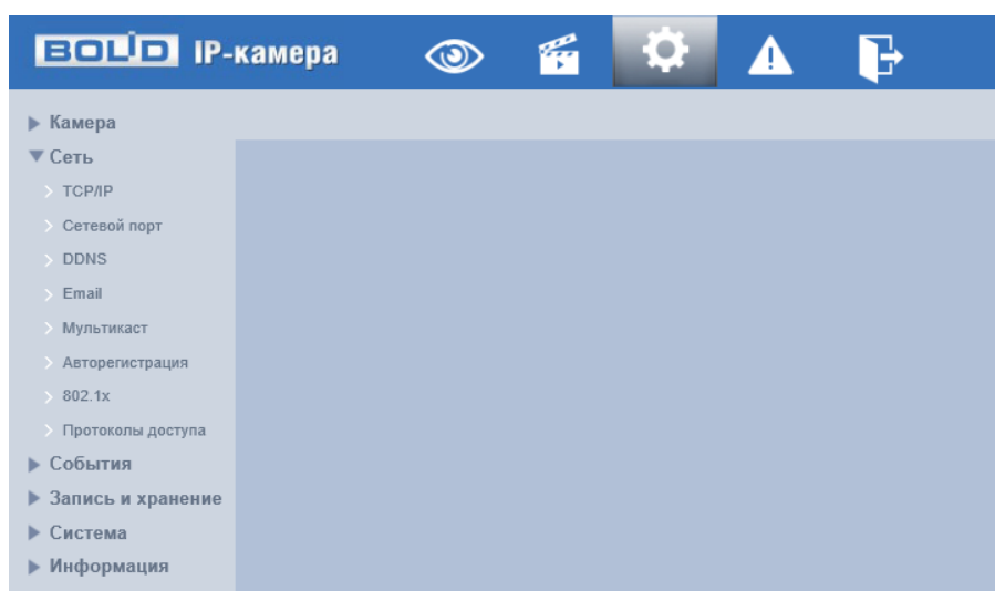
Рисунок 7.52 – Пункт меню «Сеть»
