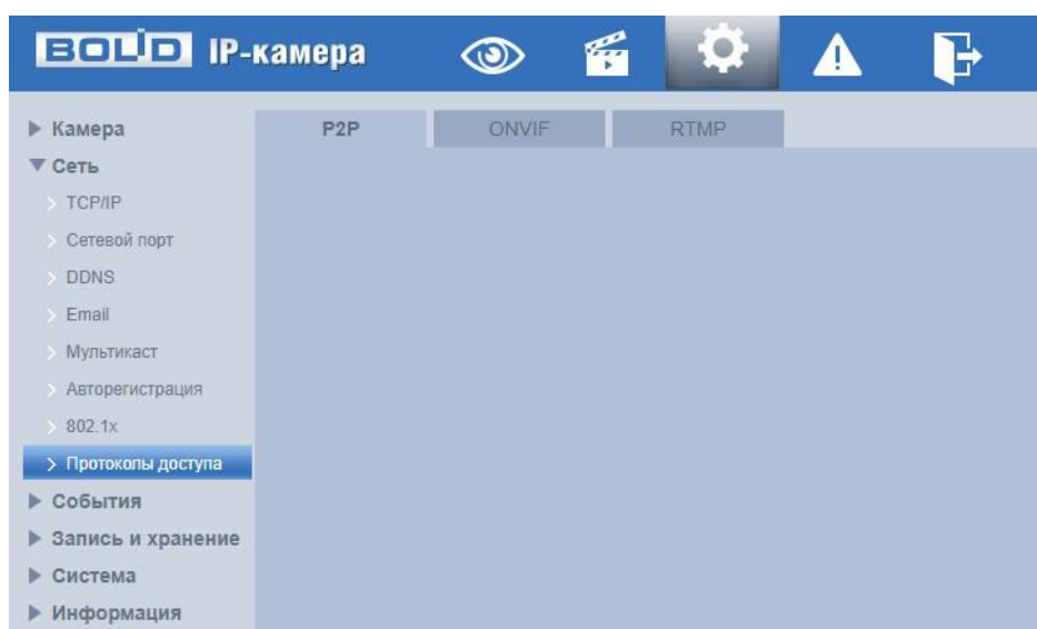
Рисунок 7.63 – Подпункт меню «Протоколы доступа»
