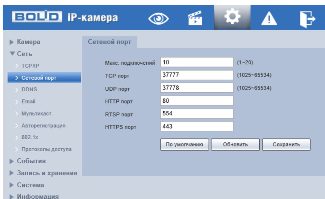
Рисунок 7.55 – Подпункт меню «Сетевой порт»
