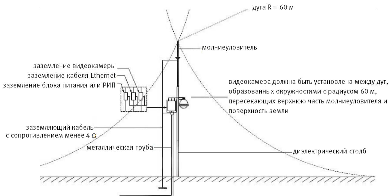
Рисунок 6.13 – Установка молниеотвода
