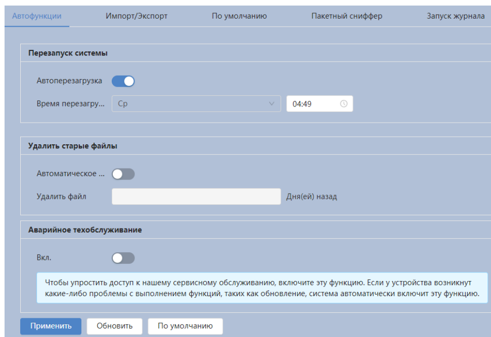
Рисунок 7.82 – Вкладка «Автофункции»
