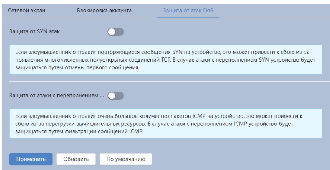
Рисунок 7.112 – Вкладка «Защита от атак DoS»
