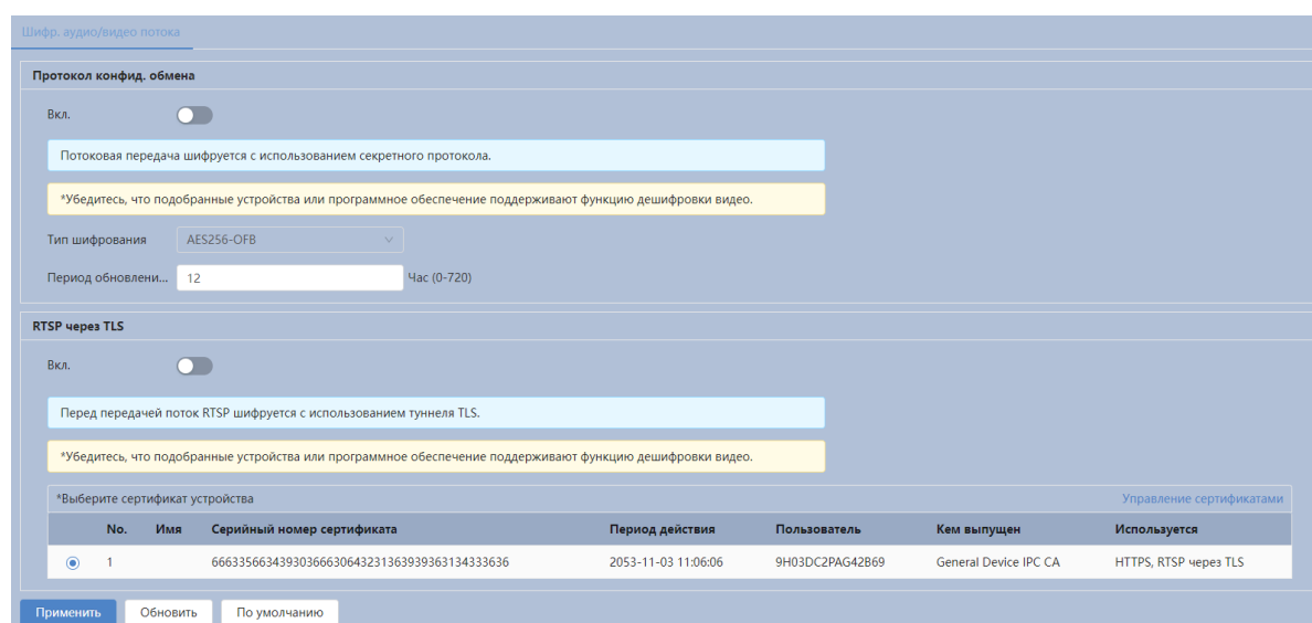
Рисунок 7.119 – Подраздел меню «Шифрование аудио/видео»
