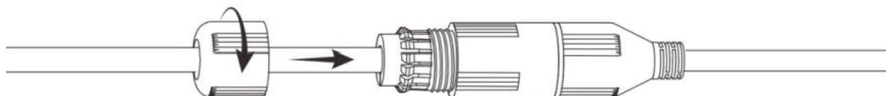
Рисунок 6.11 – Совмещение колпачка с основанием герметичной кабельной муфты
