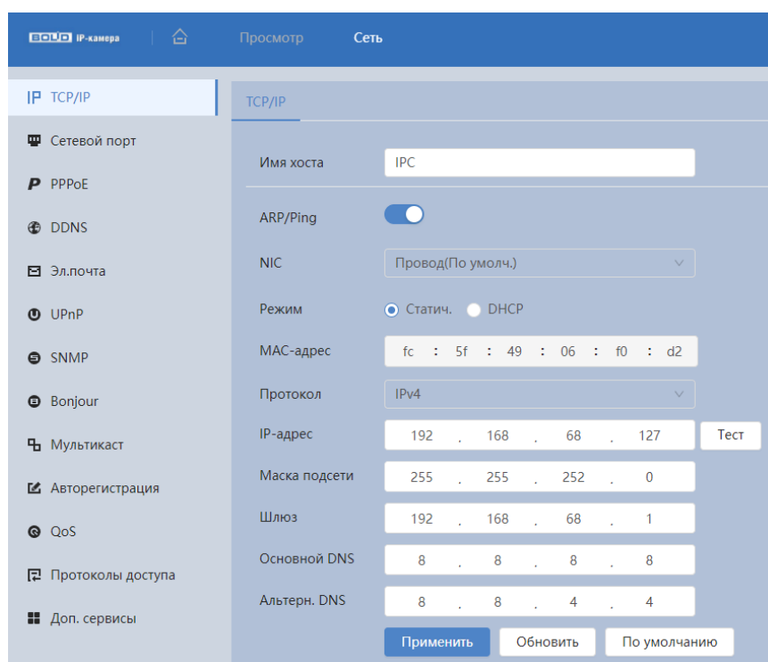
Рисунок 8.5 – Подпункт меню «TCP/IP»
