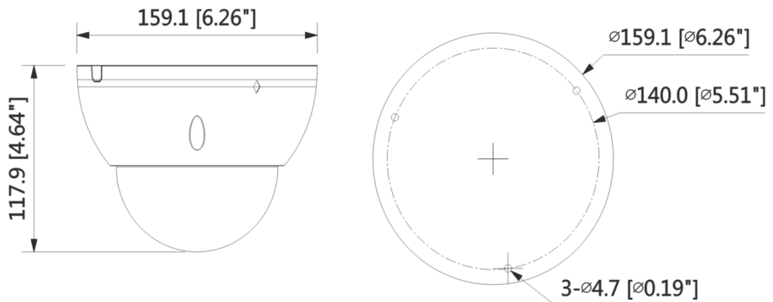
Рисунок 5.1 – Габаритные размеры видеокamеры
