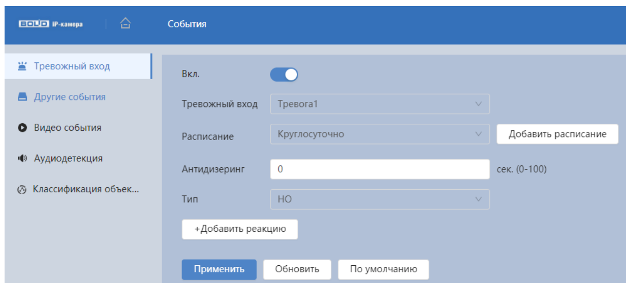
Рисунок 9.92 – Подраздел меню «Тревожный вход»
