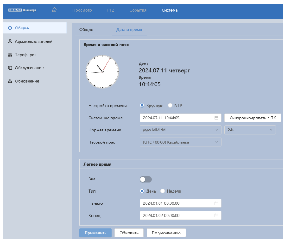
Рисунок 9.111 – Вкладка «Дата и время»
