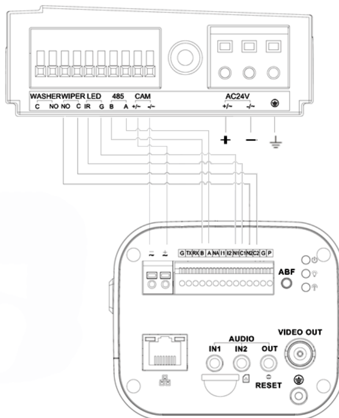
Рисунок 9.127 – Схема подключения
