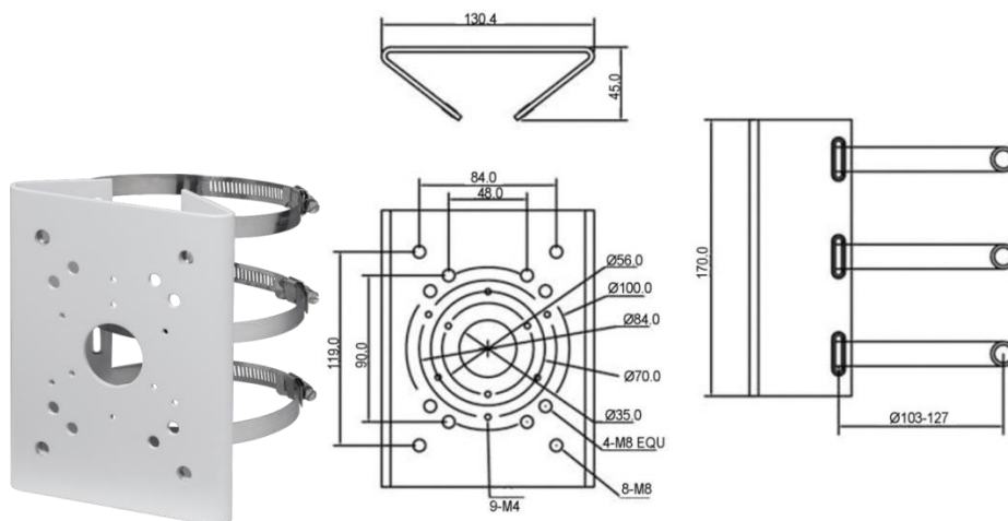
Рисунок 7.7 – Столбовой кронштейн BR-103
