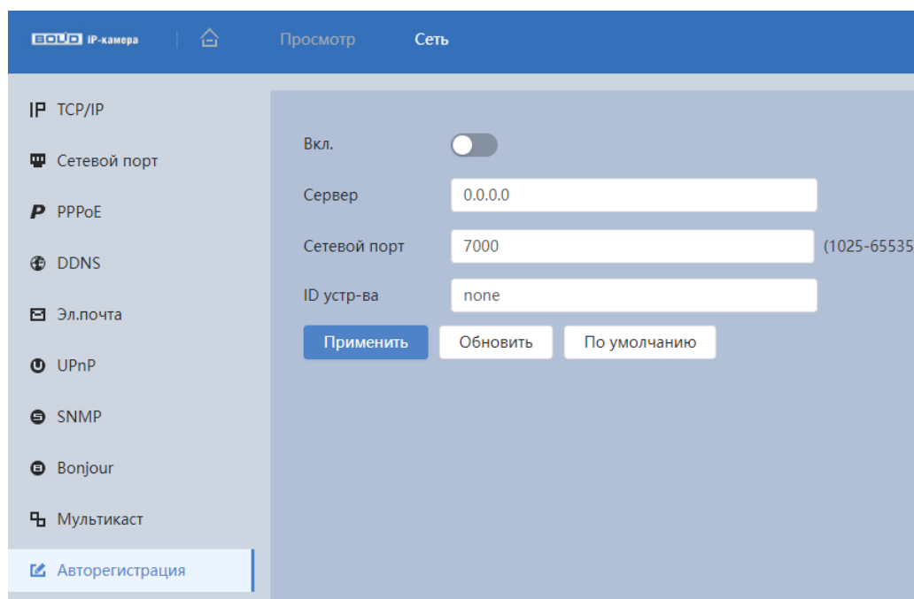
Рисунок 10.15 – Подпункт меню «Авторегистрация»
