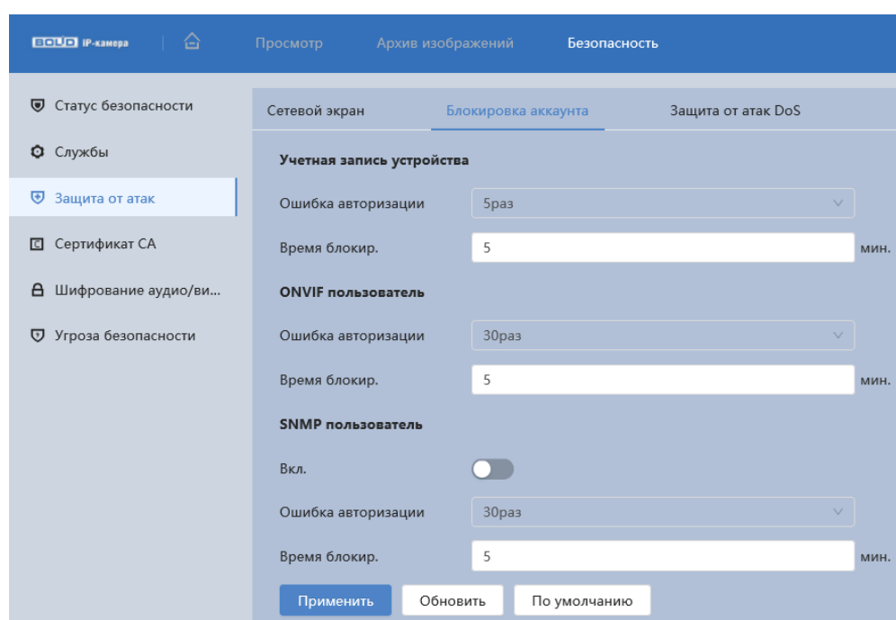
Рисунок 7.135 – Вкладка «Блокировка аккаунта»
