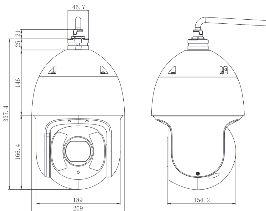
Рисунок 5.1 – Габаритные размеры видеочамеры (мм)
