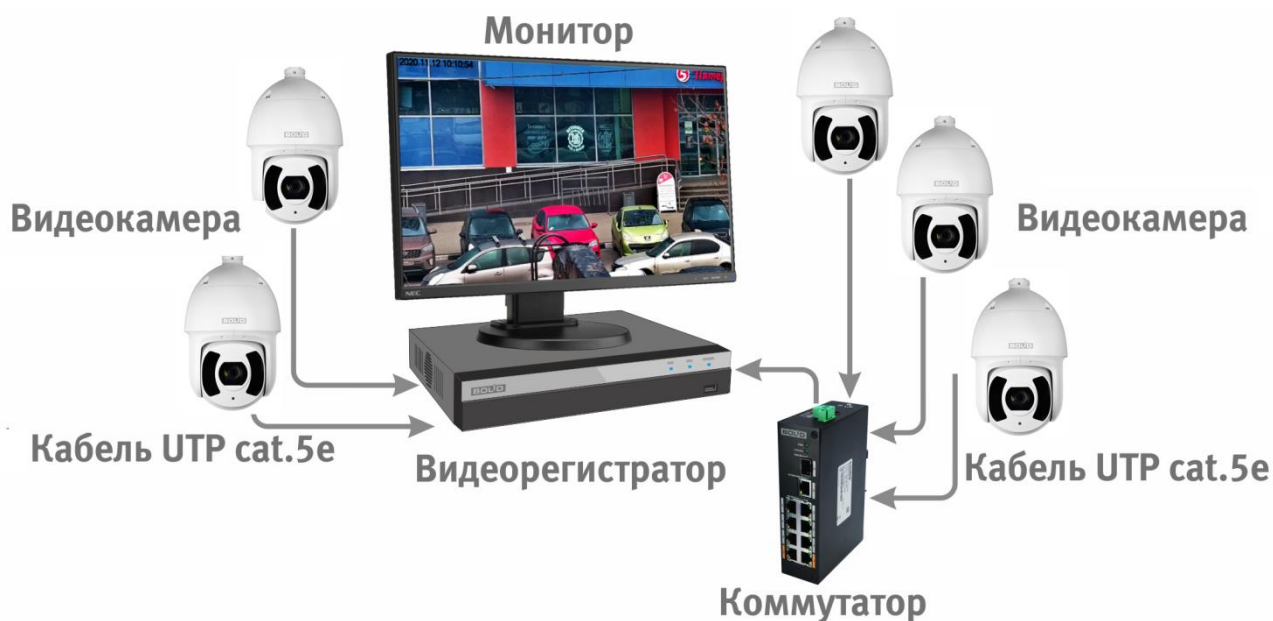
Рисунок 6.4 – Схема подключения видеокамеры к видеорегистратору
