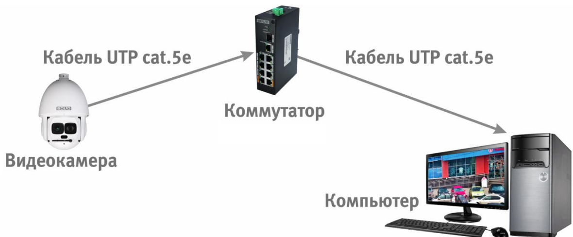
Рисунок 6.3 – Схема подключения видеокамеры к компьютеру через коммутатор
